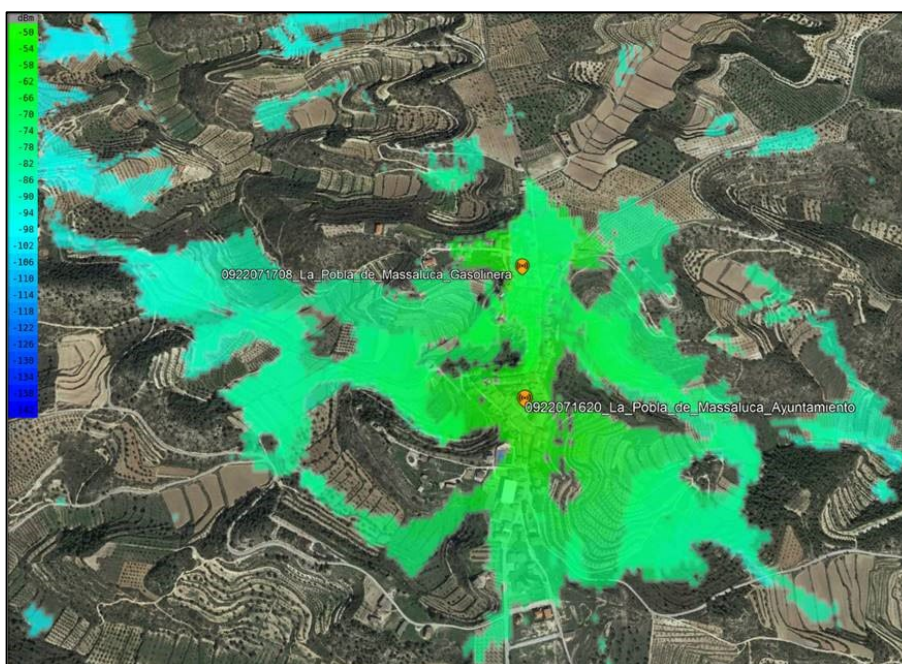
Figura núm.3 Mapa cobertures LoRaWan a La Pobla de Massalua (Font: Vodafone)
