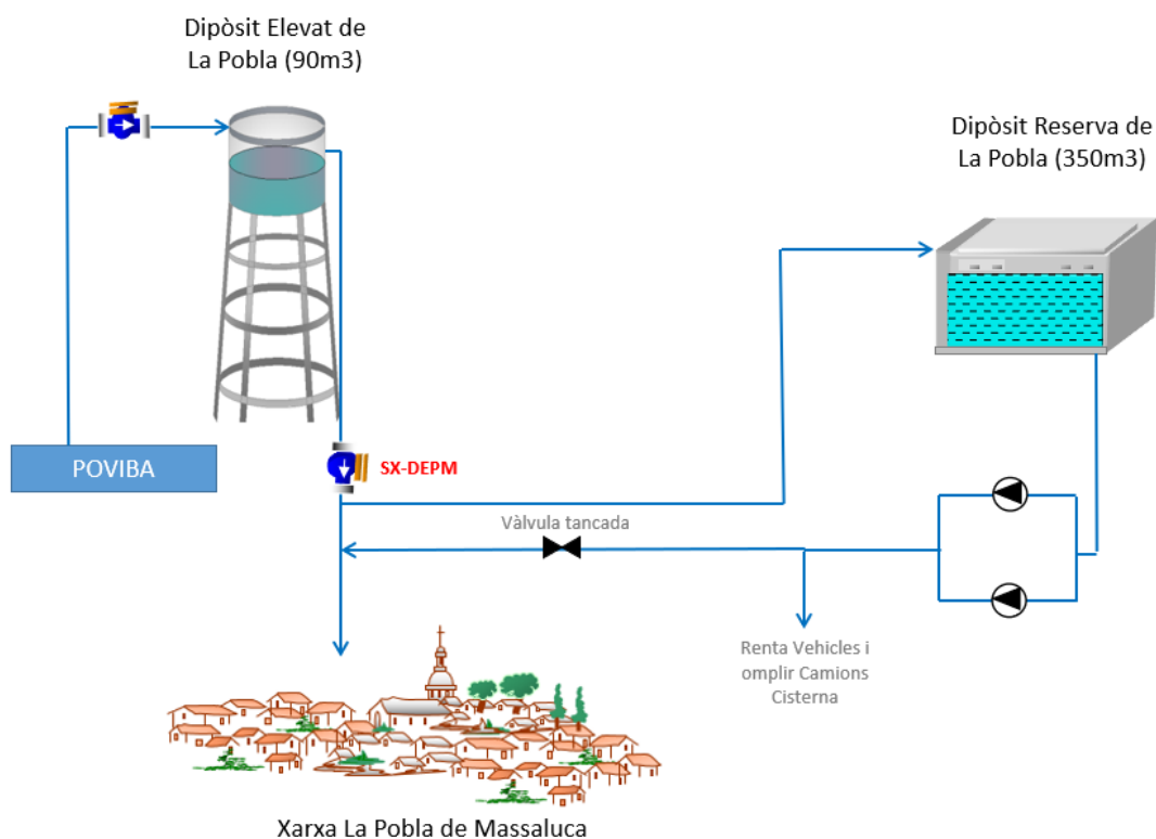
Figura núm.1 Esquema hidràulic de l'abastament a La Pobla de Massalua (Font: Ajuntament)
