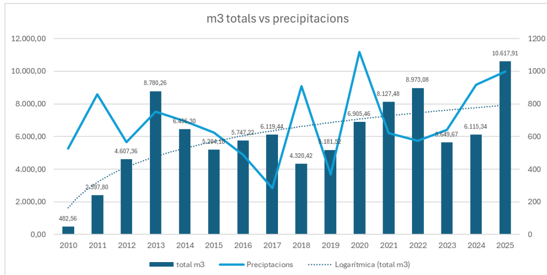
Fig. 1. Comparativa de lixiviat tractat i pluviometria (període 2010-2025).
