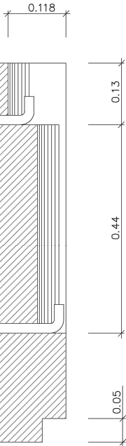
SECCIÓ B-B' ESCALA 1: 5
