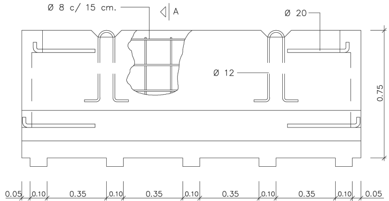
SECCIÓ A-A'
