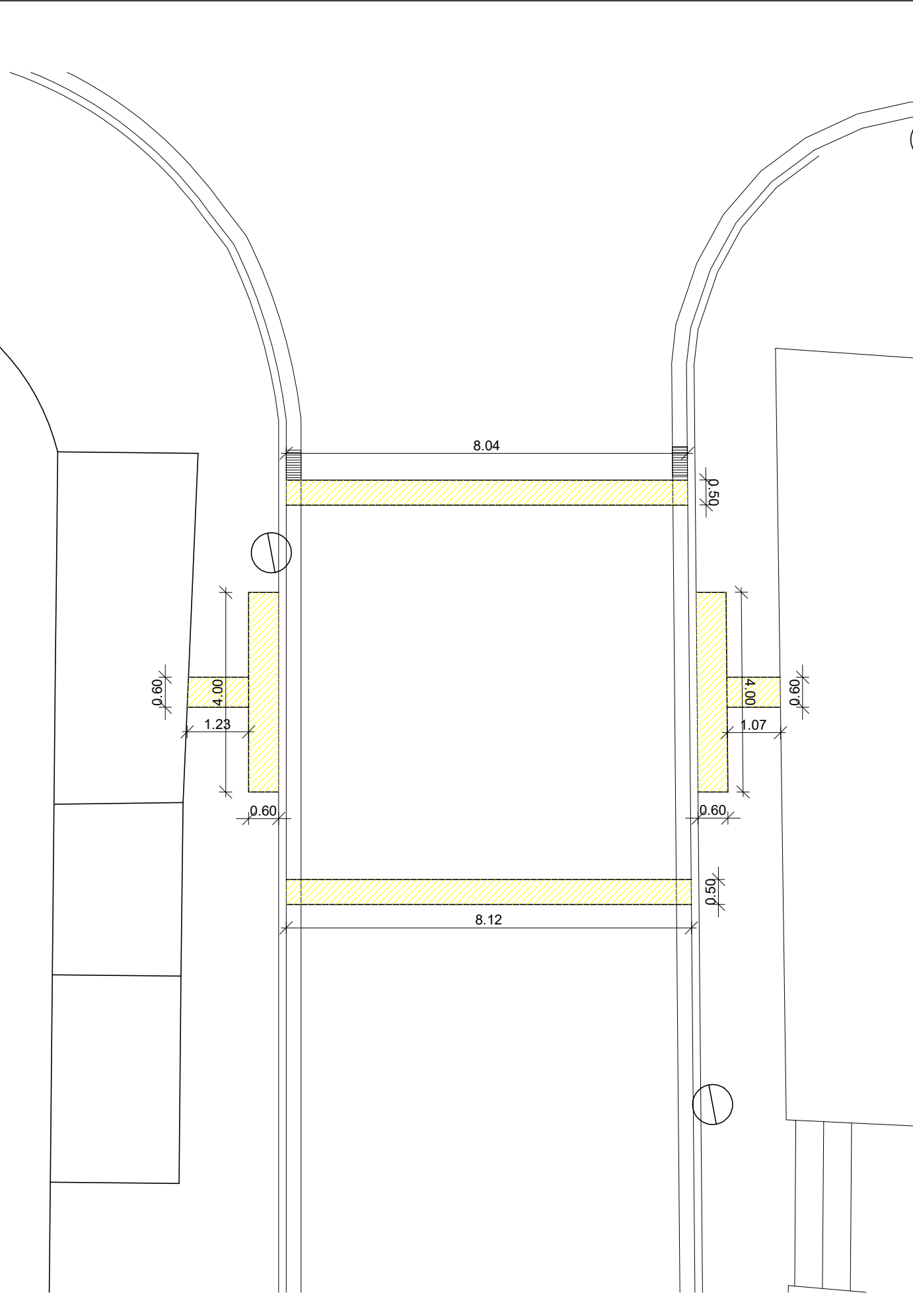
ESTAT EXISTENT
