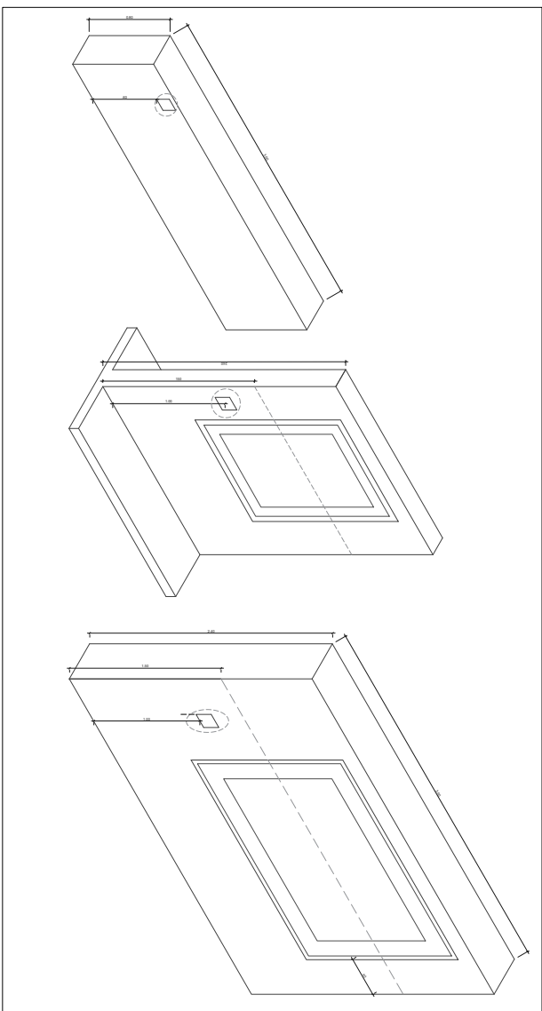
TIPOLOGIA CARTELA SOBRE SOPORTES, E 120
