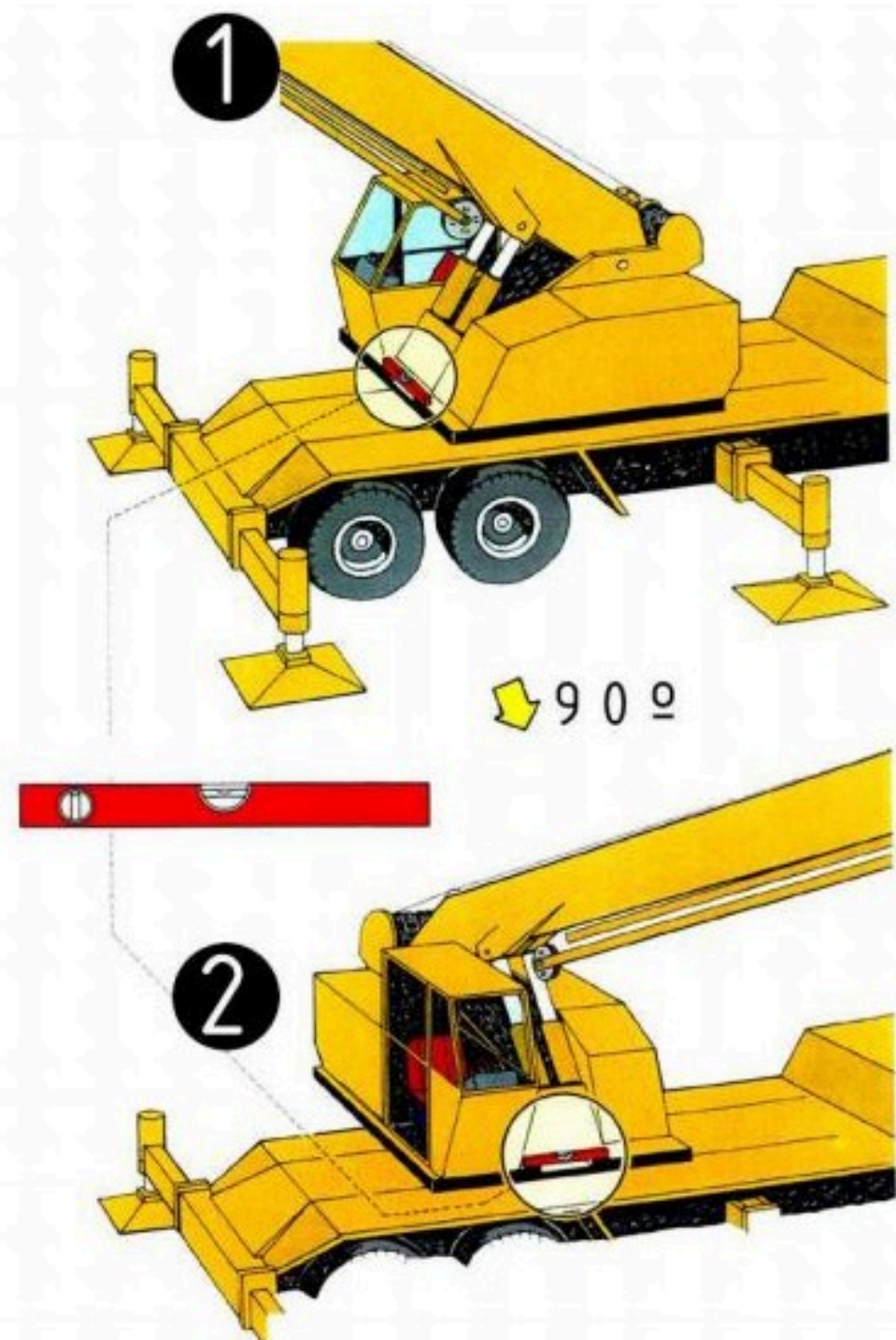
1. CONTROL DE NIVELL POSTERIOR 2. CONTROL DE NIVELL LATERAL
