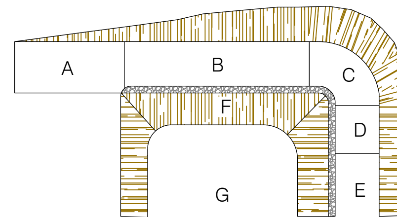
ALÇAT - SECCIÓ
