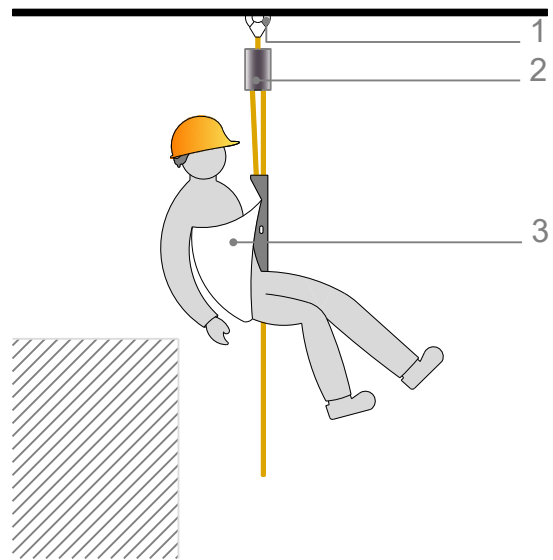
1 PUNT D'ANCORATGE 2 DISPOSITIU DE DESCENS 3 DISPOSITIU DE PRESSIÓ DEL COS (LLAÇ DE SALVAMENT)
