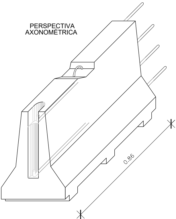
BARRERA RÍGIDA (PORTÀTIL)
