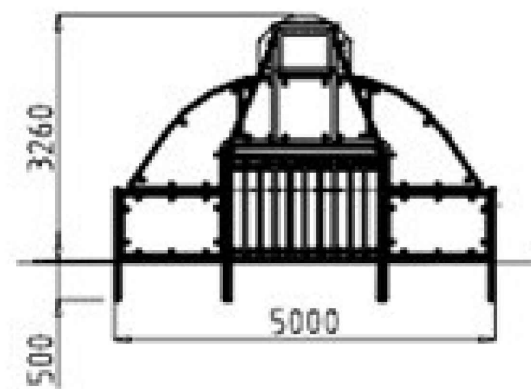
SECCIÓ TRANSVERSAL
