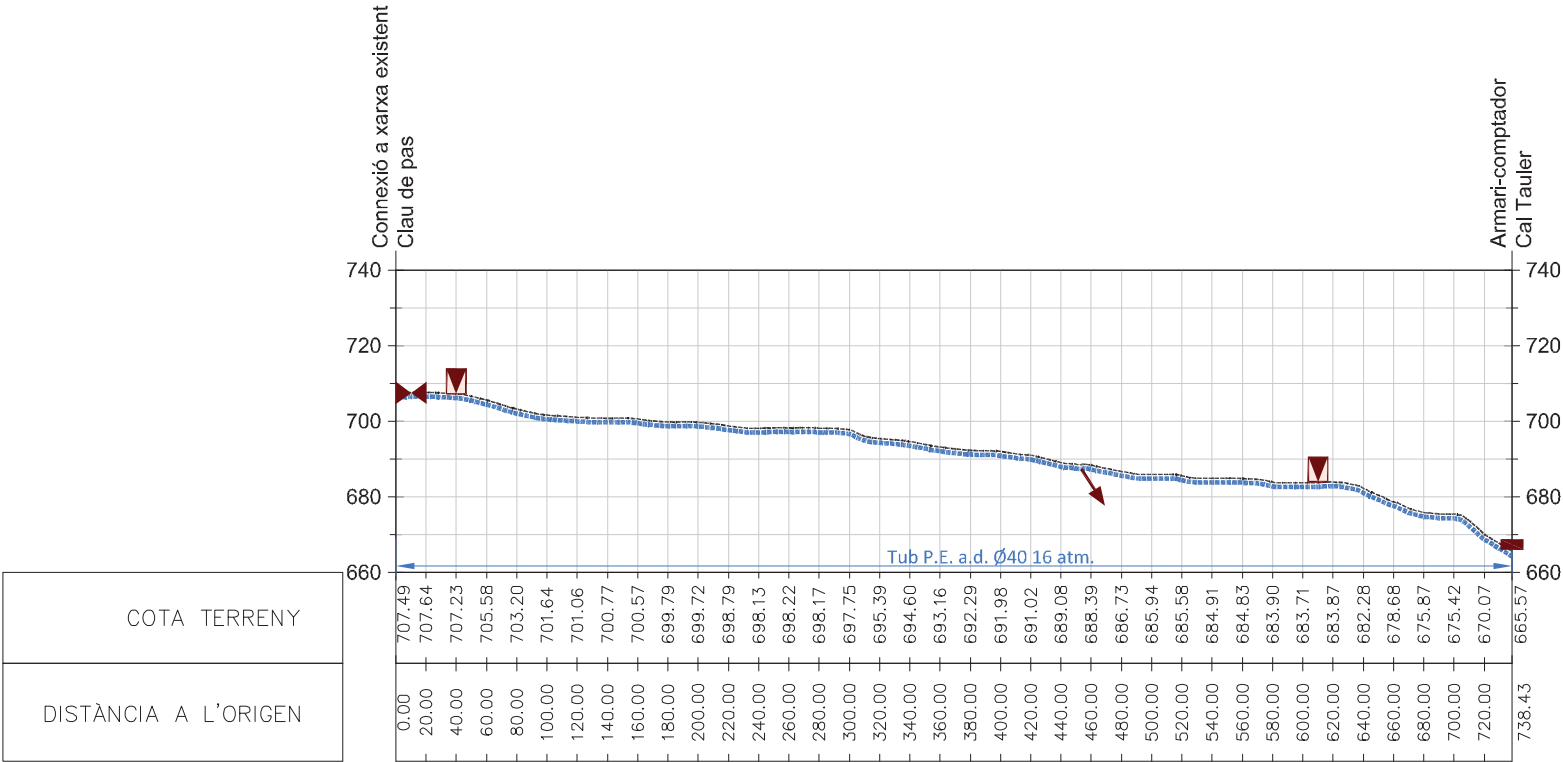
Perfil Longitudinal conducció Cal Tauler
