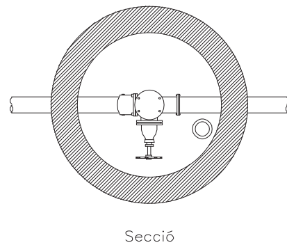
ARQUETA AMB VENTOSA
