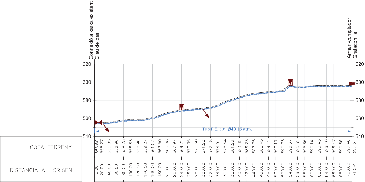
Perfil Longitudinal conducció Grataconills
