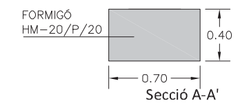
ARMARI PREFABRICAT DE FORMIGÓ
