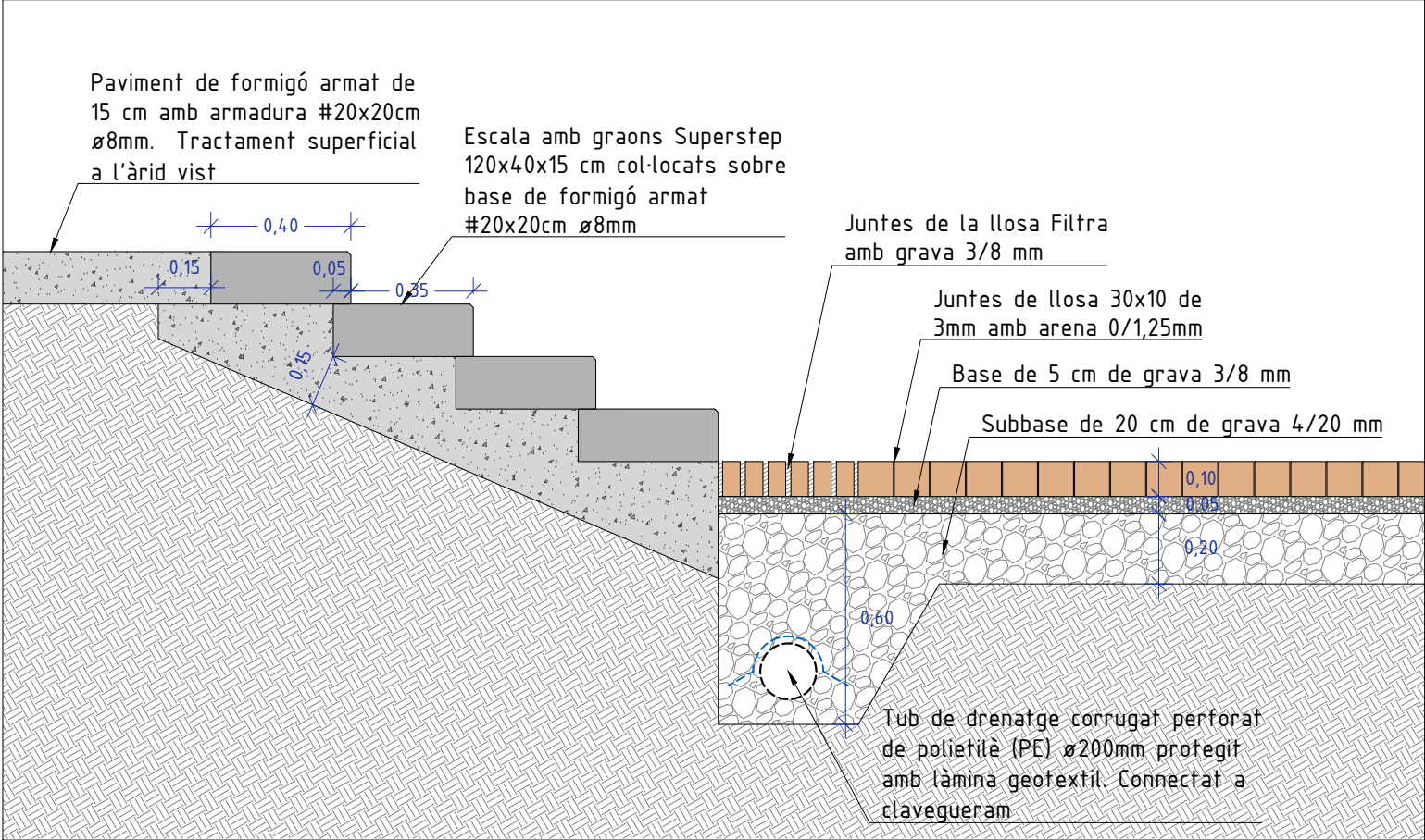
SECCIÓ 1 - 1:20
