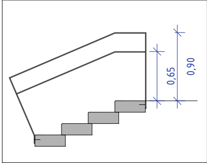
BARANA 4 - 1:50
