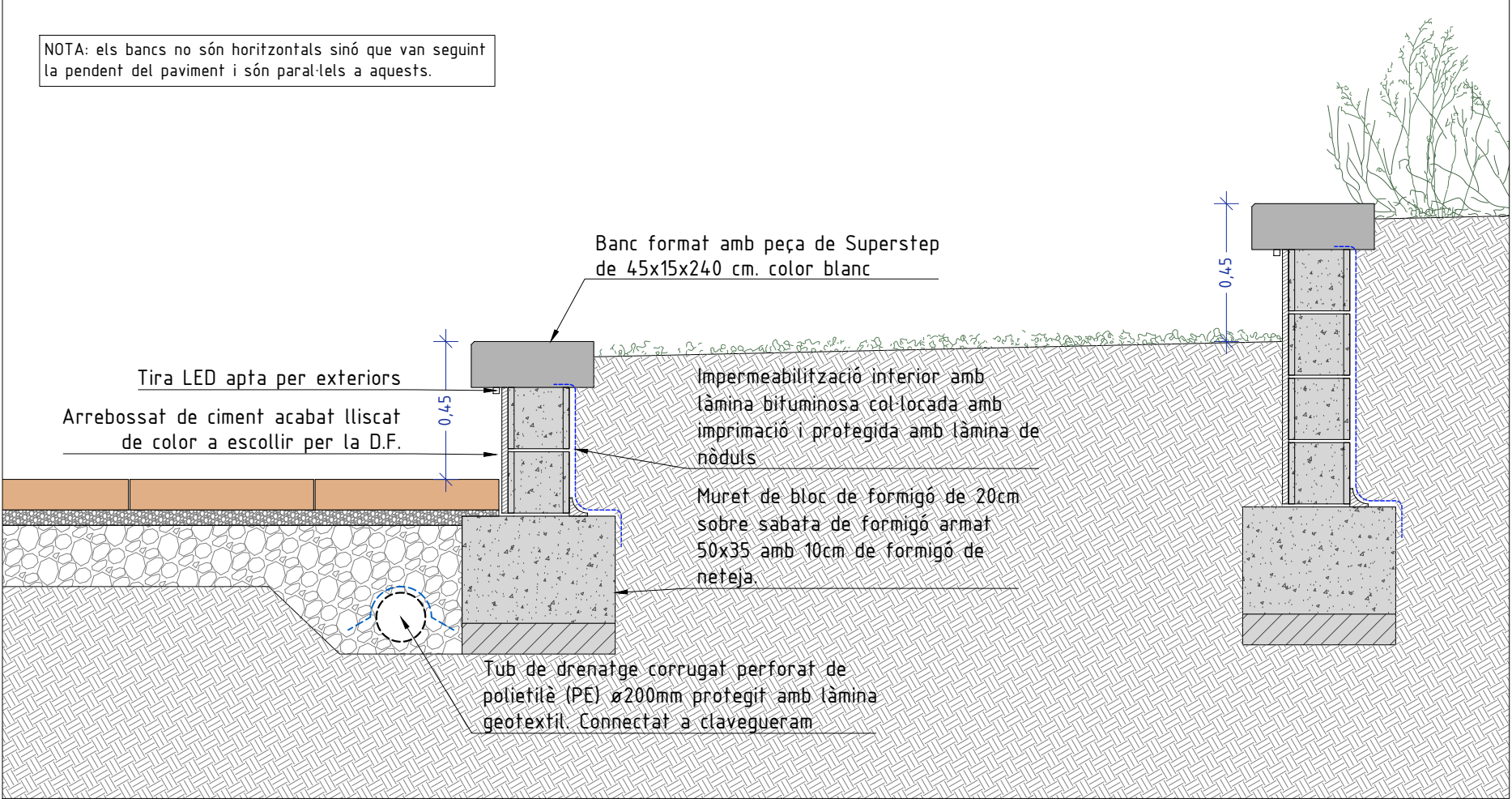
SECCIÓ 2 - 1:20
