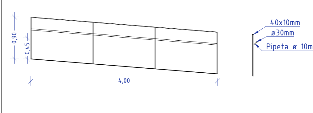
BARANA 5 - 1:50
