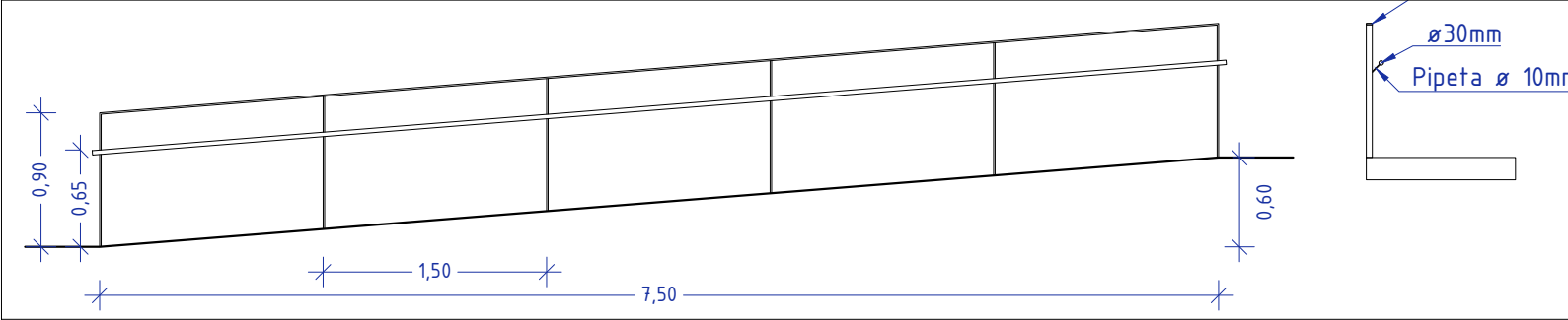
BARANA 1 - 1:50
