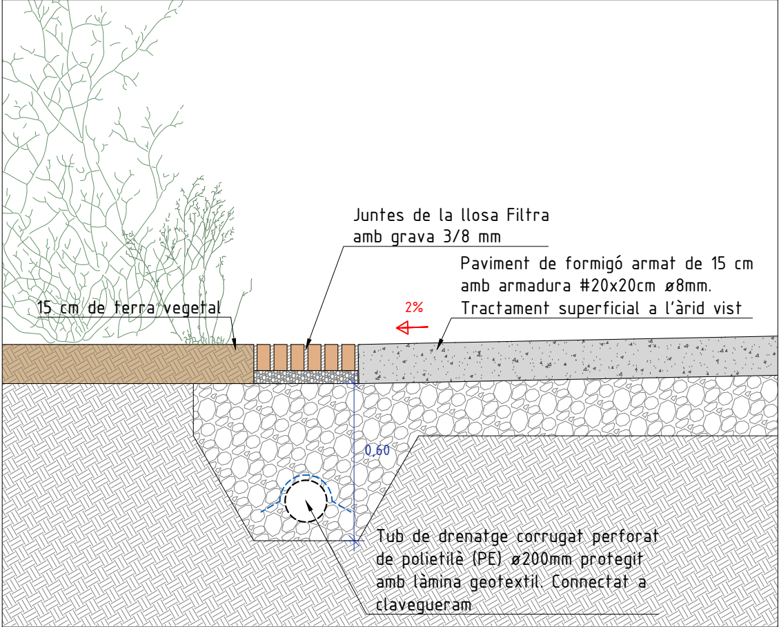
SECCIÓ 3 - 1:20
