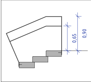
BARANA 3 - 1:50
