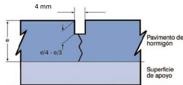
Figura 25. Esquema de junta de contracció executada per serrat.
