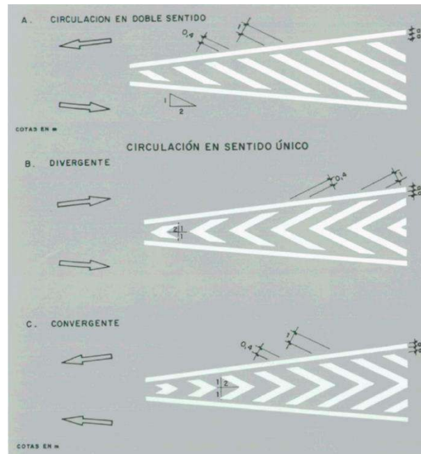
Figura 67. M7.2– Zebrejat zones excloses de trànsit
