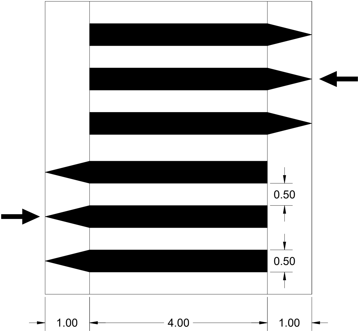
DETALL PAS DE VIANANTS EN RESALT Senyalització horitzontal. Pas de vianants elevat
