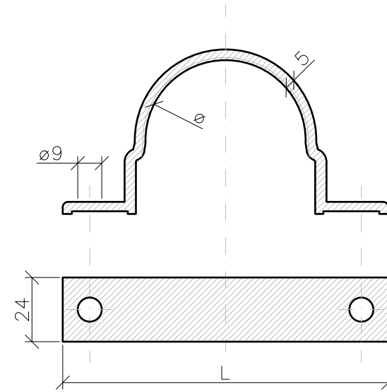
2 DETALL BRIDA
