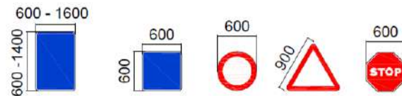
Figura 14. (Cotes en mm) Dimensions senyalització vertical. Instrucció de carreteres 8.1-IC
