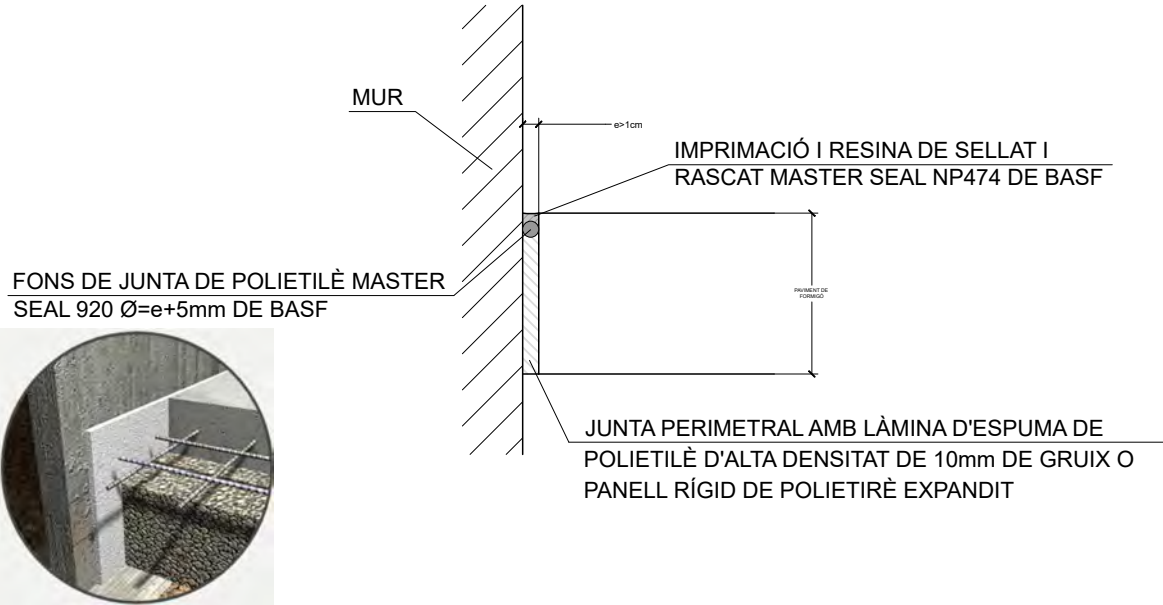
DETALL JUNTA PERIMETRAL AMB ELEMENT RÍGID E: 1/15
