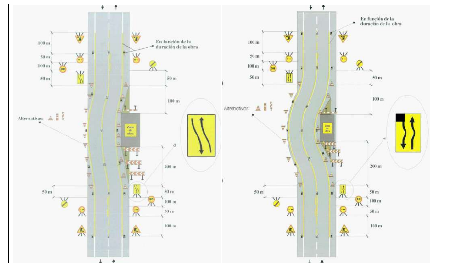
Figura 76. A) Treballs en voravia i part del carril B) Treballs en voravia i part del carril ampliant plataforma
