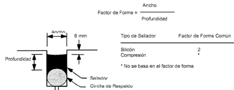
Figura 33. Esquema segellat de junta.
