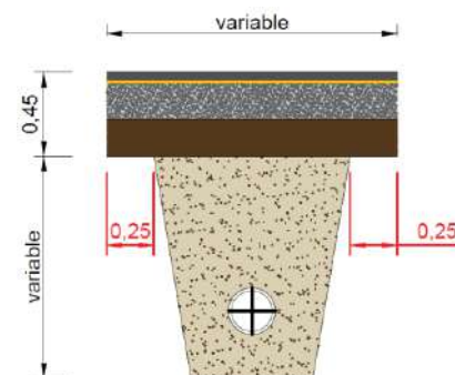
Figura 22. Croquis reposició rasa de servei en zona de calçada.
