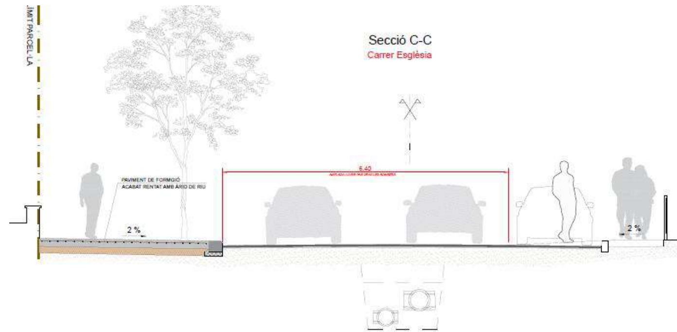
Figura 8. Secció transversal Vial 2.
