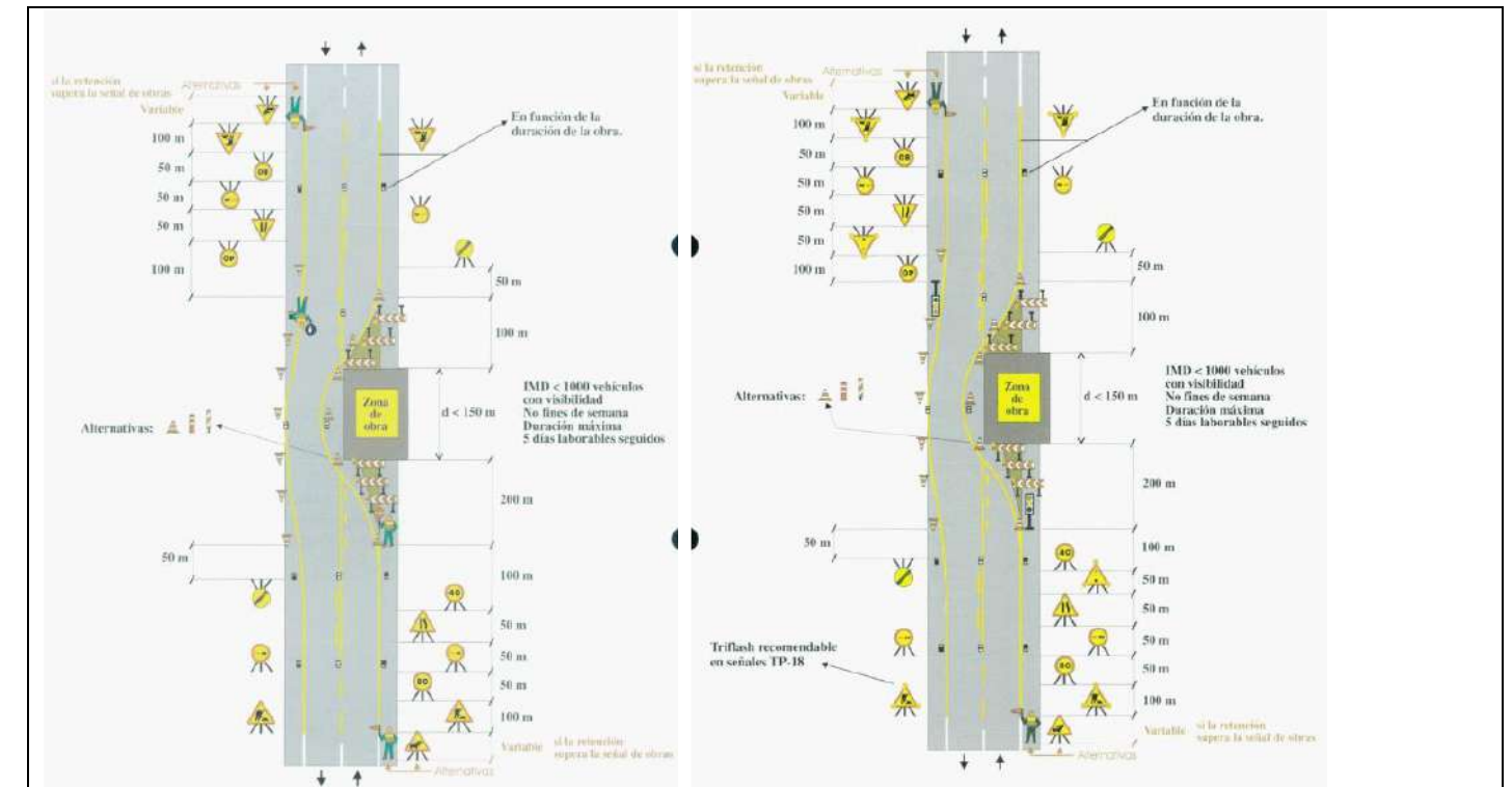
Figura 79. A) Treballs en voravia, un carril i afectació al segon carril (DIA I NIT)
