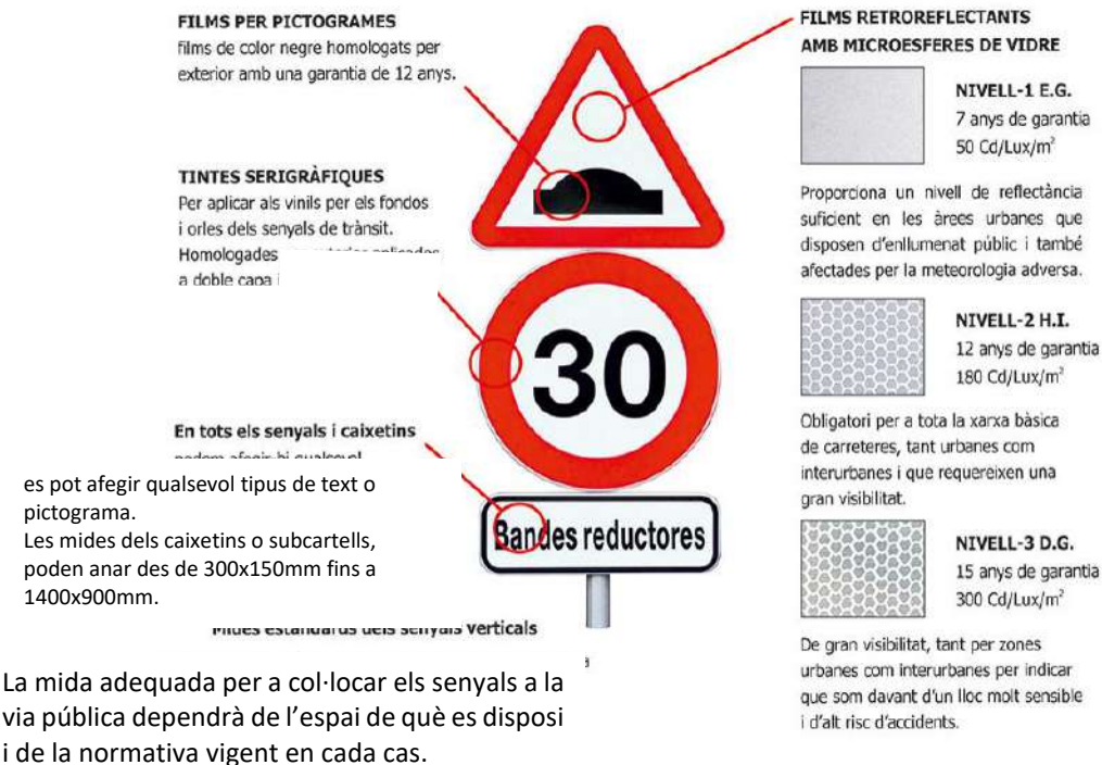
Figura 69. Característiques tipus senyals verticals part frontal.
