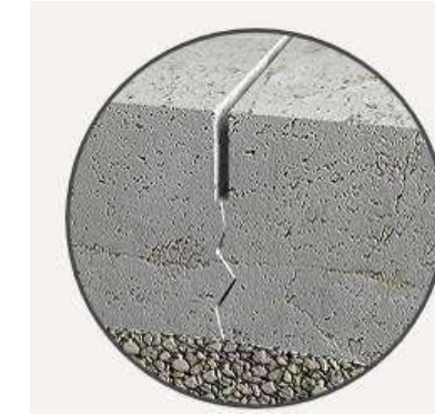
Figura 26. Imatge junta de contracció en paviment de formigó.
