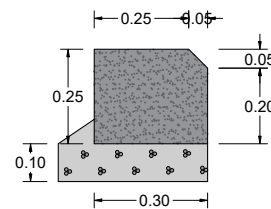
DETALL VORADA GRANÍTICA AMB ACABAT BISELLAT DE 30x40x25 cm E: 1/20
