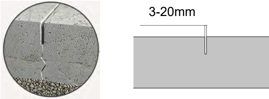
DETALL JUNTA CONTRACCIÓ EN PAVIMENT DE FORMIGÓ E: 1/5
