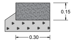
DETALL VORADA ACER GALVANITZAT PER ESCOCELLS E: 1/20
