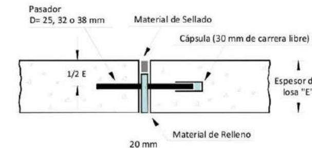
Figura 29. Junta de dilatació amb passadors.
