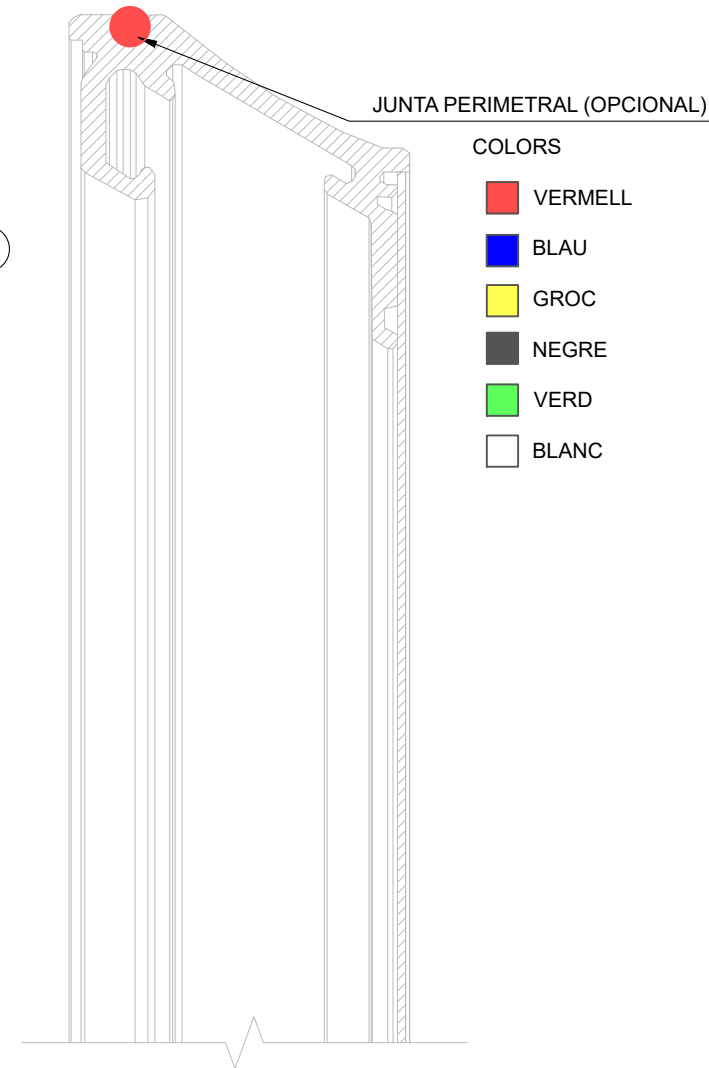
7 SECCIÓ SENYAL
