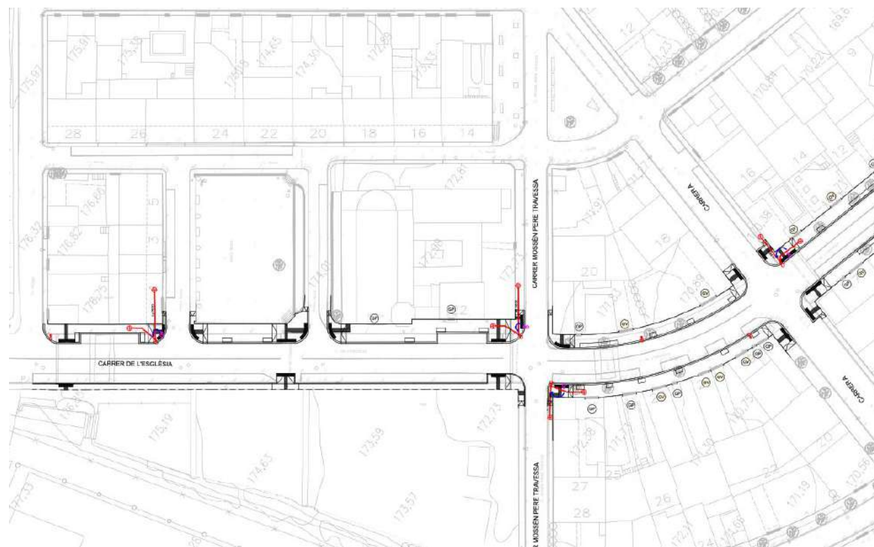
Figura 53. Plànol enllumenat públic punts de llum a reubicar.
