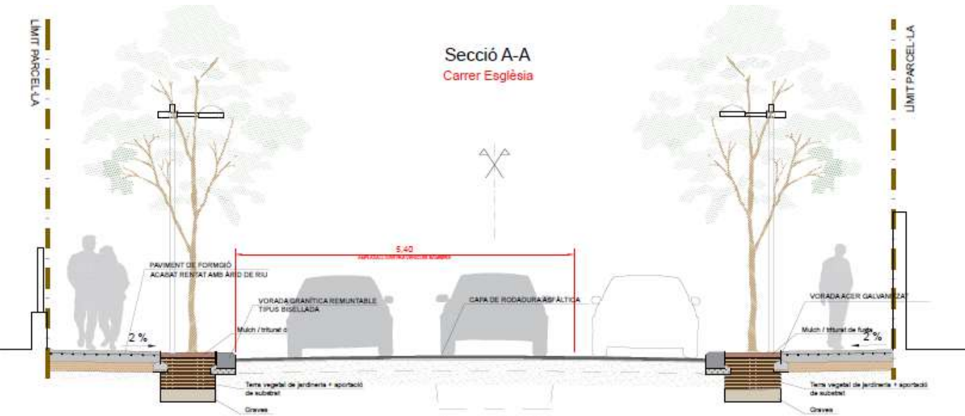
Figura 7. Secció transversal Vial 1.
