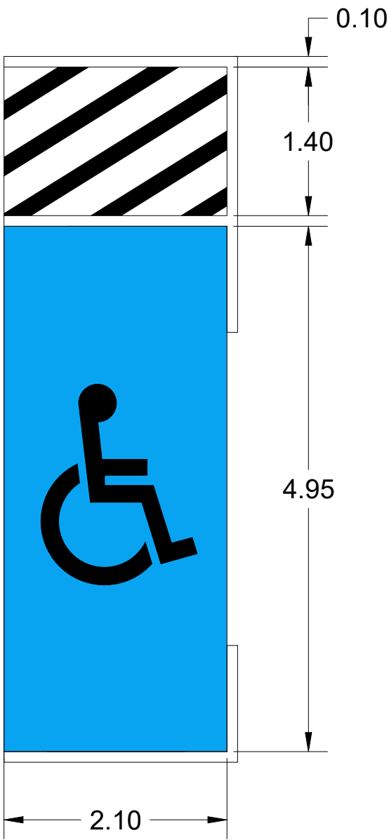
DETALL PLAÇA MR Senyalització horitzontal. Mobilitat reduïda.
