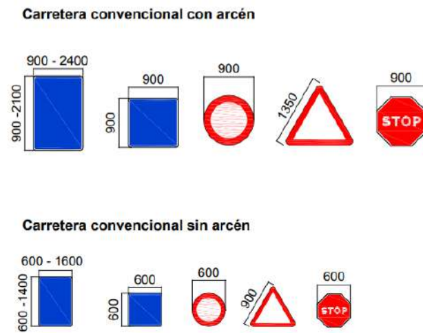
Figura 73. (Cotes en mm) Dimensions senyalització vertical. Instrucció de carreteres 8.1-IC
