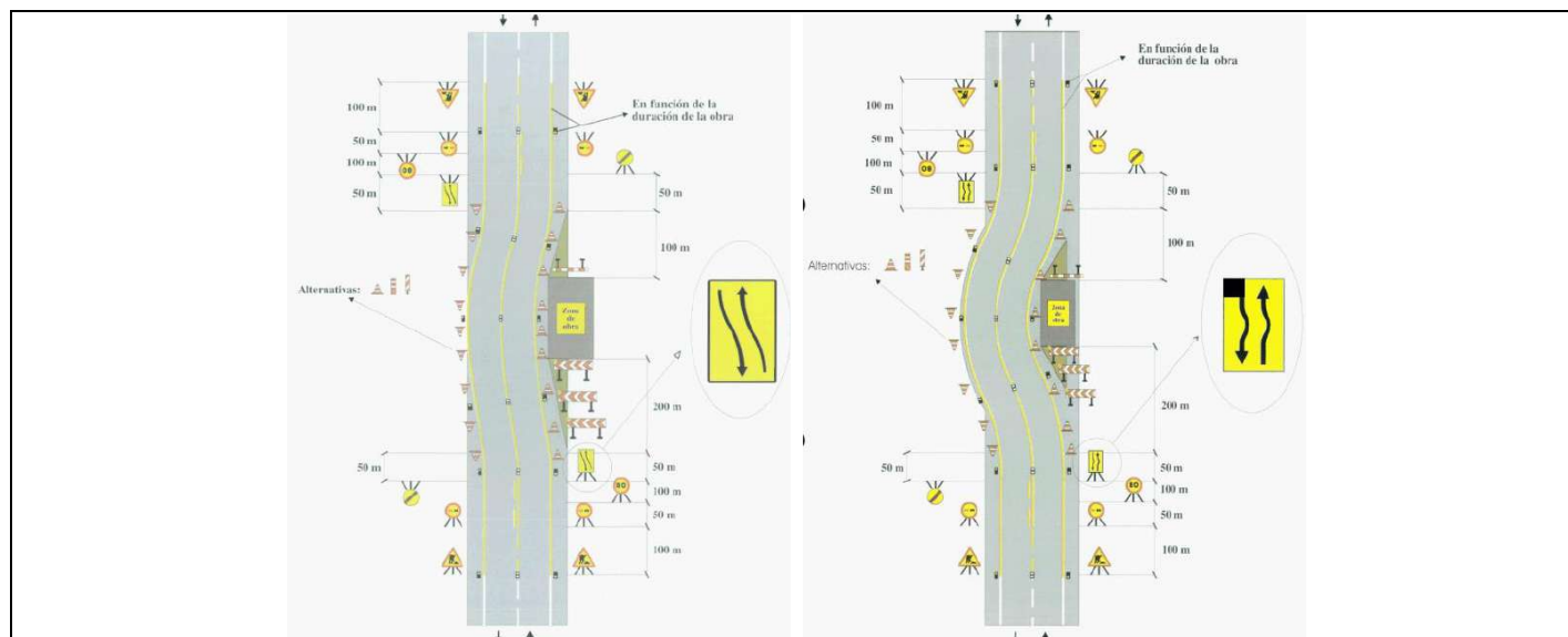
Figura 81. A) Treballs en voravia i part del carril B) Treballs en voravia i part del carril ampliant plataforma
