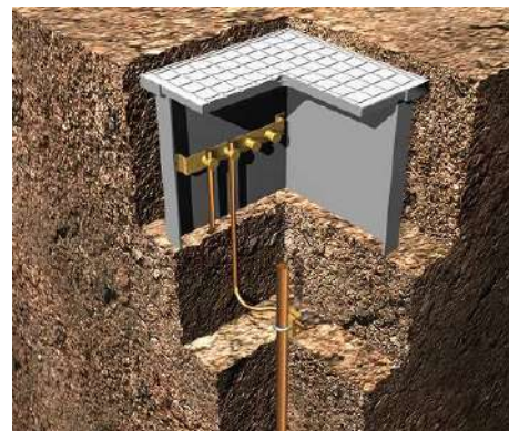
Figura 55. Imatge presa de terra amb pica.
