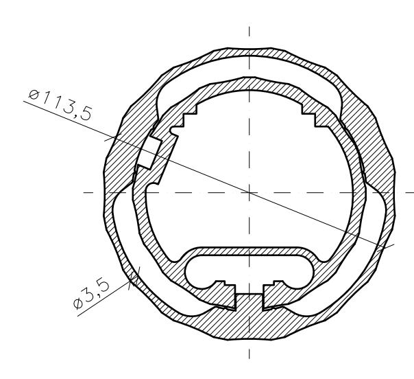
6 SECCIÓ B-B'
