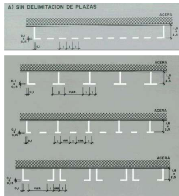
Figura 68. M7.3 i M7.4 – Aparcaments en línia i en bateria.
