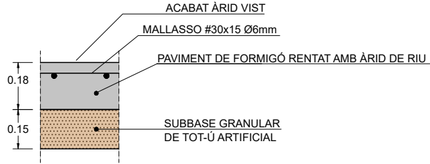
DETALL FERM VORERA DE FORMIGÓ RENTAT ESCALA 1:20
