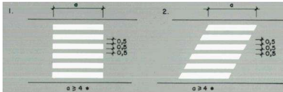
Figura 63. M4.3 – Pas de vianants
