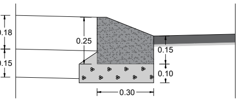
DETALL ENTREGA VORADA REMUNTABLE
