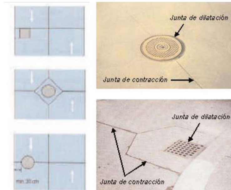
Figura 27. Croquis disposició de juntes de contracció i dilatació en pous de registre i arquetes.
