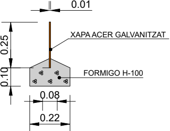
DETALL VORADA ACER GALVANITZAT PER ESCOCELLS E: 1/20
