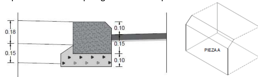
Figura 34. Detall vorada acabat bisellat
