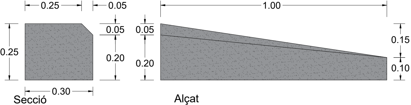
Peça especial transició tipus 1 Peça E
