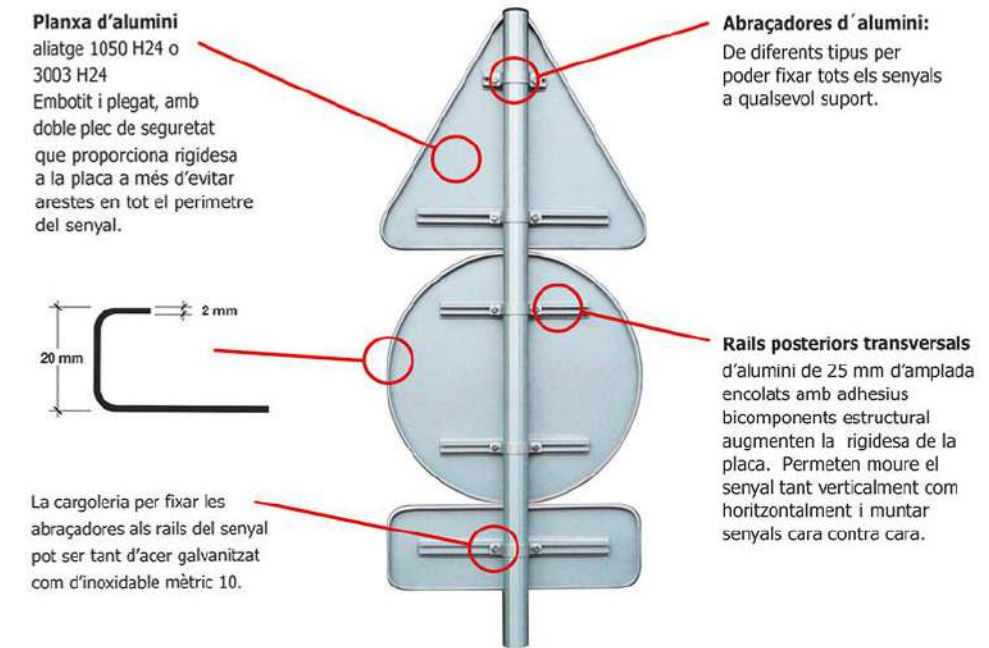
Figura 71. Característiques senyals verticals part posterior.
