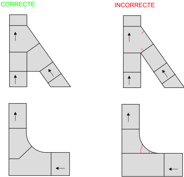
ESQUEMA DISTRIBUCIÓ JUNTES EN CREUAMENTS VIALS
