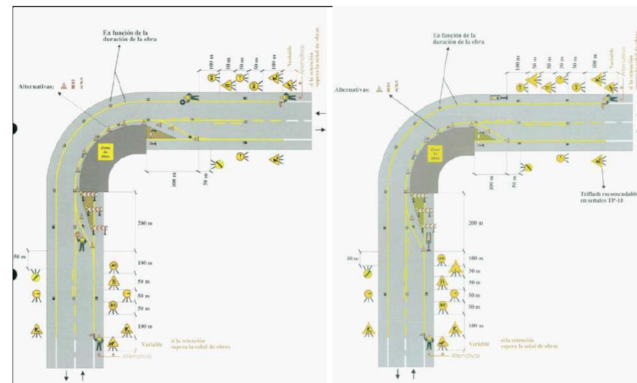
Figura 78. A) Treballs en corba amb pas alternatiu B) Treballs corba pas alternatiu (NIT)
