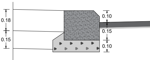
DETALL ENTREGA VORADA BISELLADA
