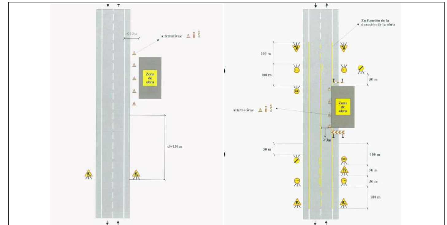
Figura 75. A) Treballs fora de la via. B) Ocupant la voravia i part de la calçada.
