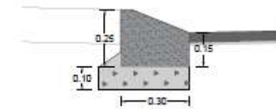
Figura 10. Detall peça granítica gual vehicles
