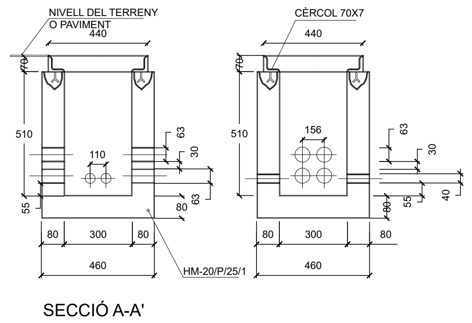
DIMENSIONS DE LA ARQUETA TIPUS M AMB TAPA DE FORMIGÓ
