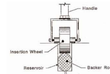
Figura 31. Esquema de instal·lació d'obturator de fons.
