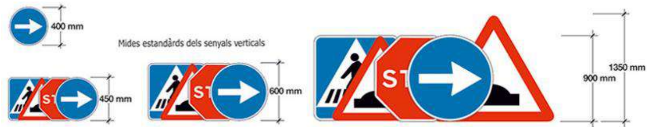
Figura 70. Diferents tipus de mides de senyals.
