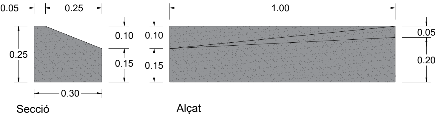
Peça especial transició tipus 2 PEÇA D
