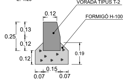
DETALL VORADA T-2 E: 1/20
