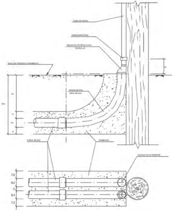
SORTIDA A POSTE O FAÇANA PER A RECONNEXIÓ D'ESCOMESA HABITATGE UNIFAMILIAR amb 2 conductes Ø63mm
