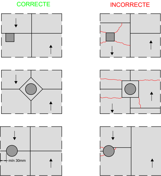
ESQUEMA DISPOSICIÓ DE JUNTES DE CONTRACCIÓ I DILATACIÓ EN POUS DE REGISTRE, ARQUETES, EMBORNALS,...
