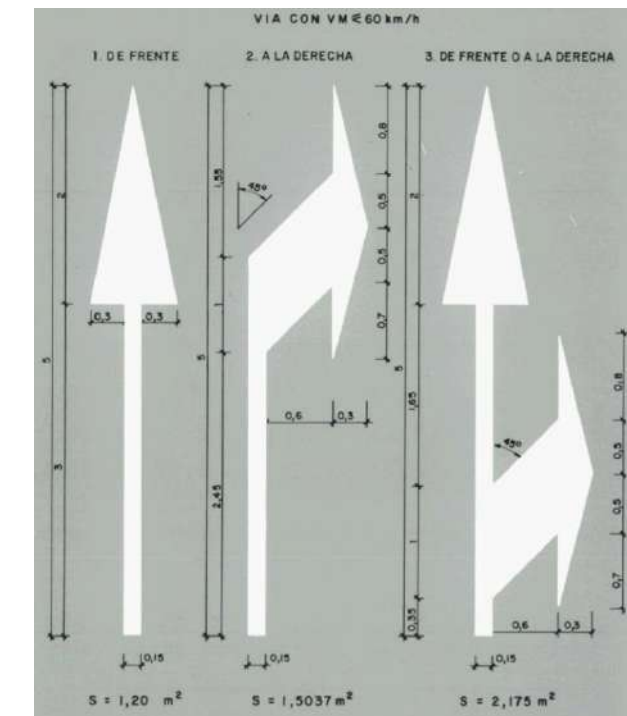
Figura 66. M5.2– Fletxes de selecció de carril.
