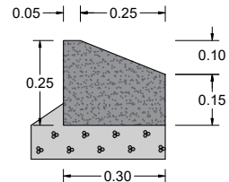
DETALL RIGOLA GRANÍTICA ENCINTAT DE 30x40x15 cm E: 1/20
