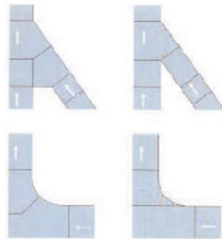
Figura 28. Disseny de juntes en creuament on en presència d'elements rígids.
