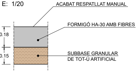
DETALL FIBRES DE VIDRE TIPUS V12-AM DE FIBRATEC O EQ
