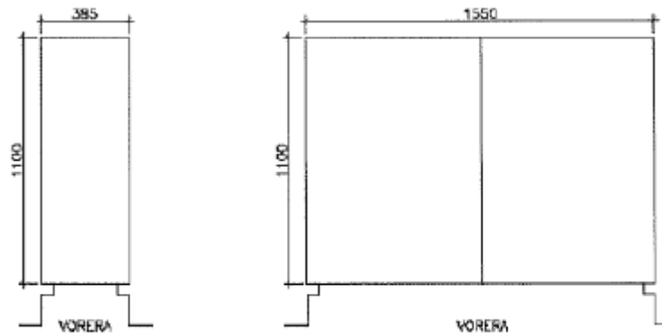
Figura 2 : Armari d'intempèrie TIPUS 2
