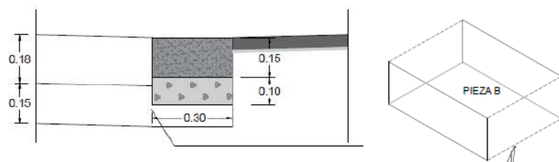
Figura 36. Detall rigola per a gual peatonal.
