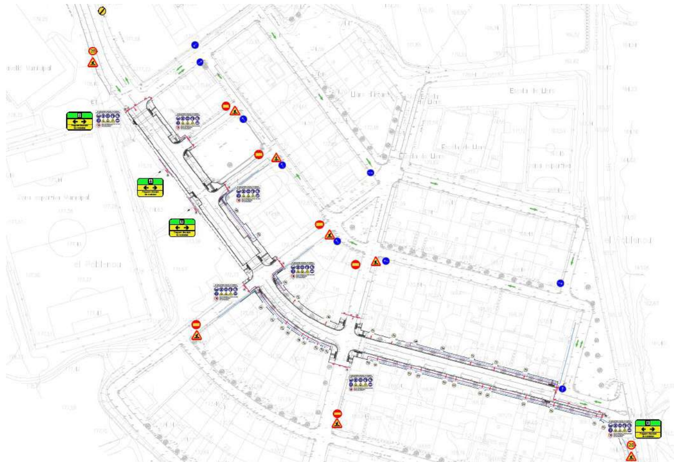
Figura 85. Plànol senyalització provisional d'obra.
