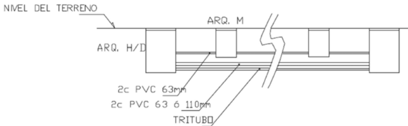
ESQUEMA SECCION DE CANALIZACION
