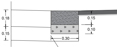
DETALL ENTREGA ESCOCELL
