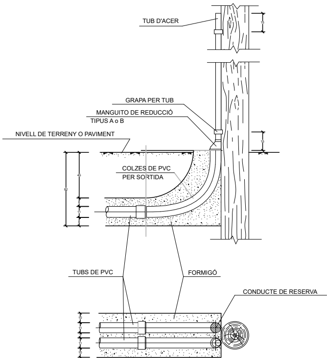
SORTIDA A POSTE O FAÇANA PER A RECONNEXIÓ D'ESCOMESA HABITATGE PLURIFAMILIAR O CONNEXIÓ A LÍNIA AÈRIA amb 2 conductes Ø110mm
