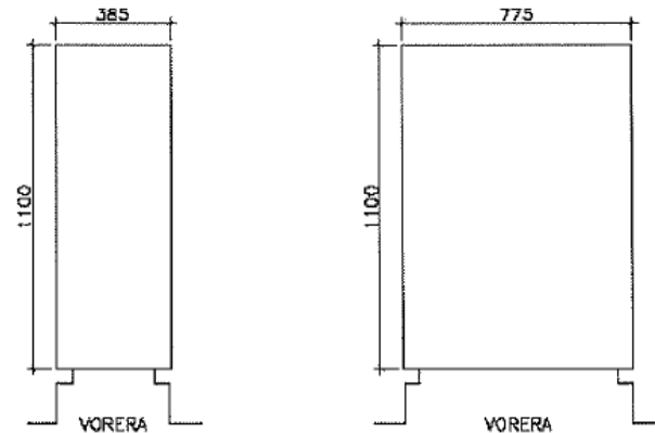
Figura 1 : Armari d'intempèrie TIPUS 1
