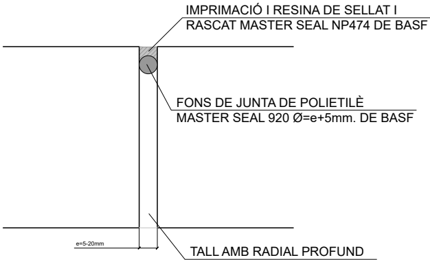
DETALL JUNTA PERIMETRAL AMB ELEMENT RÍGID E: 1/15
