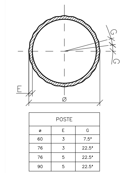
5 SECCIÓ A-A'
