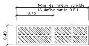
PLANTA REIXA
