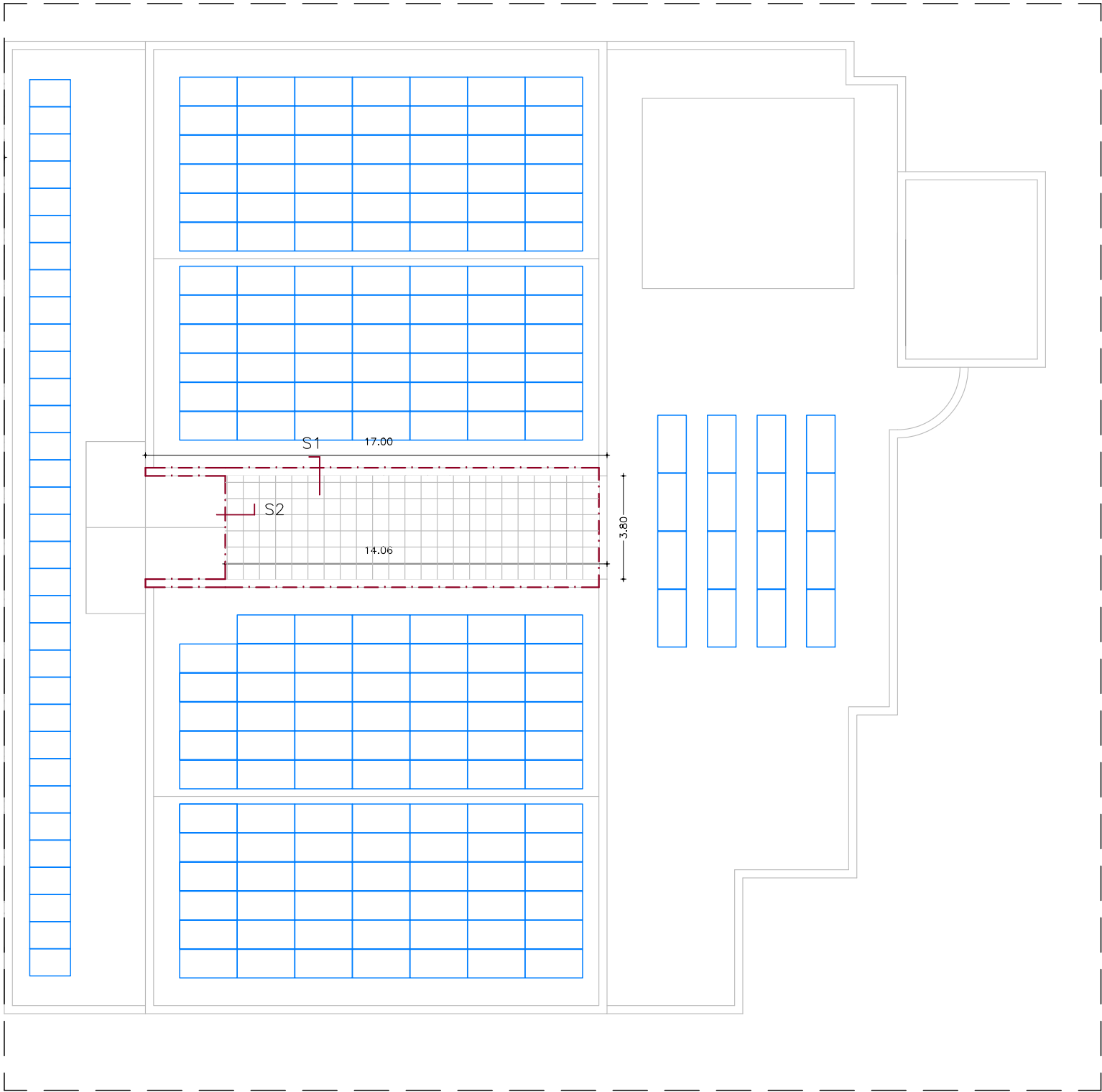
PROPOSTA. PLANTA COBERTA MUSEU
