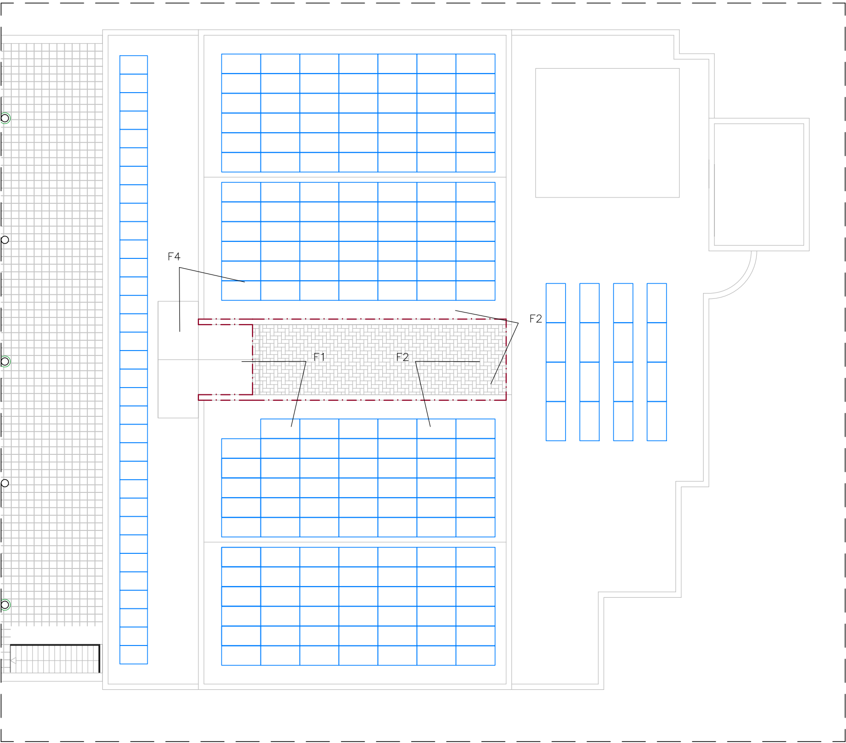
ESTAT ACTUAL. PLANTA COBERTA MUSEU
