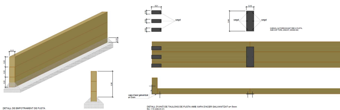
Figura 6. Detall fusteria
