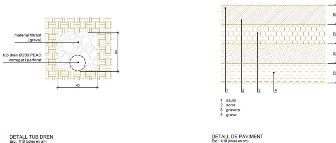
Figura 4. Detall drenatge i paviment
