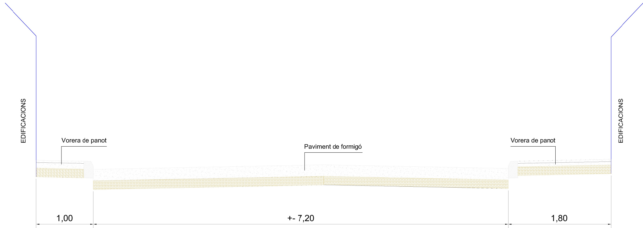
SECCIÓ ACTUAL
