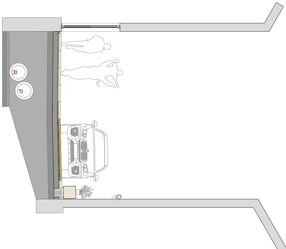
SECCIÓ TÍPUS PROJECTE
