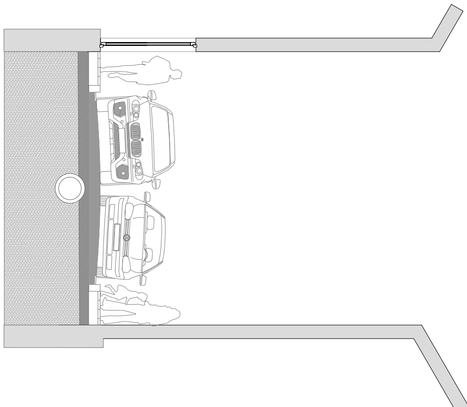
SECCIÓ TÍPUS ORIGINAL
