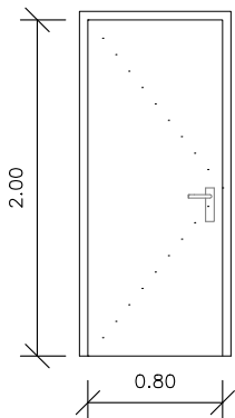
Porta d'una fulla batent, bastiment 10cm 3u amb condemna
