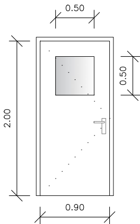
Porta d'una fulla batent Finestra de vidre transparent
