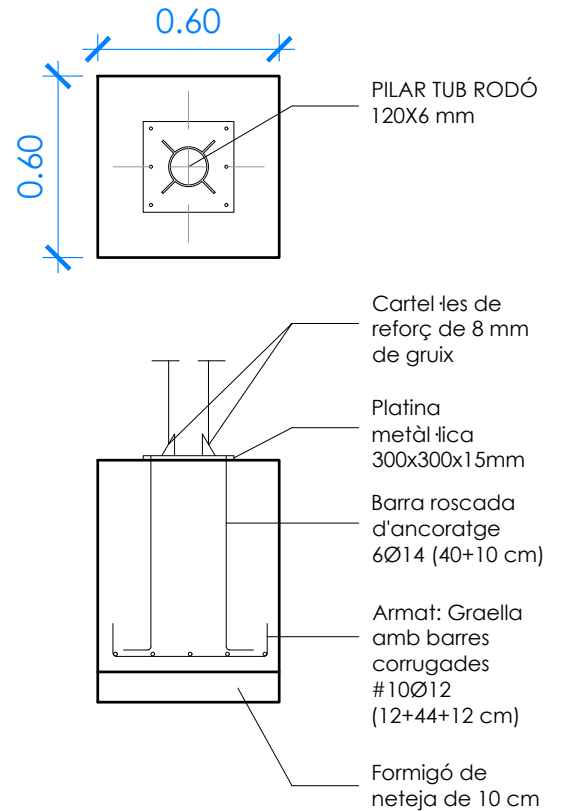
2 DETALL PILAR CENTRAL ESTAT PROPOSTA E:1/25
