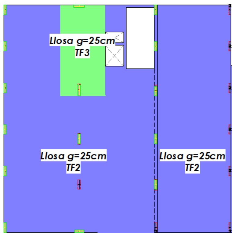
DB SE-AE-PI. Baixa
