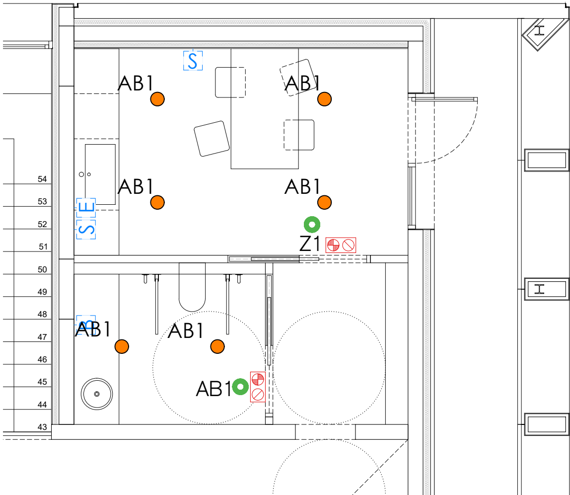
PLANTA ELECTRICITAT I ENLLUMENAT. OFFICE I BANY P1
