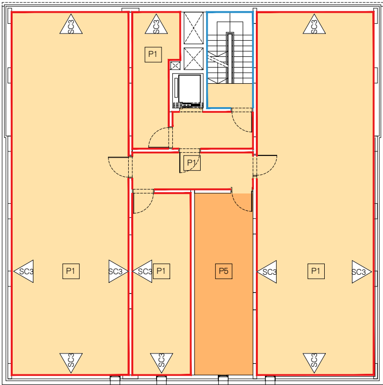
Planta soterrani 1
