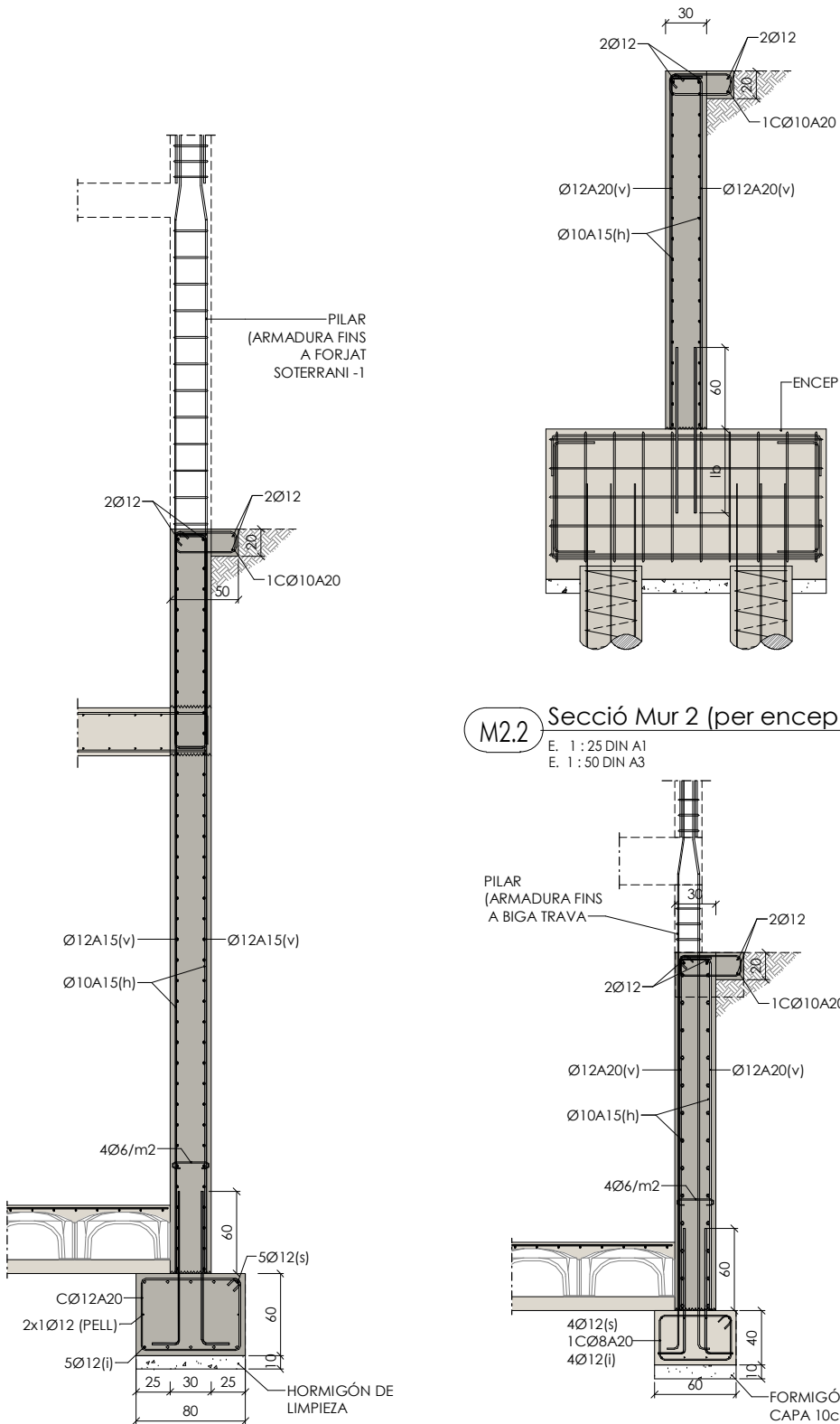
M1 Secció Mur 1
