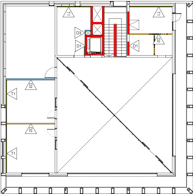
Planta primera
