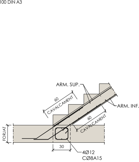
Arrencada escala a forjat
