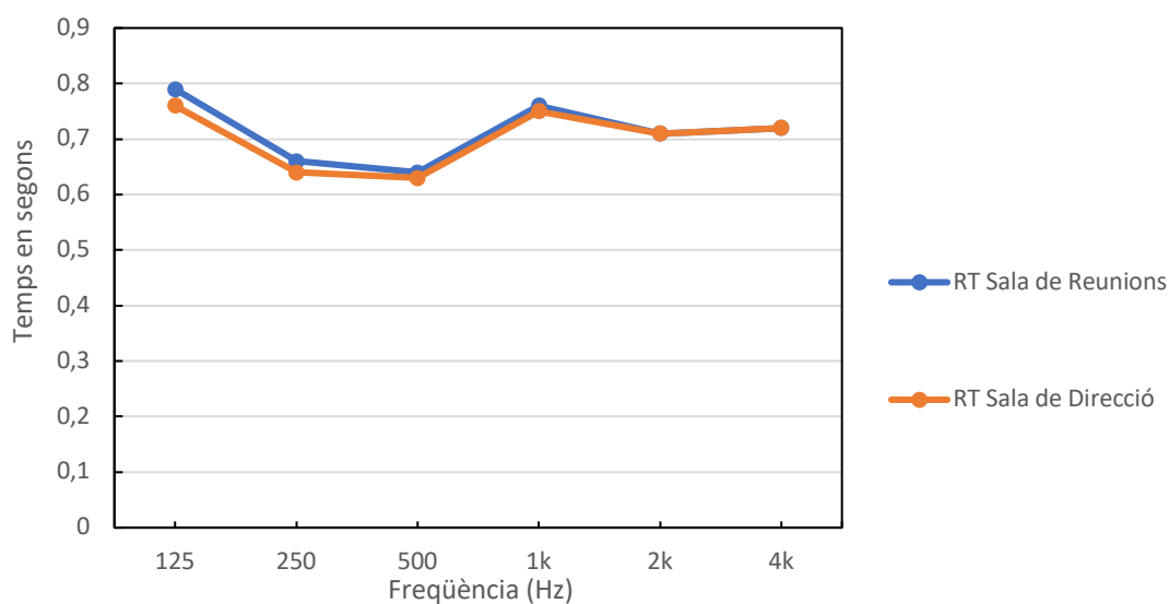
RT Sales de Reunions i Direcció
