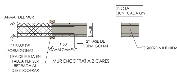
Junt de formigonat en mur
