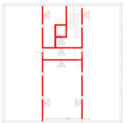
Planta soterrani 2
