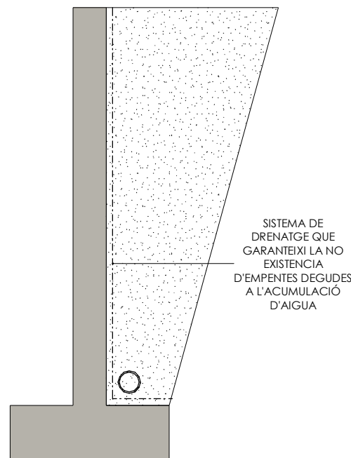
Drenatge en murs
