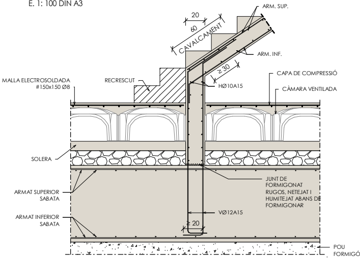
Arrencada escala en sabata
