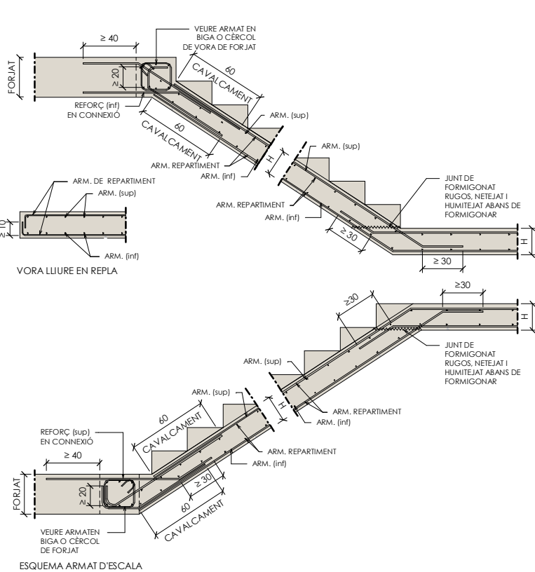
Arrencada escala a forjat
