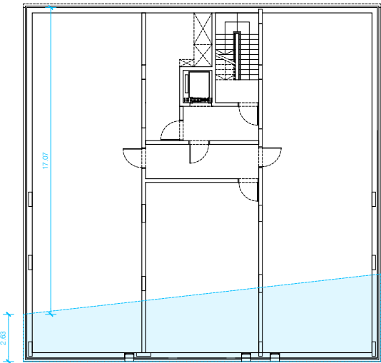
PLANTA SOTERRANI -2
