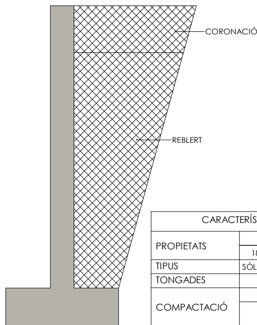
Reblert en murs
