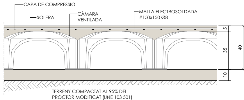
Secció forjat cavitat
