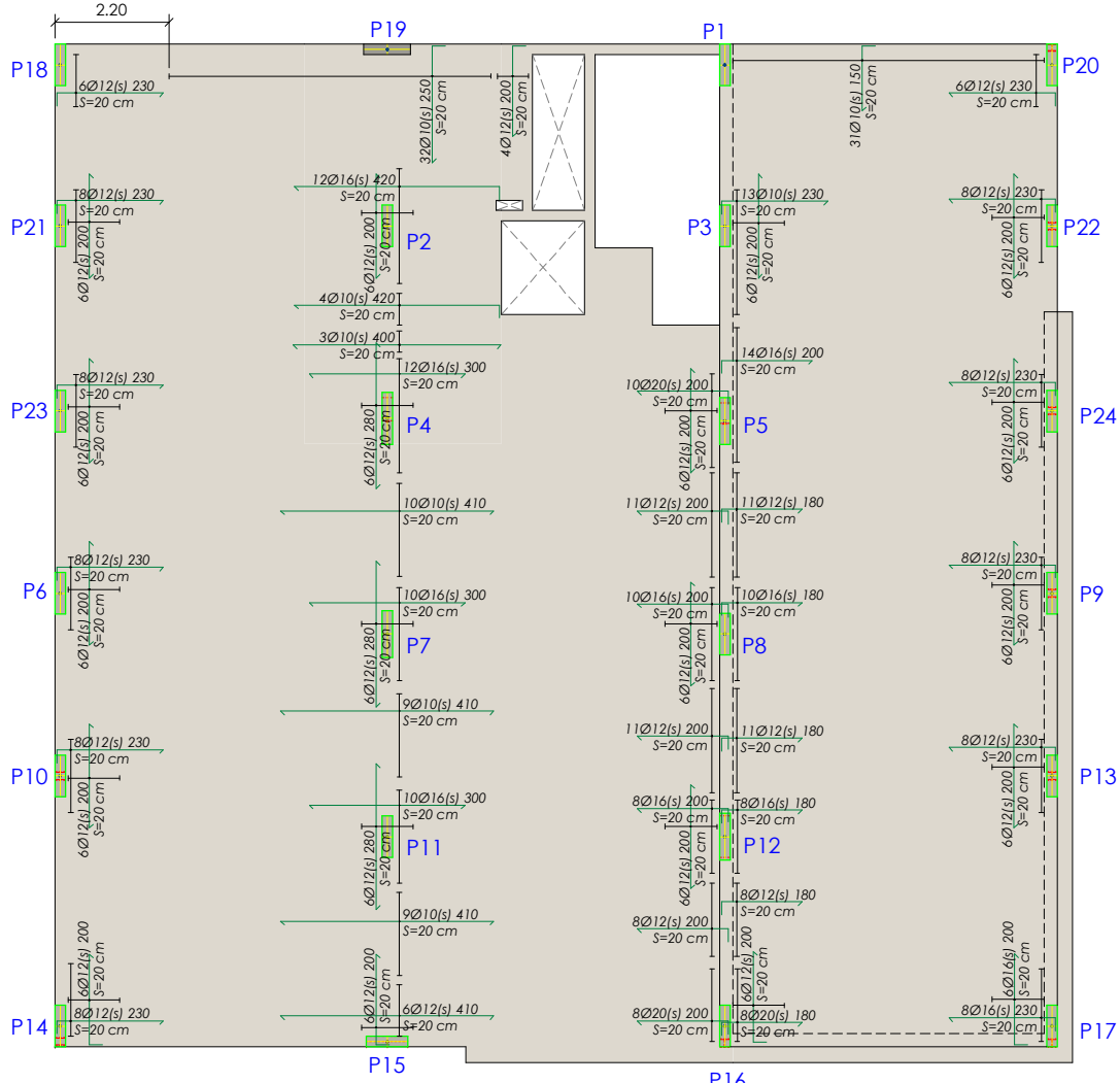
Sostre Pl. Soterrani-1 - Reforç superior
