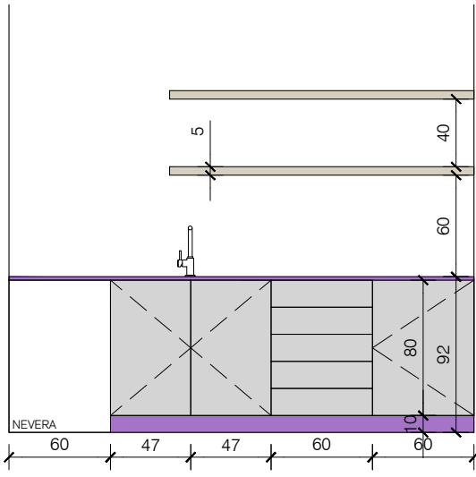
ALÇAT FRONTAL
