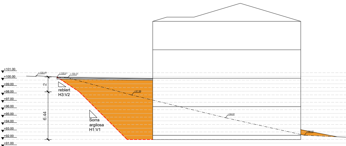
SECCIÓ 4
