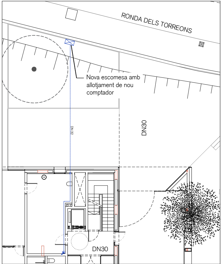
ZONA EXTERIOR E: 1/200
