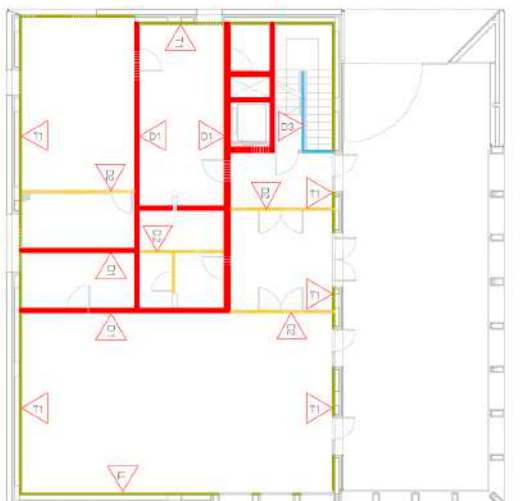
Planta baixa
