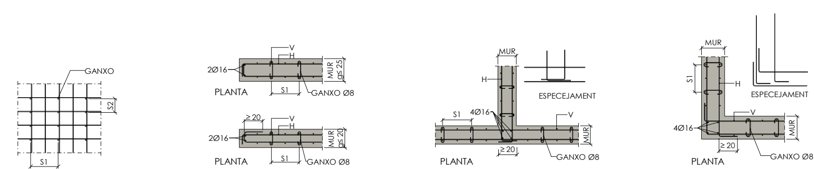
Especejament armat
