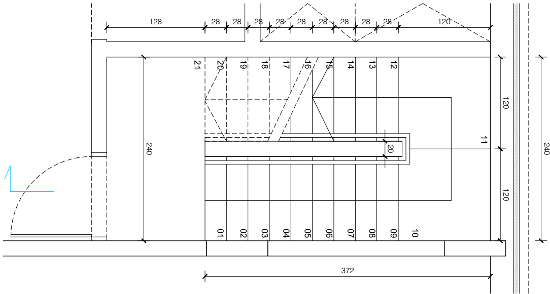
PLANTA ARRENCADA ESCALA DE P-2 A P-1
