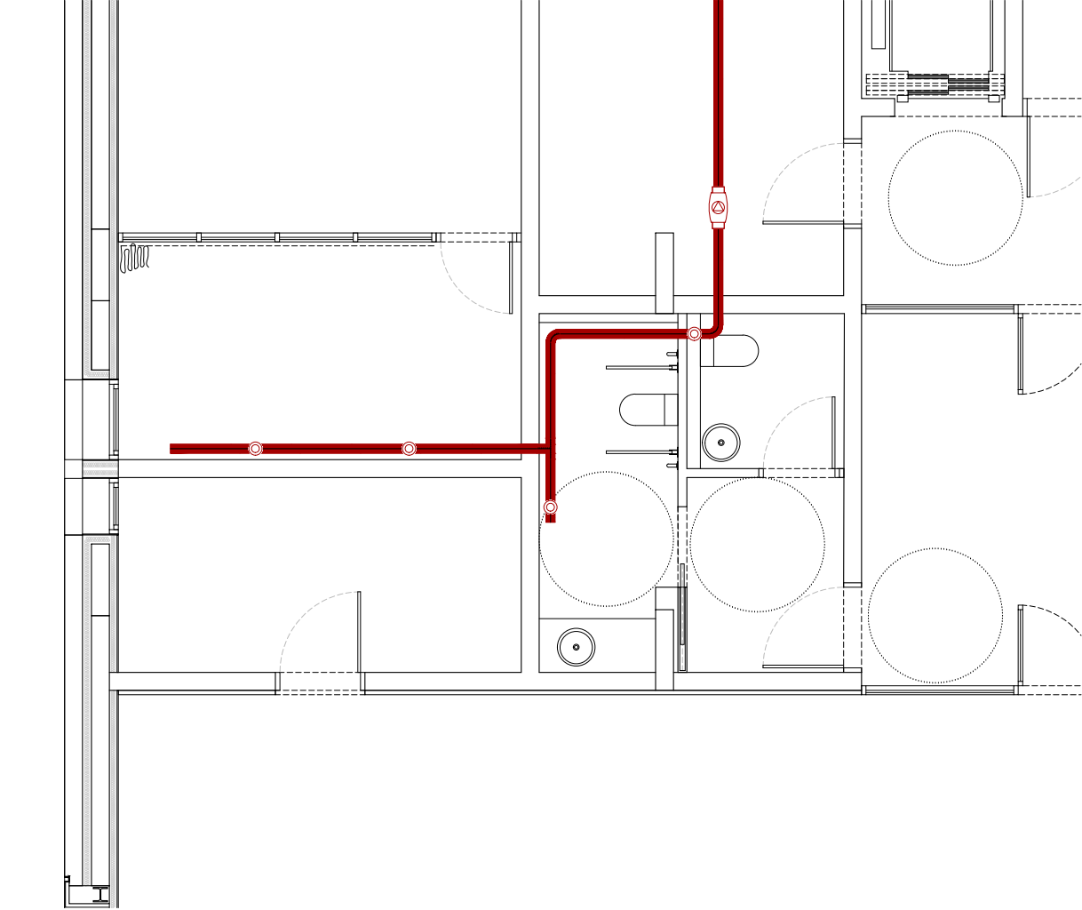
PLANTA CLIMA I VENTILACIÓ. BANYS PB I SALA DESINSECTACIÓ
