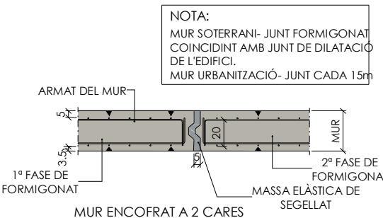
Junta de dilatació en mur
