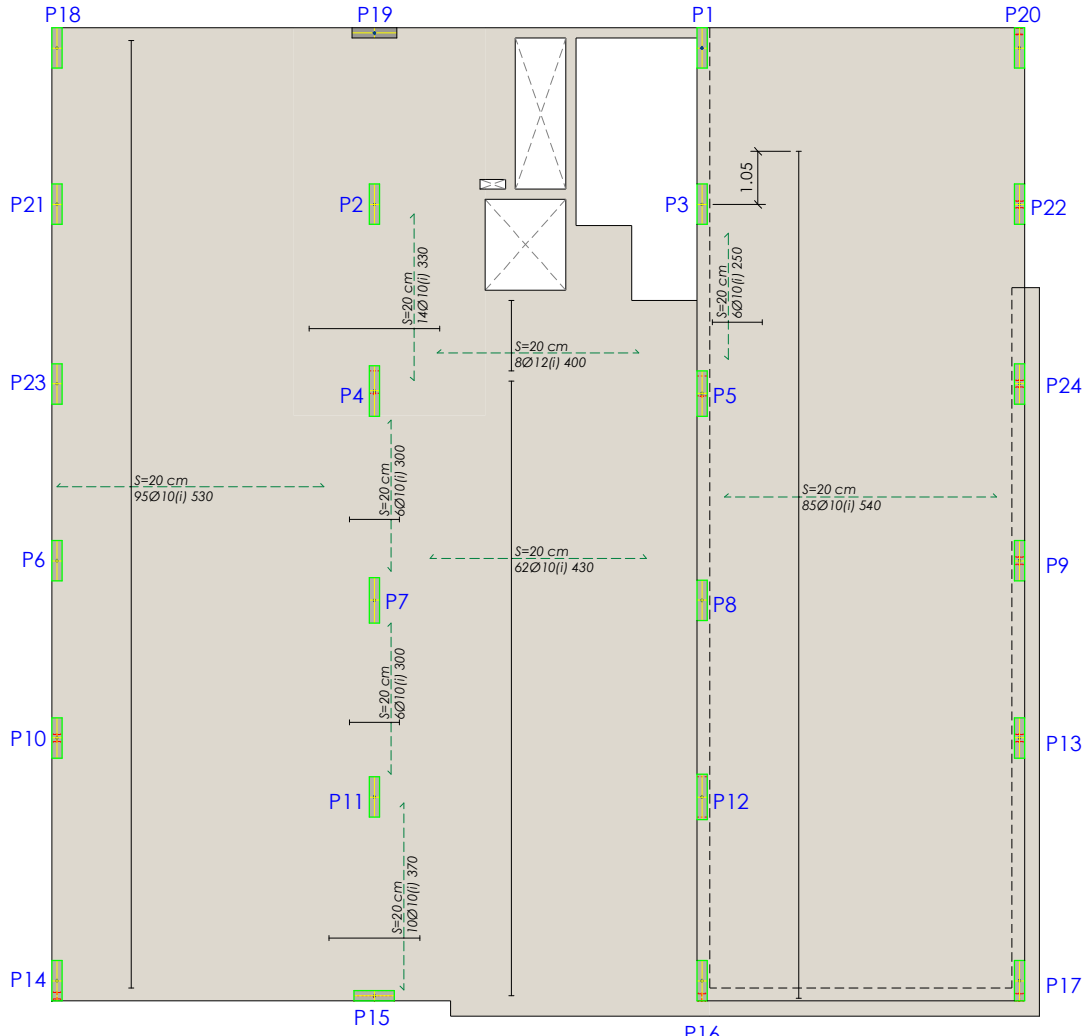
Sostre Pl. Soterrani-1 - Reforç inferior
