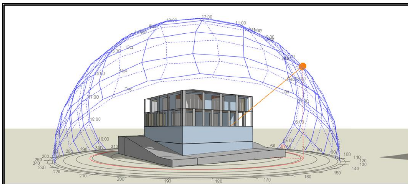
Imatge del software DesignBuilder, visualització del recorregut solar
