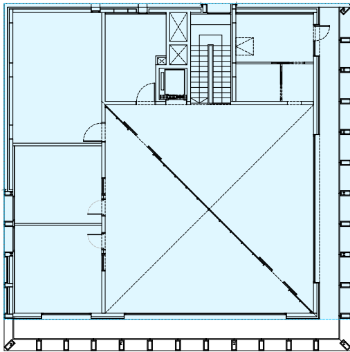
PLANTA PRIMERA
