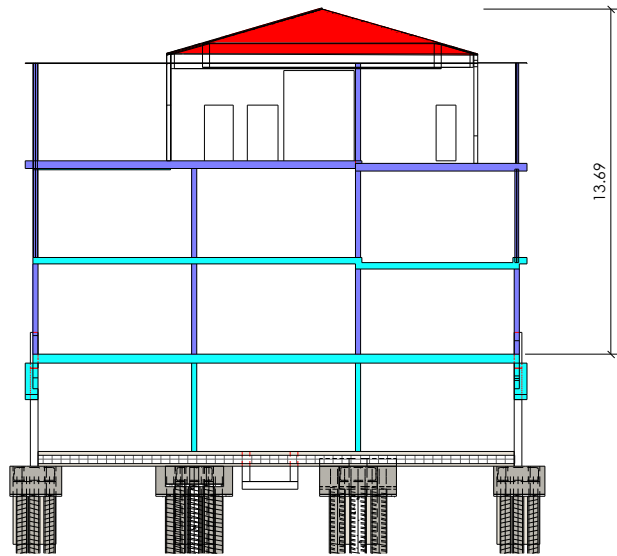
SX Secció DB SI-S6
