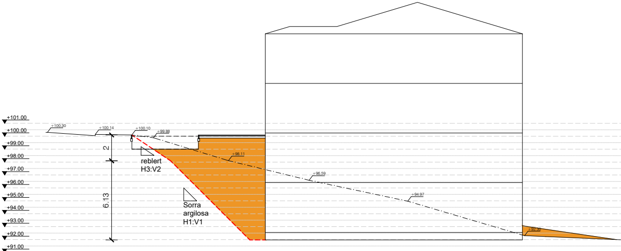
SECCIÓ 6
