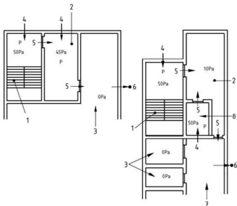
10a Presurización de escalera y de todos los vestíbulos anexos. 10b Presurización de escalera y del pozo de ascensor
