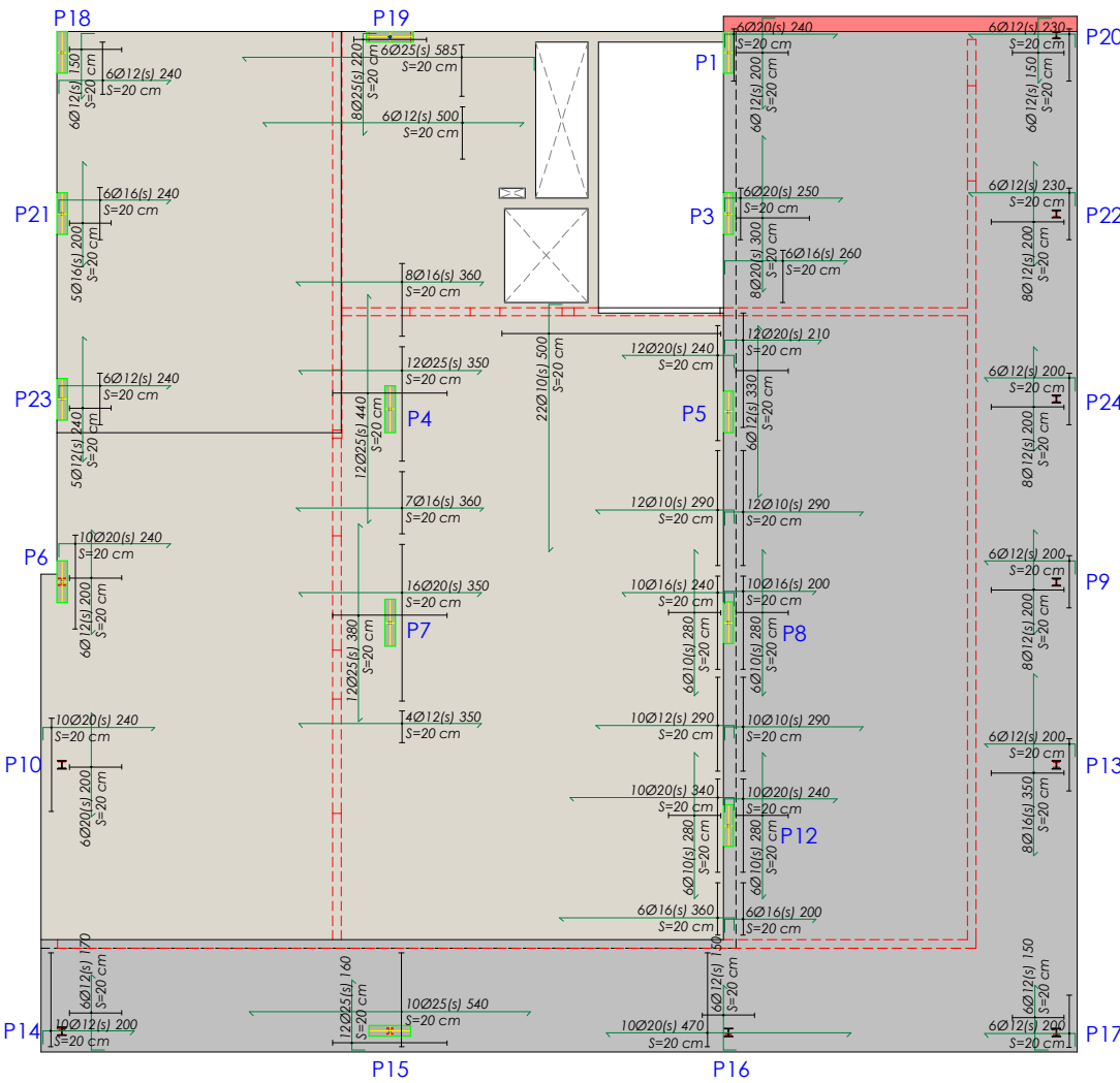
Sostre Pl. Baixa - Reforç superior
