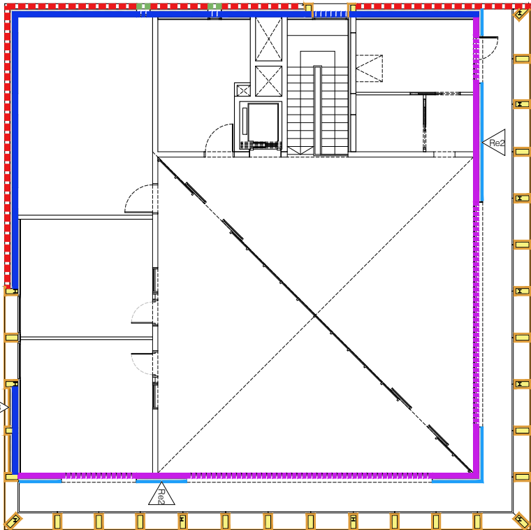
Planta primera
