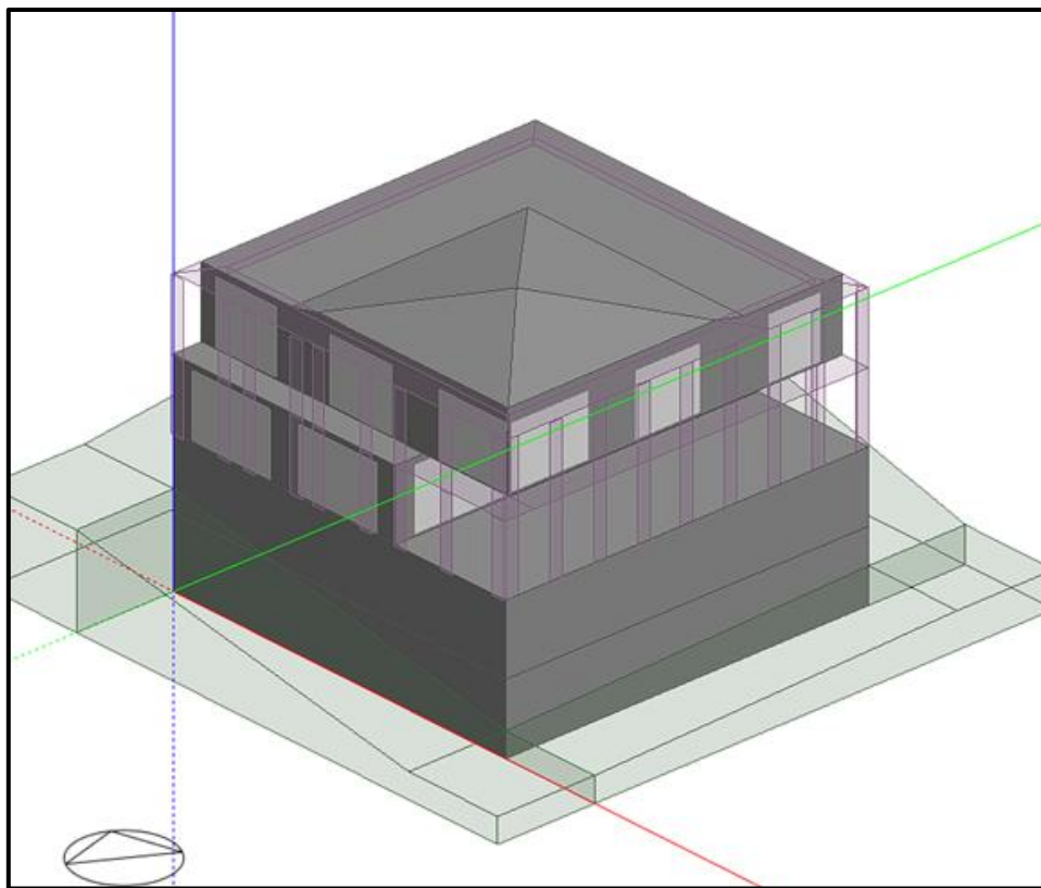
Model de càlcul, geometria exterior i elements de protecció solar
