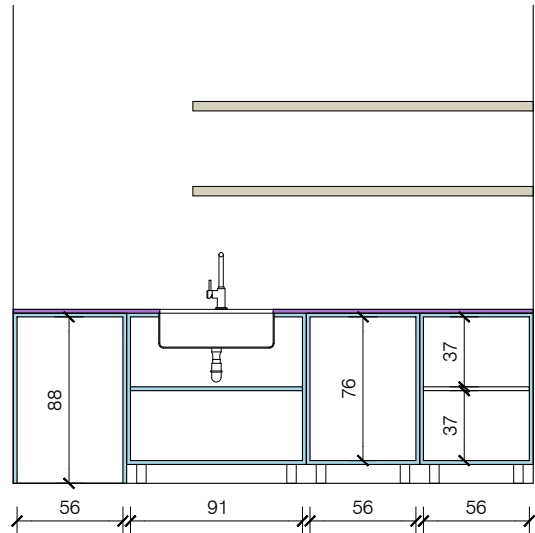
SECCIÓ 1
