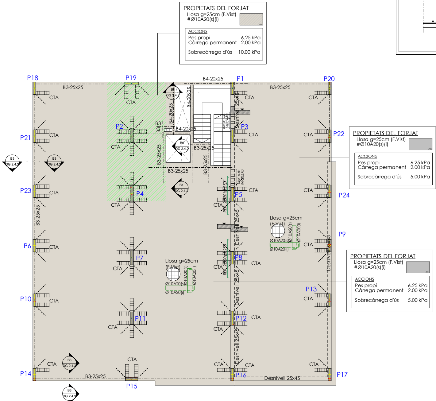
Sostre Pl. Soterrani-1 - Armadura general
