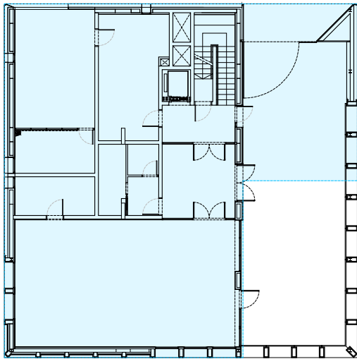
PLANTA BAIXA
