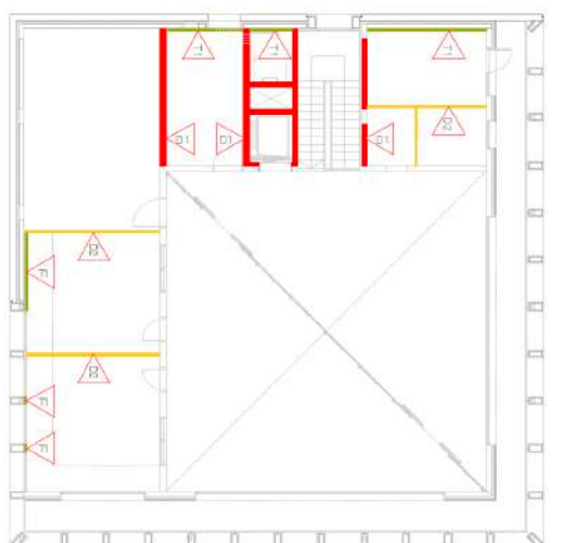
Planta primera
