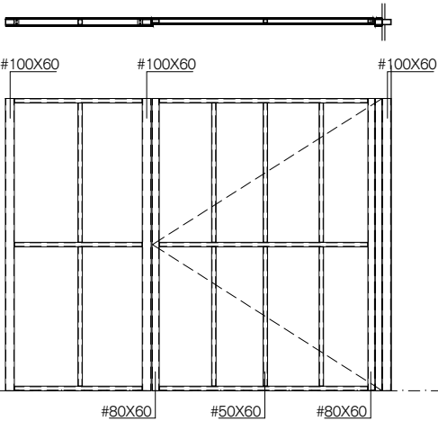
Detall estructura interior porta
