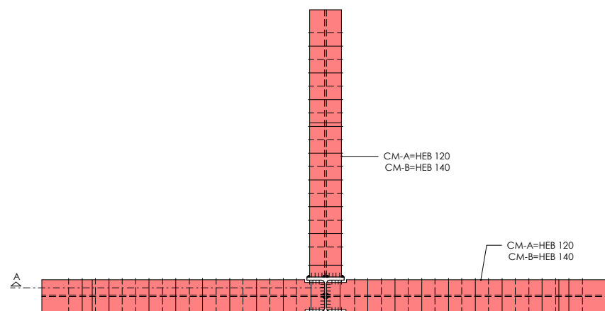
Detall creueta formigó
