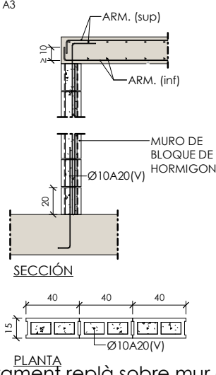
Recolzament replà sobre mur de bloc
