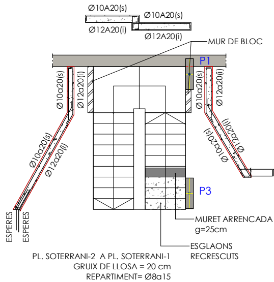
Escala de PI.Soterrani-2 a PI.Soterrani-1
