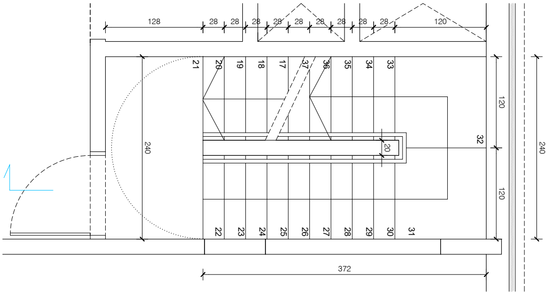
PLANTA ARRENCADA ESCALA DE P-1 A PB
