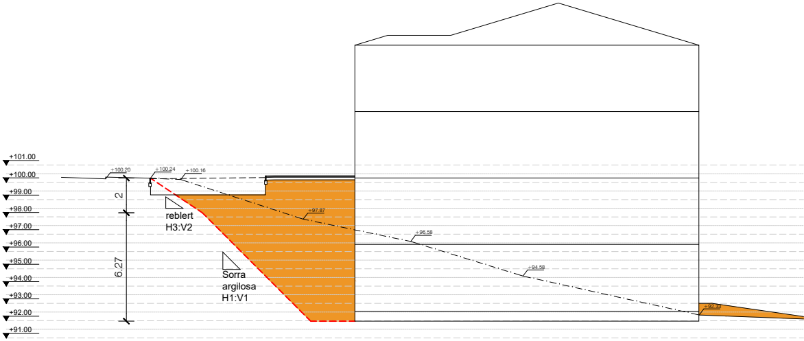
SECCIÓ 5
