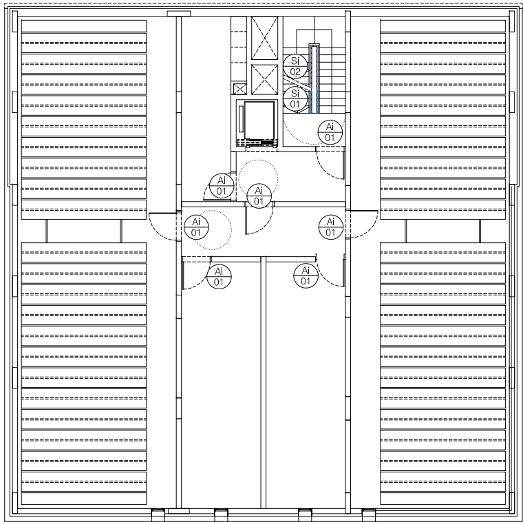
Planta soterrani 1
