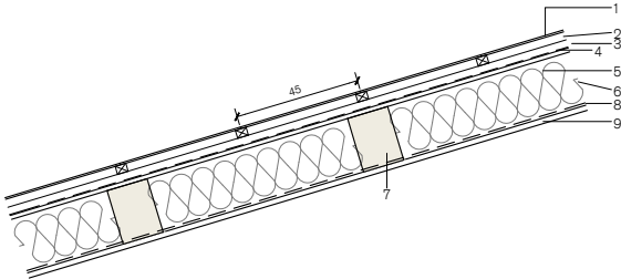
C1. Coberta inclinada E/ 1:30
