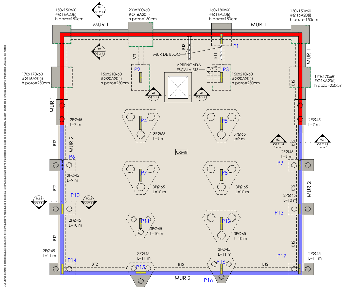
Planta Cimentación
