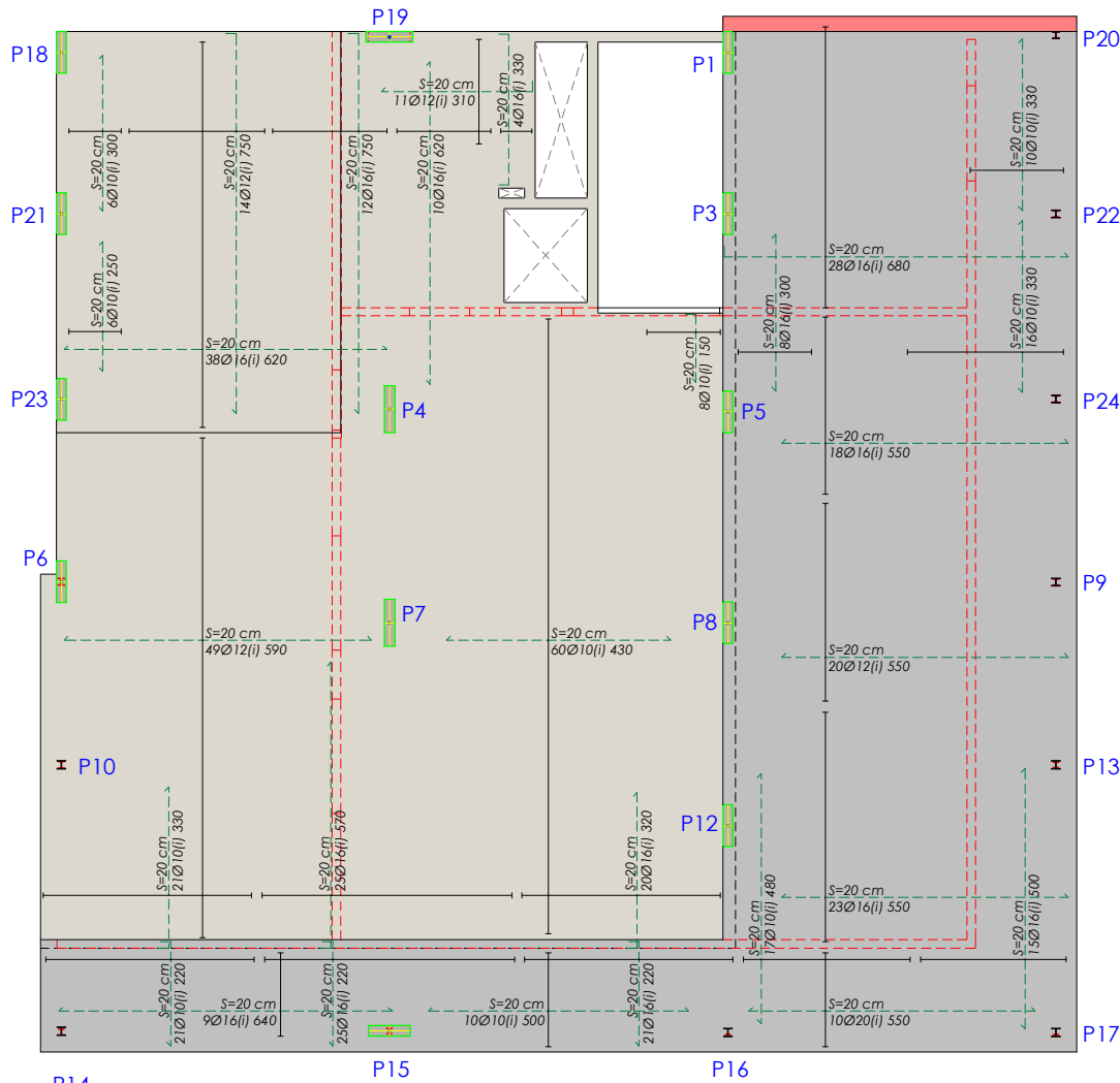
P14 Sostre Pl. Baixa - Reforç inferior
