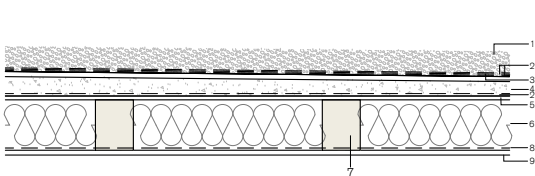
C2. Coberta plana convencional E/ 1:30
