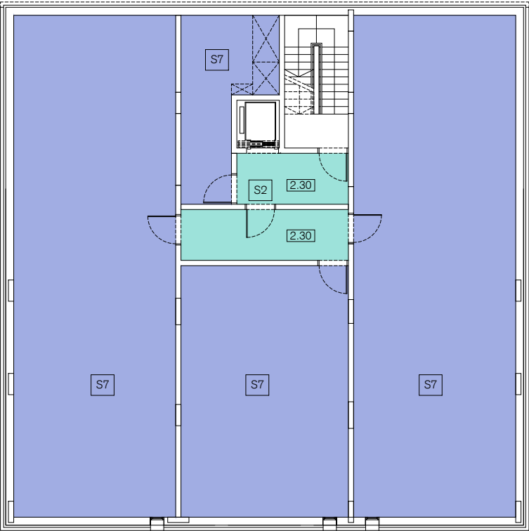
Planta soterrani 2
