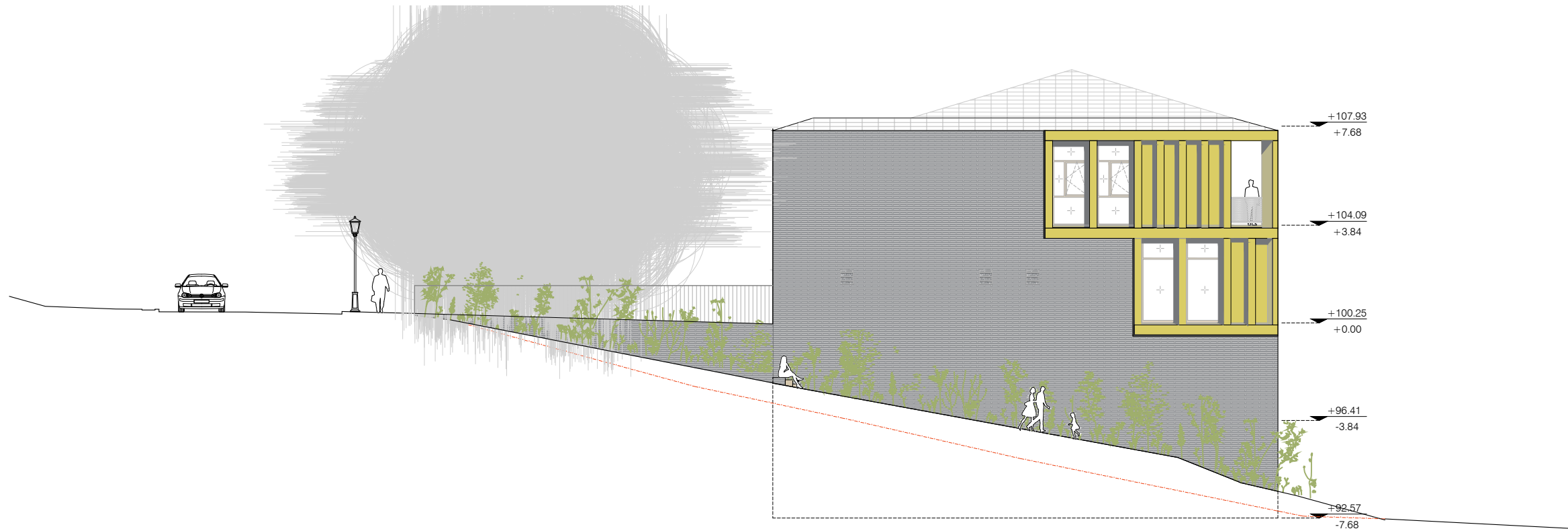
ALÇAT NORD - OEST
