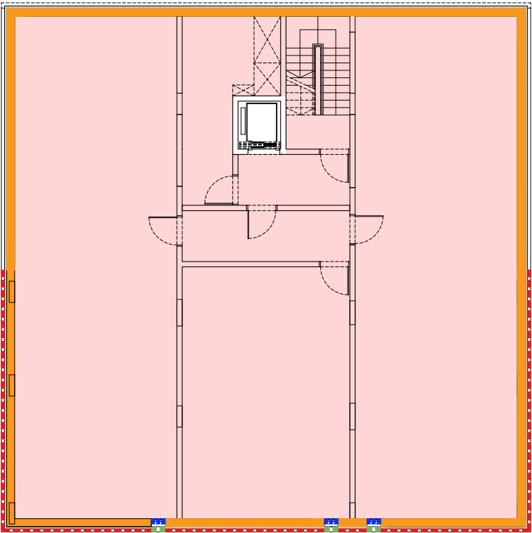
Planta semi soterrani 2
