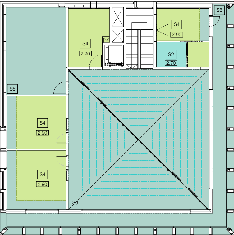
Planta primera
