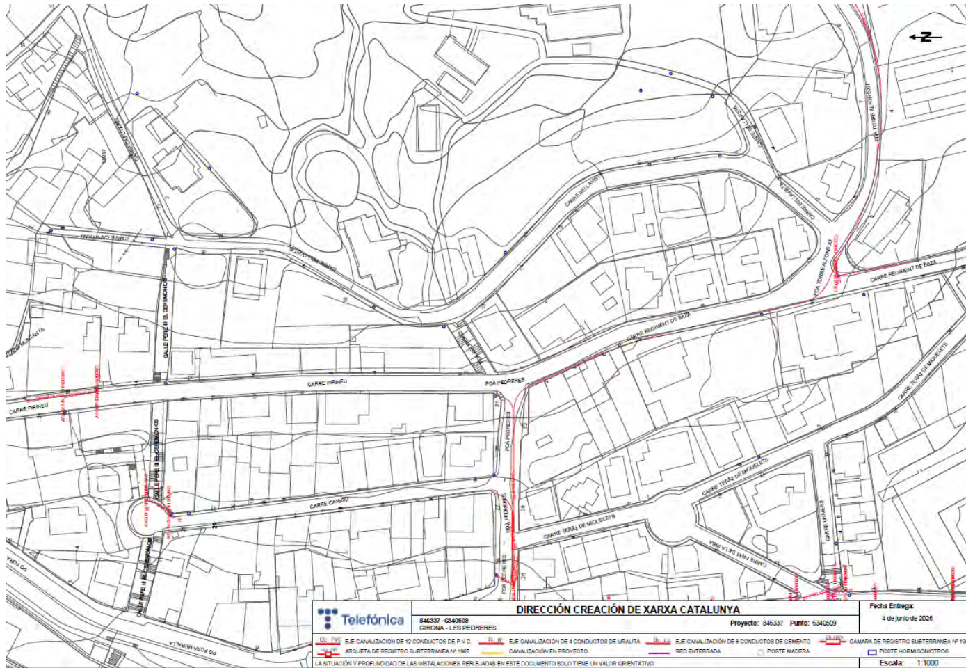
Figura 20. Plànol xarxa telefonia existent – ACEFAT.
