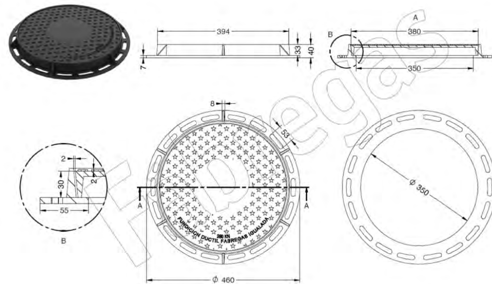
Figura 49. Tapa de registre B-6DU de Fàbregas, per a vàlvules de comporta \varnothing < 80 mm.
