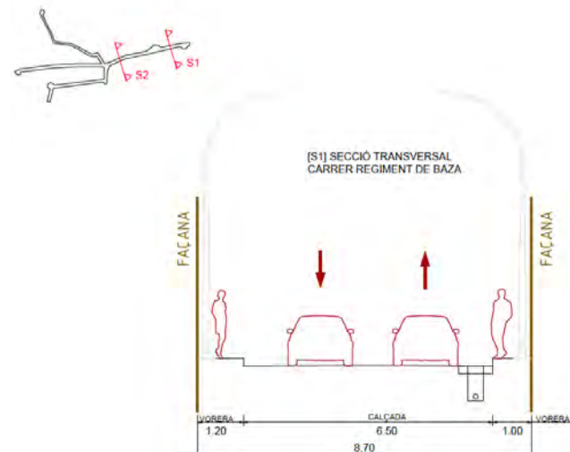
Figura 27. Secció transversal Carrer del Regiment de Baza.
