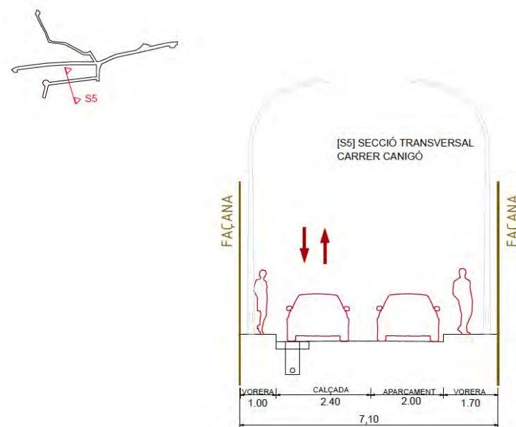
Figura 31. Secció transversal carrer Canigó.
