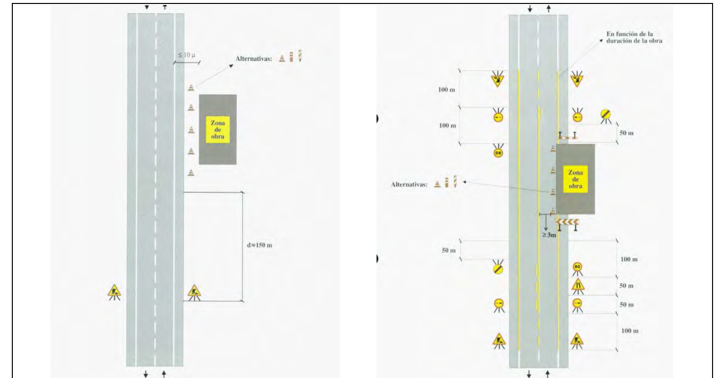
Figura 54. A) Treballs fora de la via. B) Ocupant la voravia i part de la calçada.
