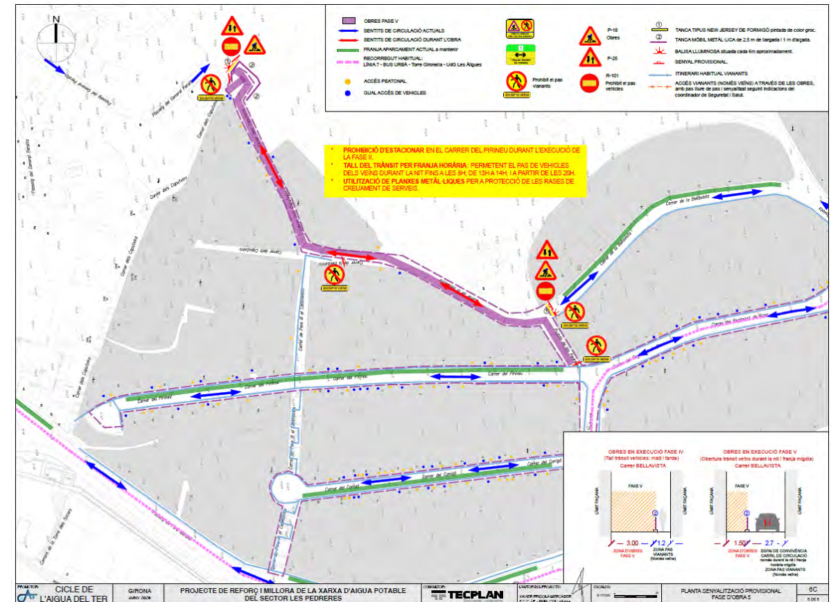
Figura 64. Planta senyalització provisional Fase d'obra 5
