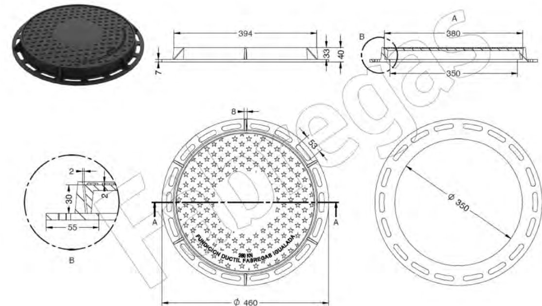
Figura 42. Tapa de registre B-6DU de Fàbregas, per a vàlvules de comporta Ø < 80 mm.
