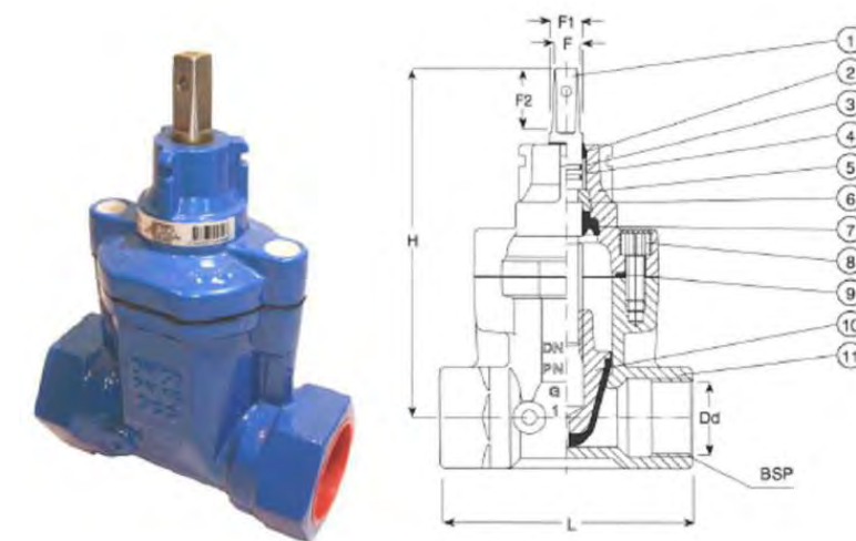
Figura 52. Imatge vàlvula de registre a instal·lar a peu de façana, segons fitxes tècniques.
