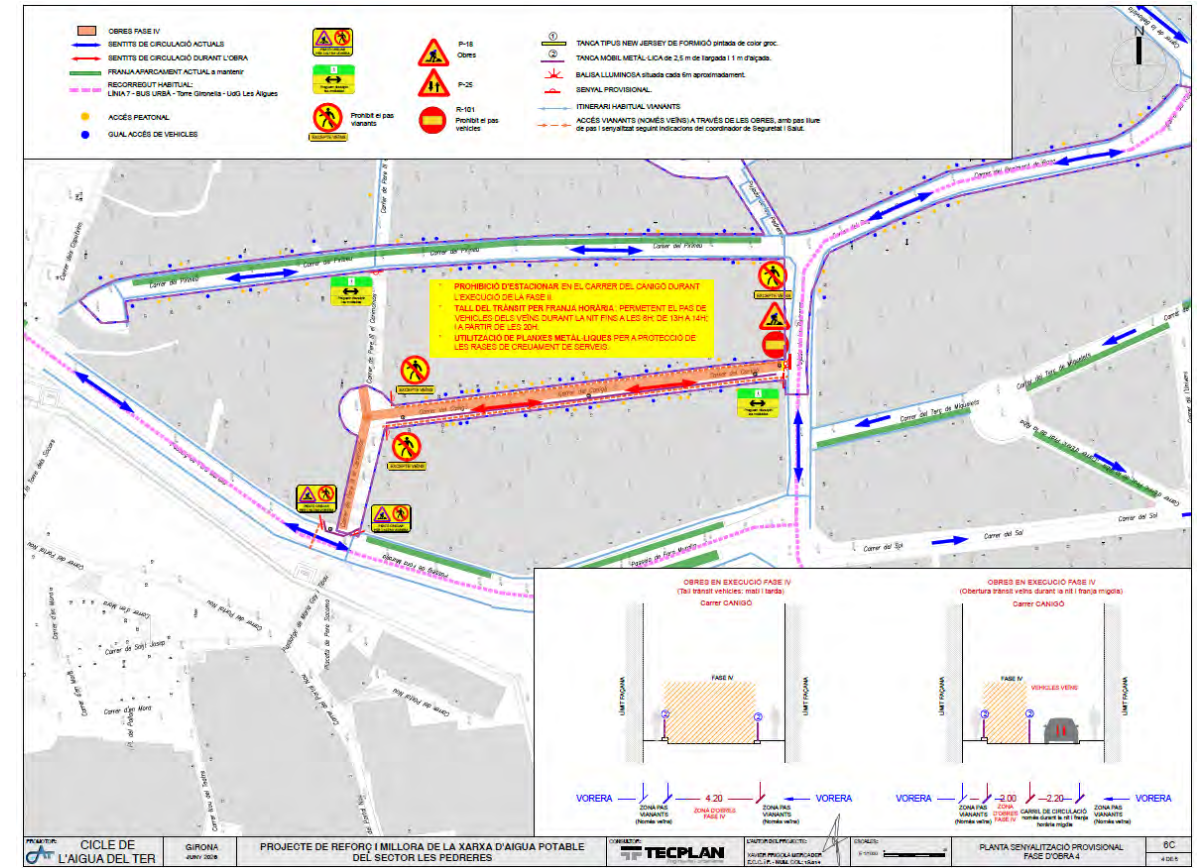
Figura 63. Planta senyalització provisional Fase d'obra 4
