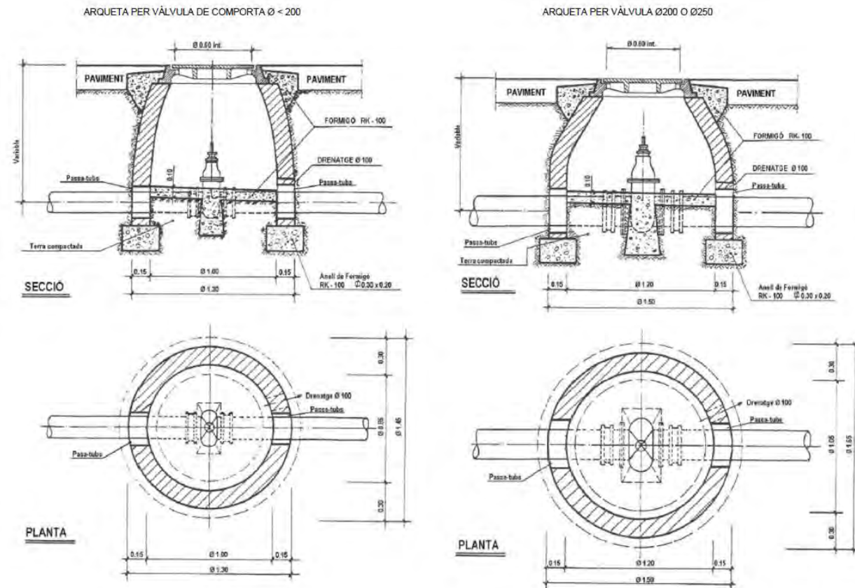
Figura 50. Detall pou de registre per a vàlvula de comporta \varnothing > o = a 80 mm.
