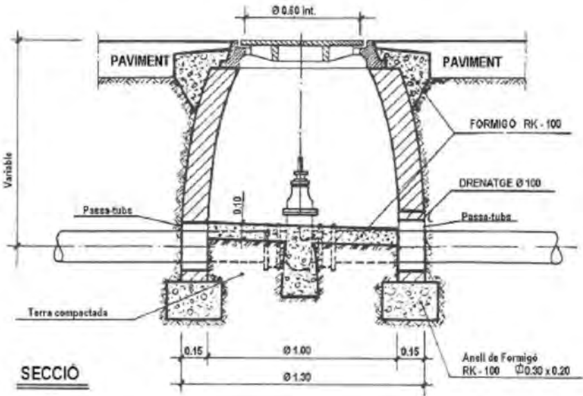
ARQUETA PER VÁLVULA DE COMPORTA Ø < 200
