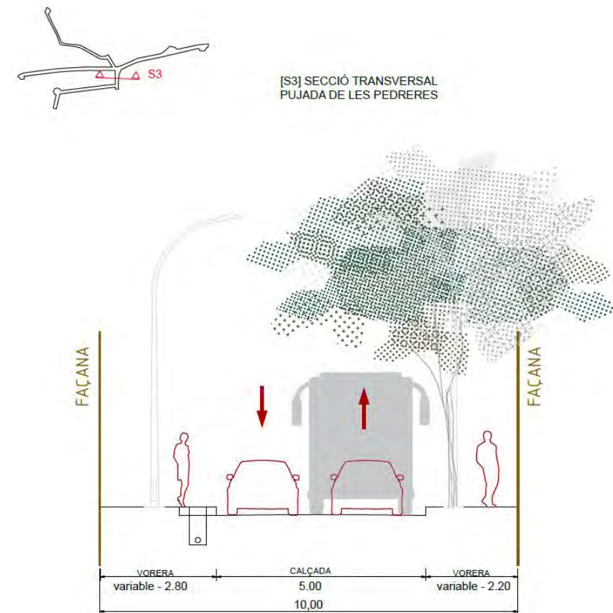
Figura 29. Secció transversal Pujada de les Pedreres.
