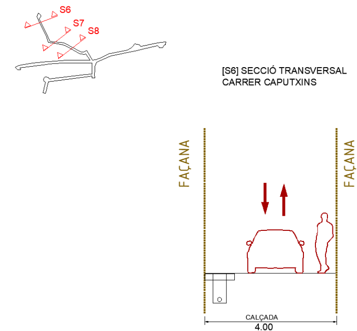
Figura 32. Secció transversal carrer Caputxins
