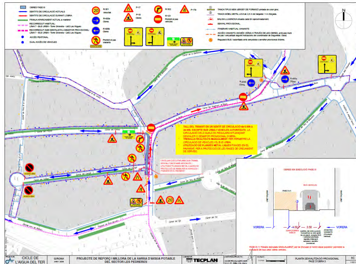
Figura 62. Planta senyalització provisional Fase d'obra 3
