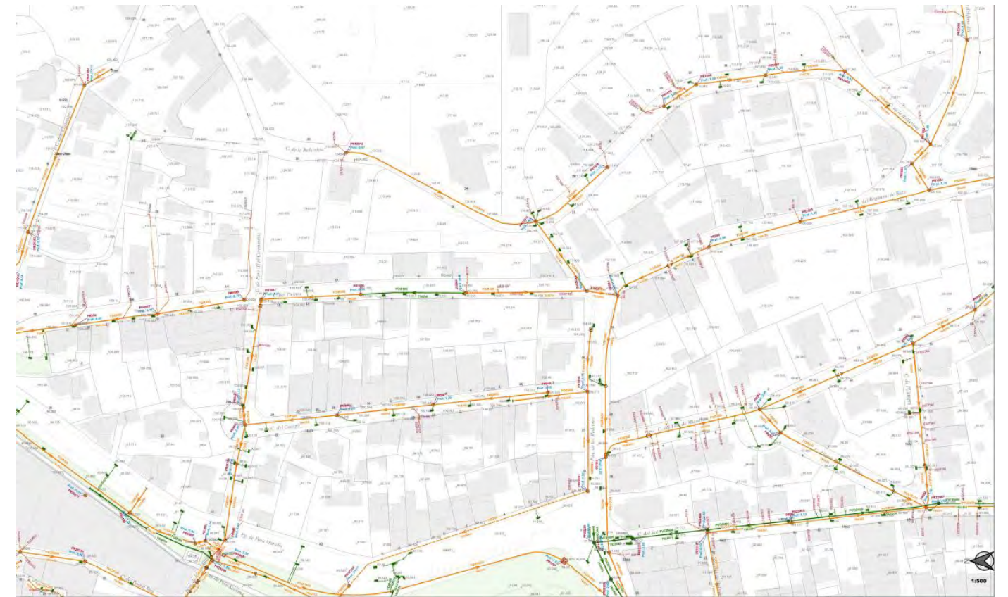
Figura 16. Plànol xarxa drenatge i clavegueram existent – Cicle de l'Aigua del Ter, S.A.
