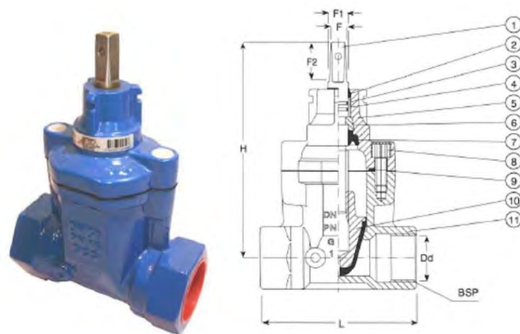
Figura 45. Imatge vàlvula de registre a instal·lar a peu de façana, segons fitxes tècniques.
