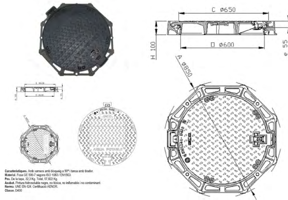
Figura 44. Tapa de registre tipus GEO D400 de EJ o equivalent.
