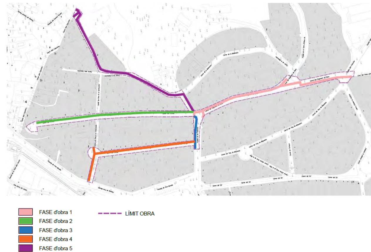
Figura 53. Plànol FASES D'OBRA.
