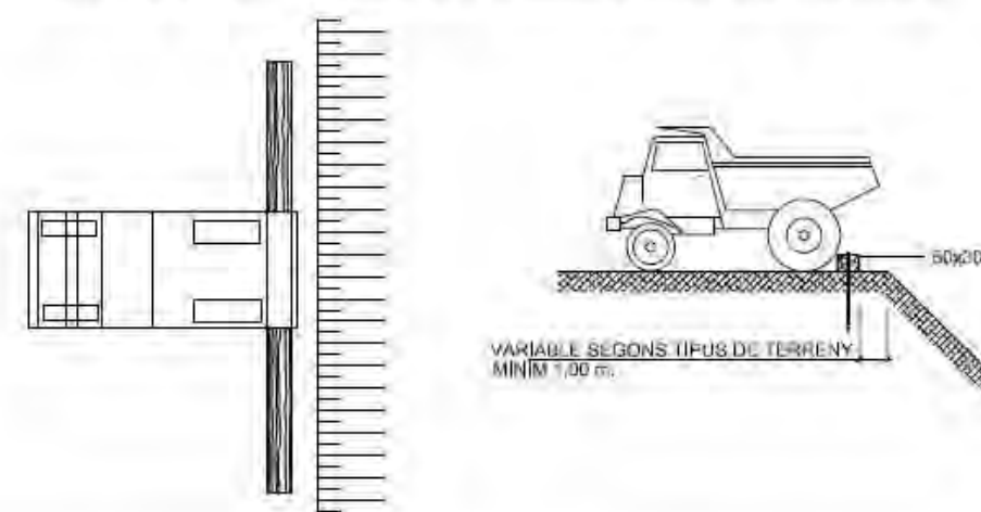
Proteccions col·lectives: DESMUNTS, TERRAPLENS I VESSAMENT DE TERRES
