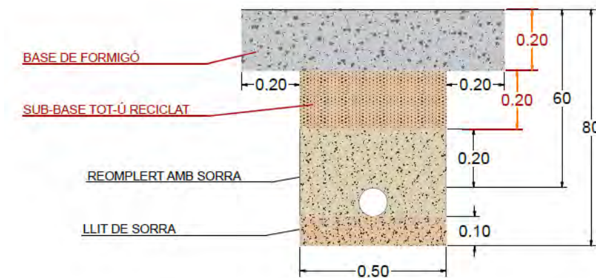
Figura 39. Execució capa de formigó fins a cota rasant.
