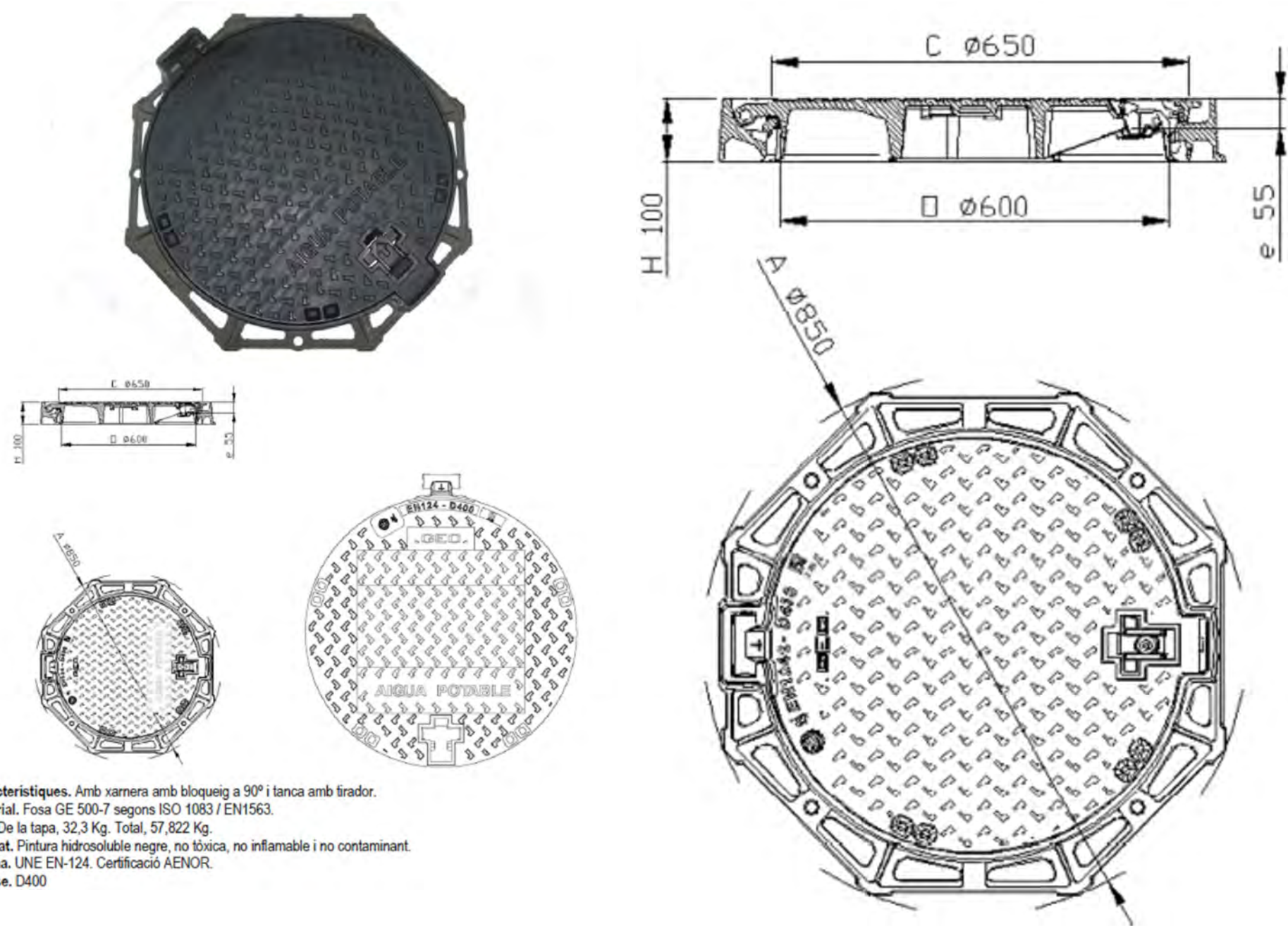
TAPA AIGUA FOSA DÚCTIL Ø600 mm TIPUS EJ MODEL GEO D400 o equivalent
