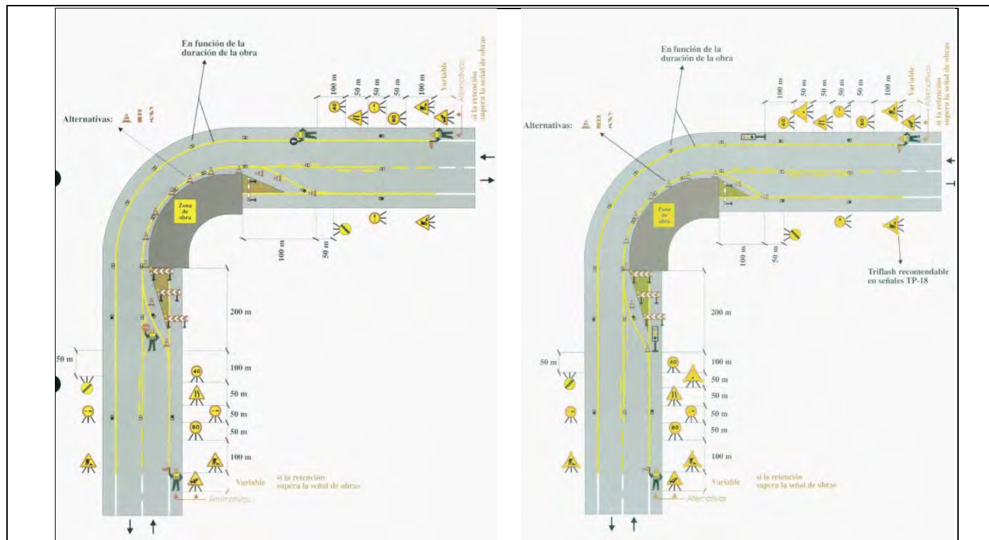
Figura 57. A) Treballs en corba amb pas alternatiu B) Treballs en corba pas alternatiu (NIT)
