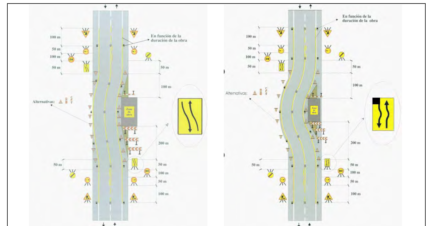
Figura 55. A) Treballs en voravia i part del carril B) Treballs en voravia i part del carril ampliant plataforma
