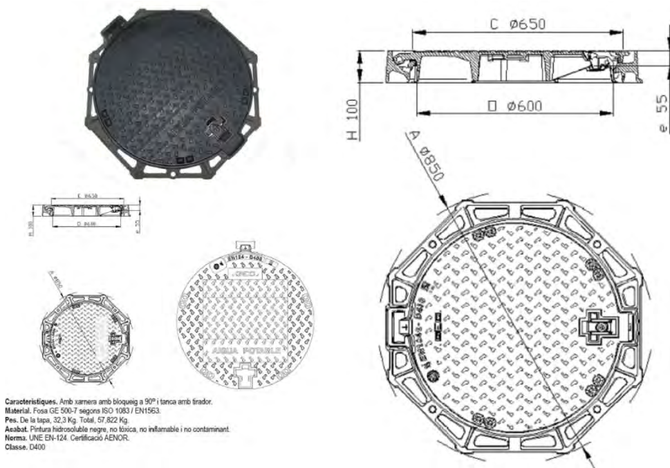
Figura 51. Tapa de registre tipus GEO D400 de EJ o equivalent.
