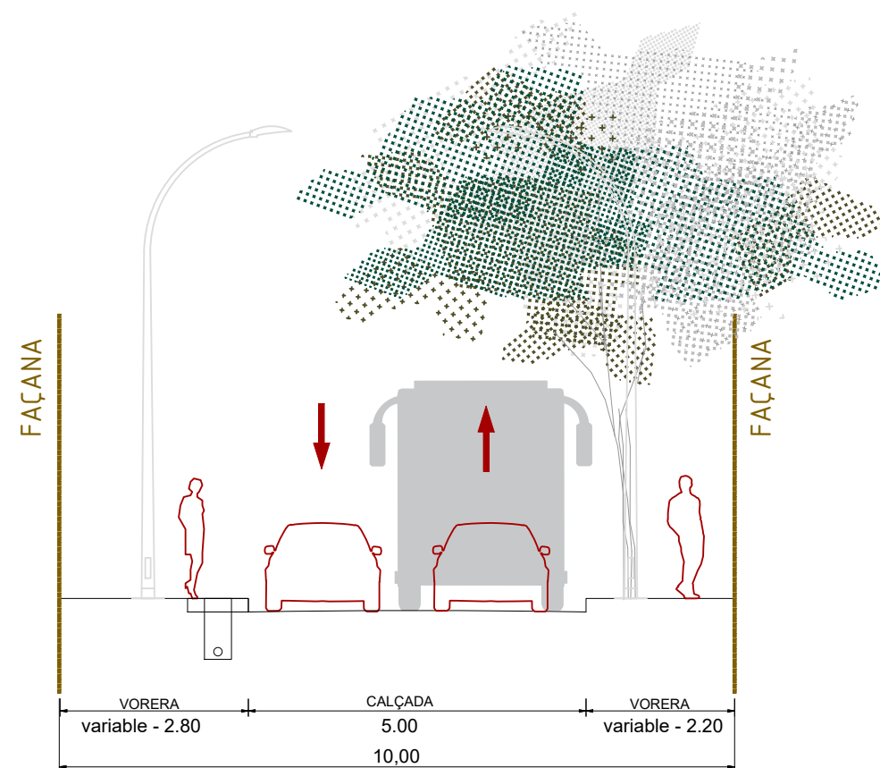
[S3] SECCIÓ TRANSVERSAL PUJADA DE LES PEDRERES
