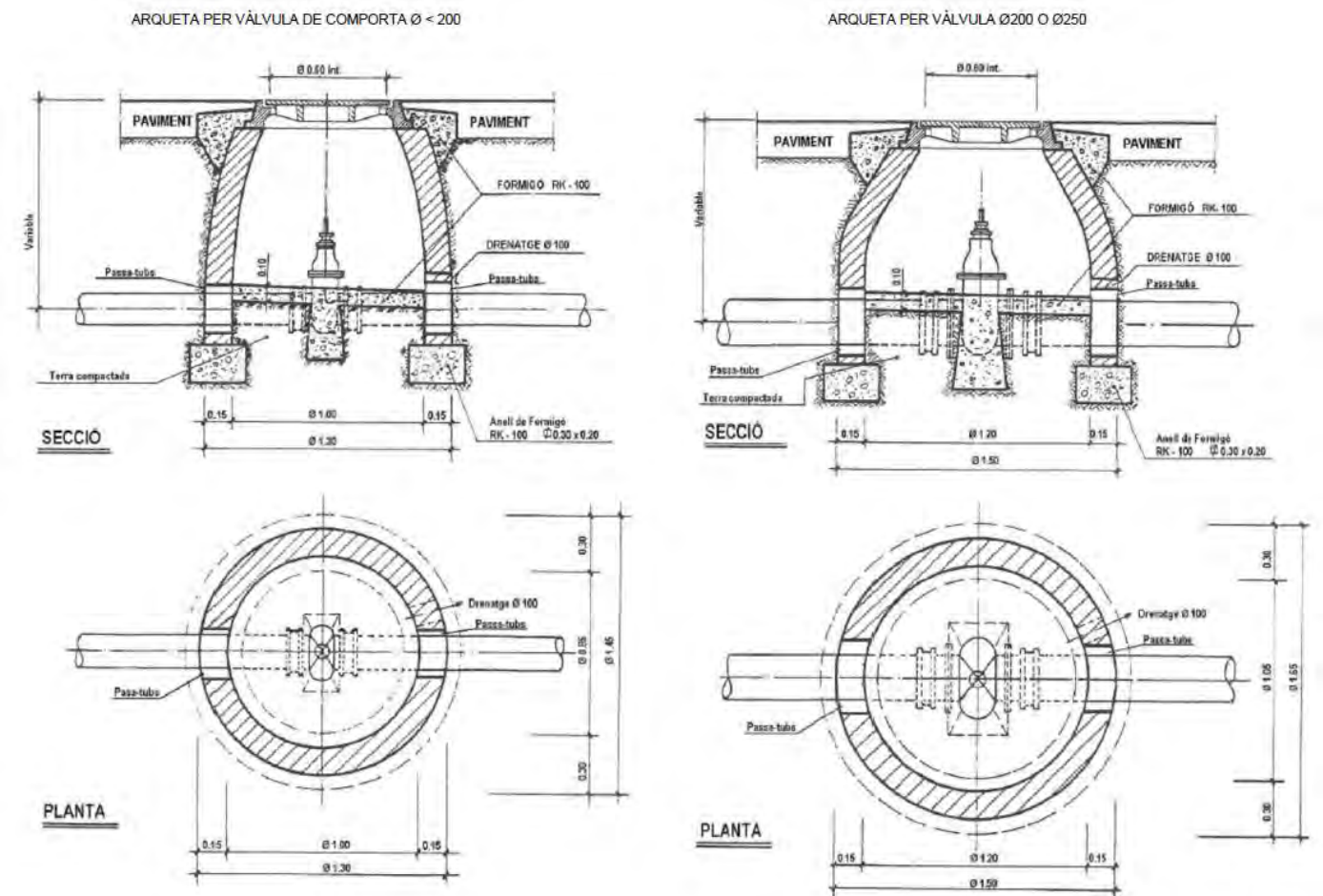
Figura 43. Detall pou de registre per a vàlvula de comporta Ø > o = a 80 mm.
