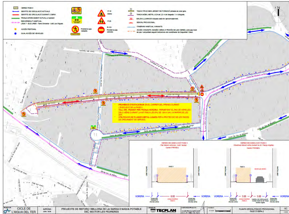
Figura 61. Planta senyalització provisional Fase d'obra 2
