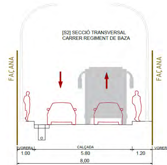
Figura 28. Secció transversal Carrer del Regiment de Baza
