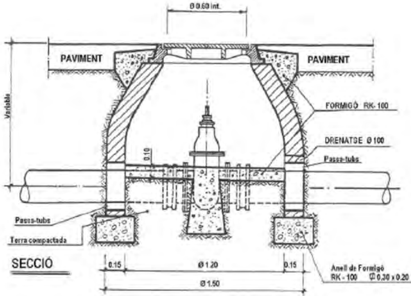
ARQUETA PER VÁLVULA Ø200 O Ø250
