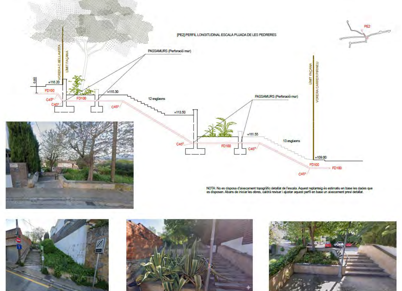
Figura 35. Perfil longitudinal escala Pujada de les Pedreres.
