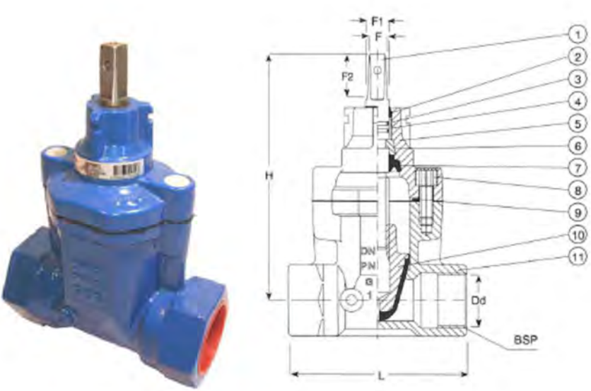
VÀLVULA DE REGISTRE ESCOMESA A PEU DE FAÇANA
