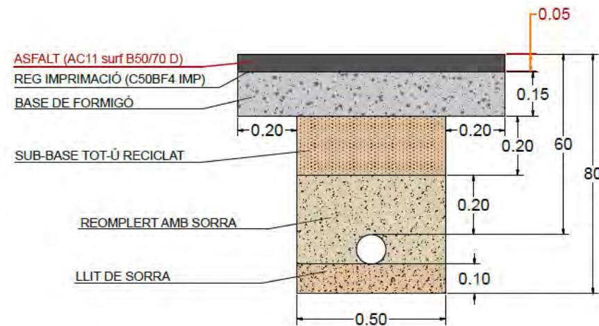
Figura 41. Execució capa rodadura de 5cm de gruix.
