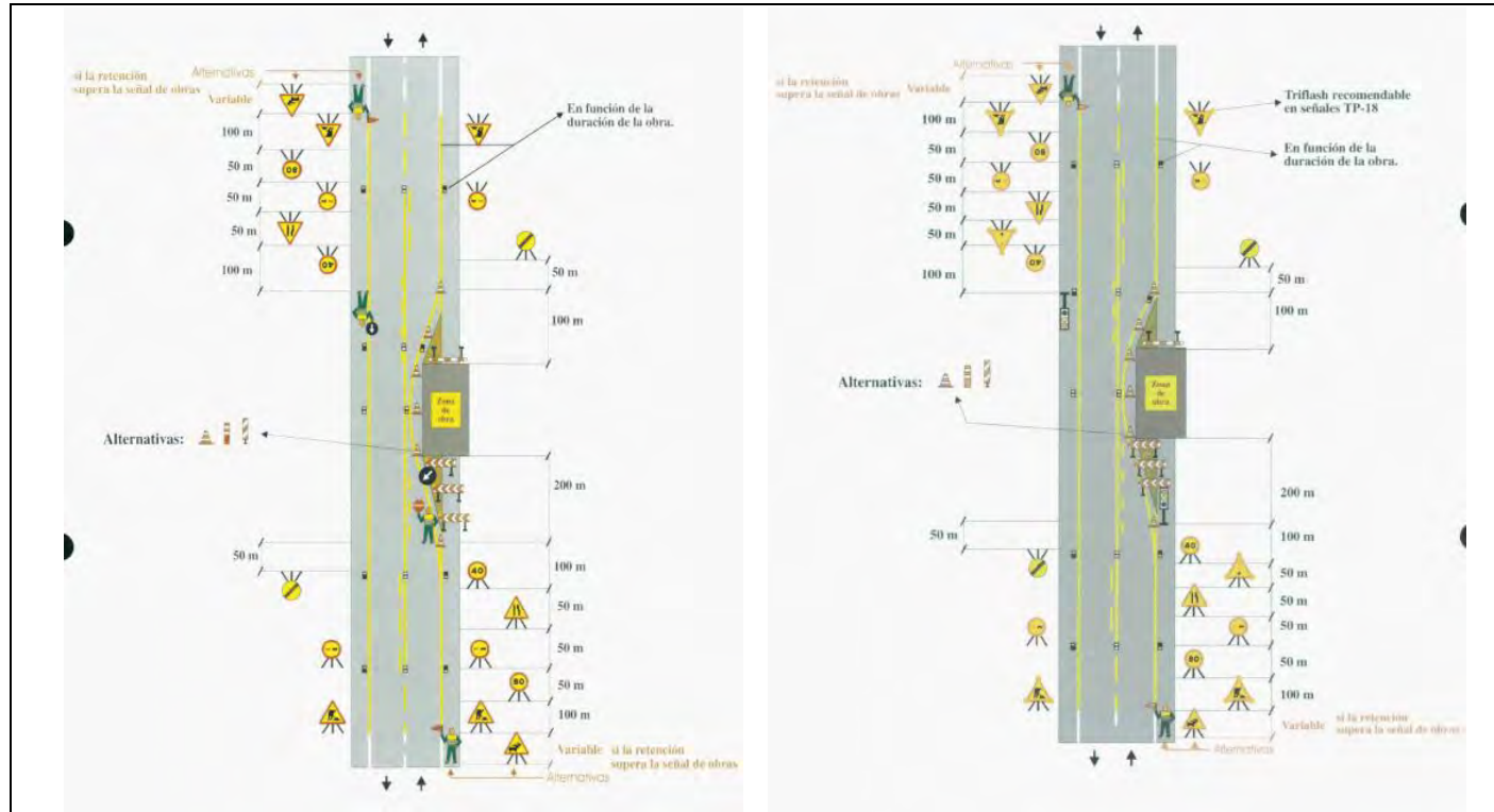
Figura 56. A) Treballs en voravia i carril amb pas alternatiu B) Treballs en voravia i carril pas alternatiu (NIT)
