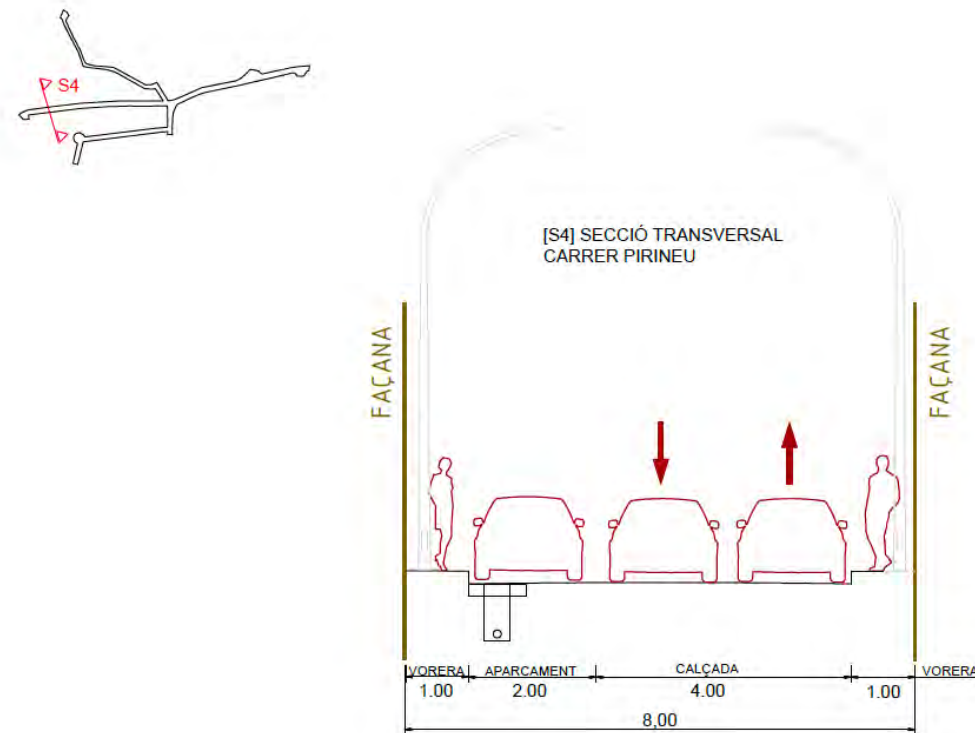
Figura 30. Secció transversal carrer Pirineu.
