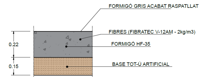
Figura 36. Detall reposició paviment formigó
