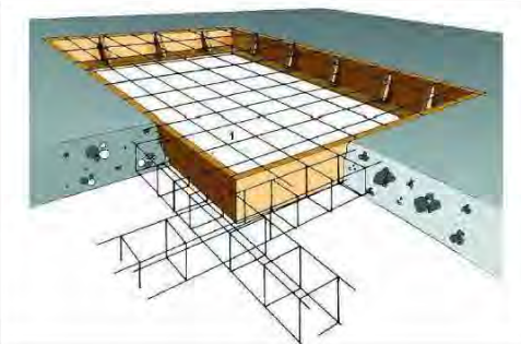
Tapes en forats de forjats Malla electrosoldada en capa superior
