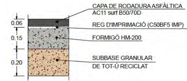
Figura 38. Detall reposició ferm asfàltic.
