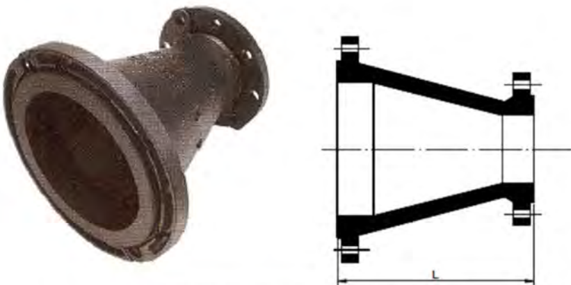
CON DE REDUCCIÓ EMBRIDAT FOSA DÚCTIL
