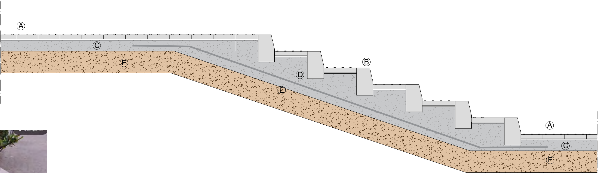
DETALL TIPUS ESCALA AMB PAVIMENT DE PECES DE PEDRA NATURAL
