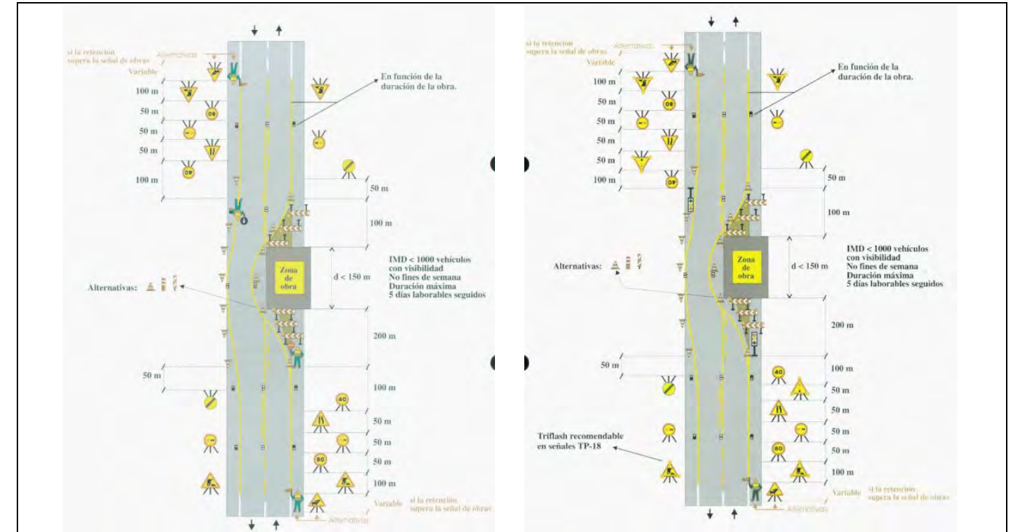
Figura 58. A) Treballs en voravia, un carril i afectació al segon carril (DIA i NIT)
