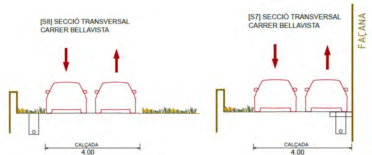
Figura 33. Seccions transversals carrer Bellavista.
