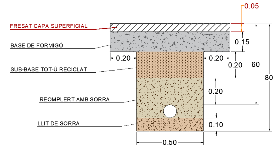
Figura 40. Execució fresat superficial de 5cm de gruix de la base de formigó.
