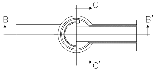
POU DE REGISTRE TIPUS D PER A TUB CIRCULAR <80
