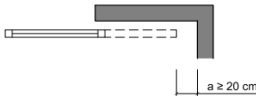
Figura 2.1 Folgança per evitar atrapaments
