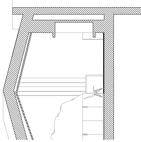
SECCIÓ C-C'
