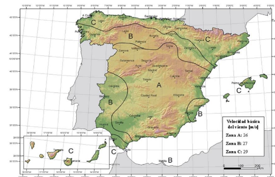
Figura AN.1 - Mapa de isotacas de la velocidad básica fundamental del viento V_{b,0}
