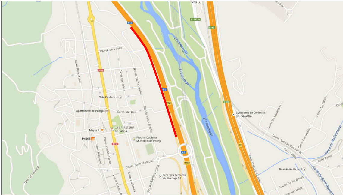
Imatge 25: Ubicació de l'apantallament acústic proposat a Pallejà.
