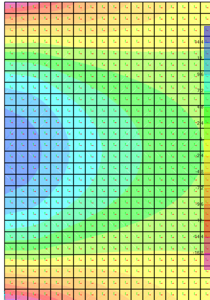
Momento flector debido a barrera New Jersey
