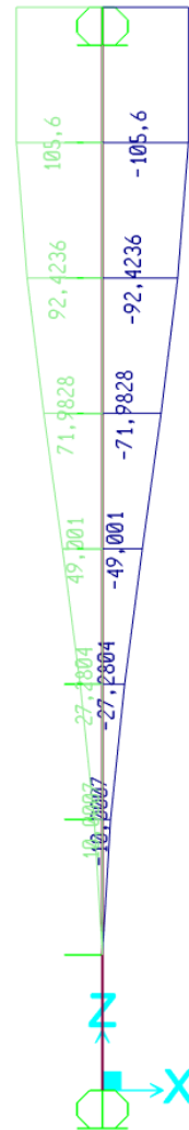
Esfuerzo flector resultante en ELU
