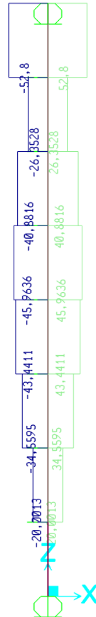
Esfuerzo cortante resultante en ELU
