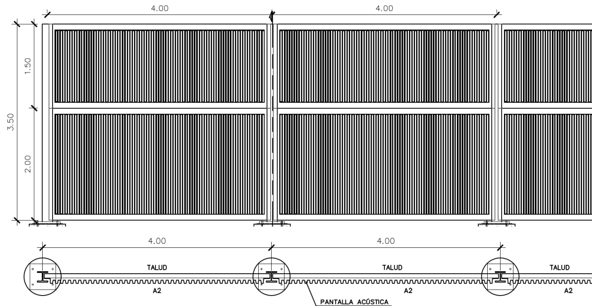
Alzado y planta del apantallamiento acústico propuesto en el presente proyecto
