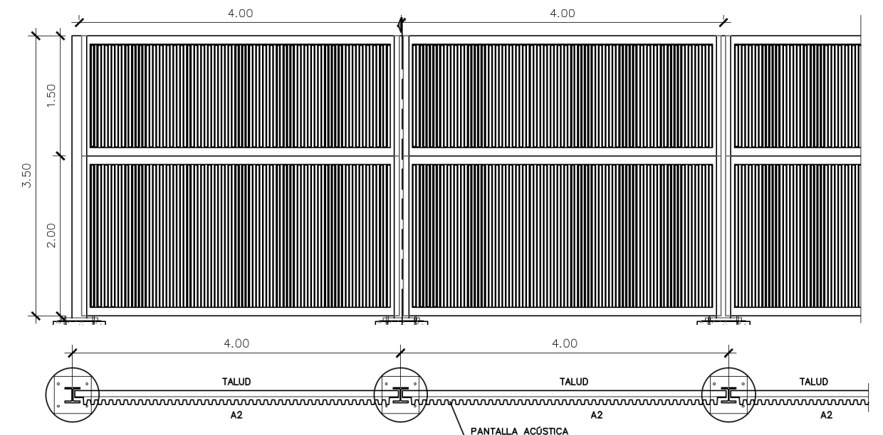
Alzado y planta del apantallamiento acústico propuesto en el presente proyecto
