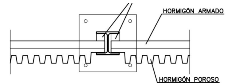
Detalle del apantallamiento acústico propuesto en el presente proyecto
