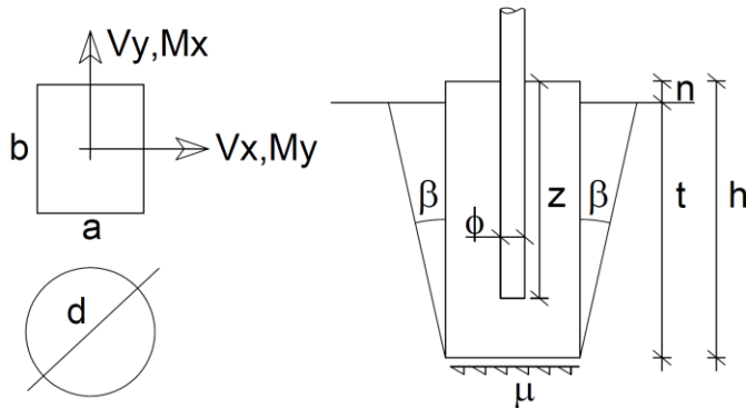
Croquis de las variables de cálculo
