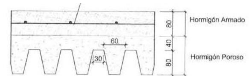
Croquis ilustrativo de la pantalla considerada
