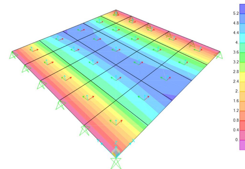
Momentos flectores de diseño
