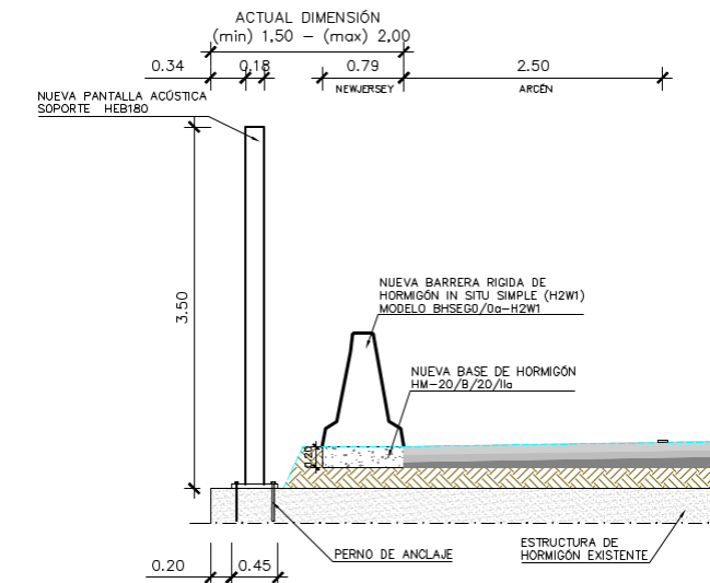
SECCIÓN TIPO (EN ESTRUCTURA) (SECCIÓN TIPO B)
