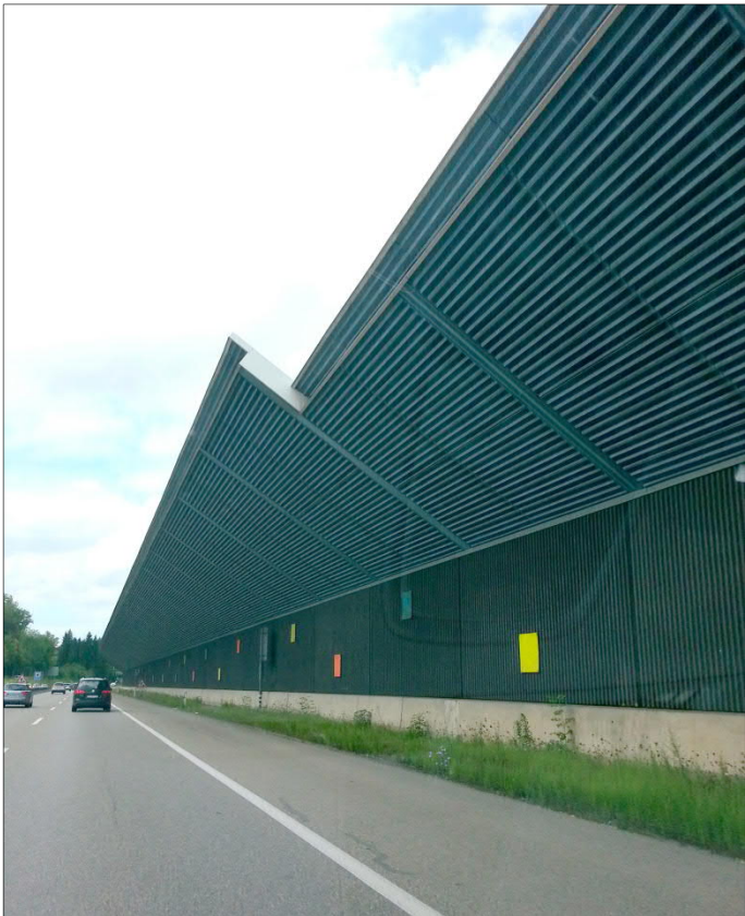
Imatge 24: Exemple d'apantallament acústic amb voladís.
