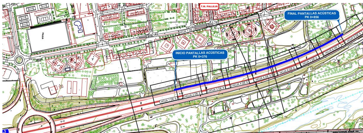
Planta de conjunto del apantallamiento propuesto, de 480 metros de longitud.
