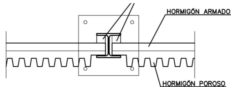
Detalle del apantallamiento acústico propuesto en el presente proyecto
