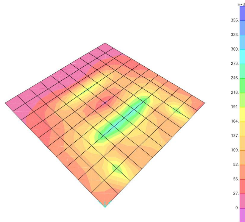
Criterio de von Mises en cimentación 2
