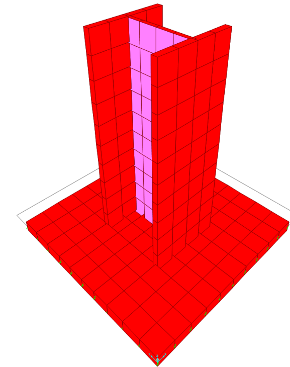
Geometría de la simulación de la placa de anclaje
