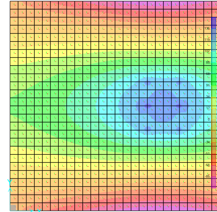
Momento flector debido a cargas de tráfico
