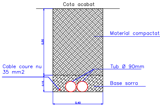
RASA TIPUS (E: 1/10)
