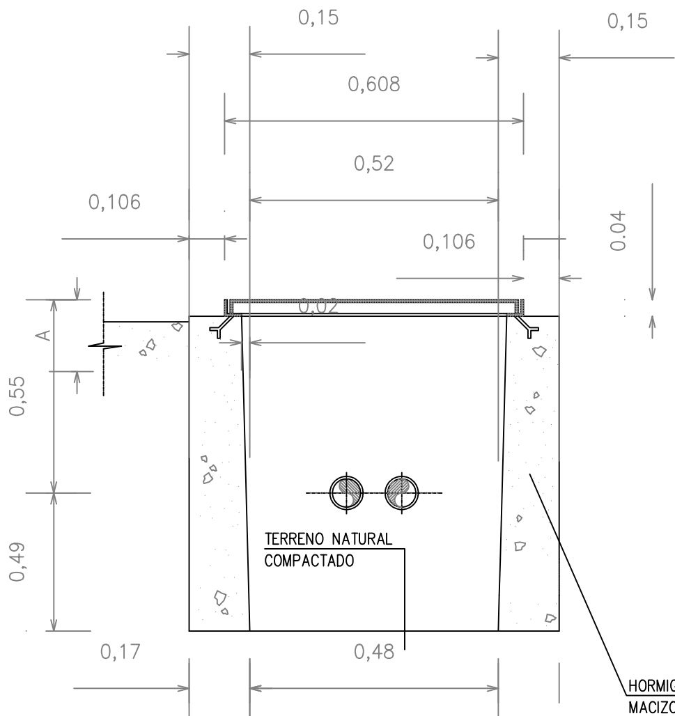
SECCION A-A
