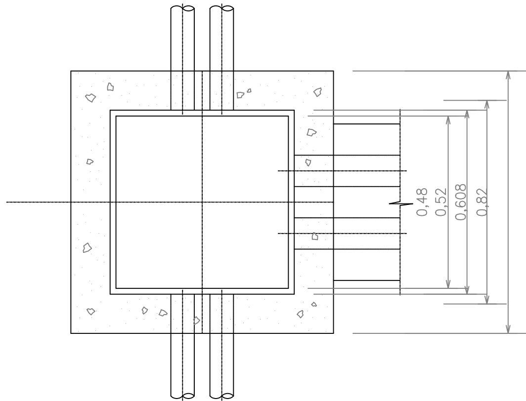
PLANTA SECCION
