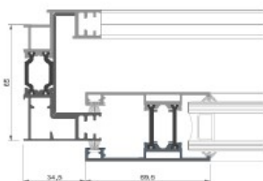
MARCO / HOJA LATERAL
