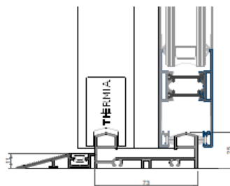
MARCO INFERIOR SOBREPUESTO PMR
