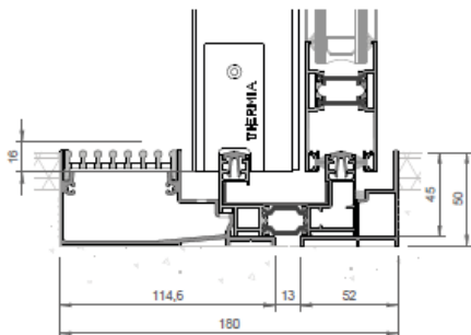
MARCO INFERIOR EMPOTRADO CON RECOCAGUA
