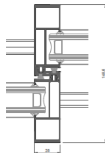
CENTRAL REDUCIDO REFORZADO
