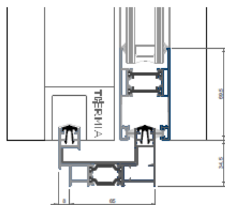
MARCO INFERIOR SOBREPUESTO
