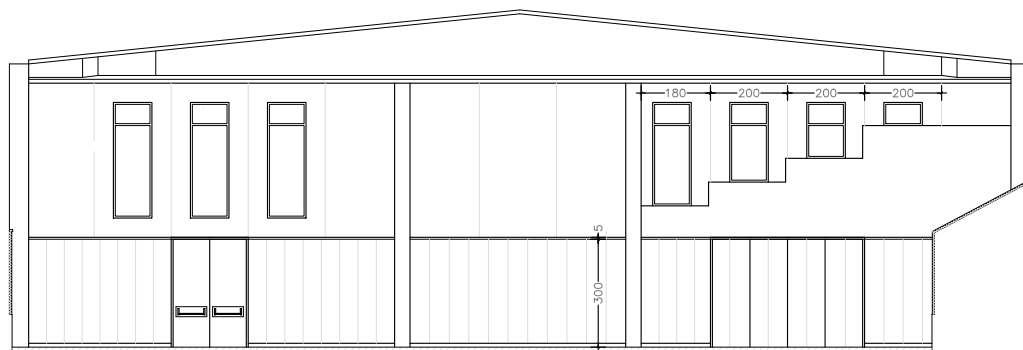
ALÇAT INTERIOR 1 (PASSEIG) ESC. 1/200
