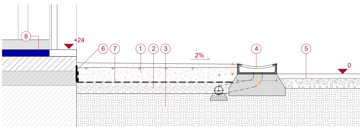
DET. REIXA INTEGRADA EN CANAL EN RECOLLIDA D'AIGÜES E: 1/20
