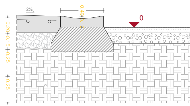
DET. CANAL DE RECOLLIDA D'AIGÜES E: 1/20
