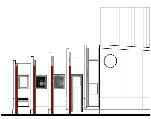
ALÇAT 3. E: 1/200
