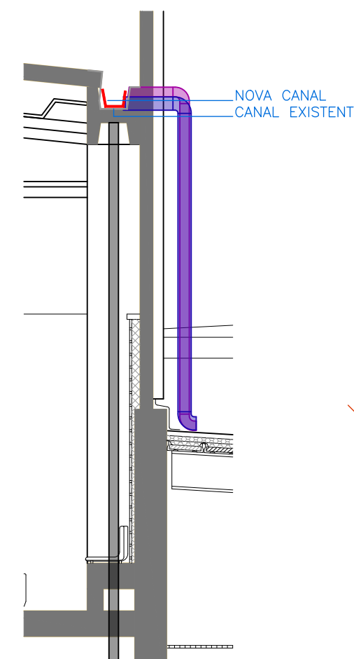
DET. NOVA CANAL
