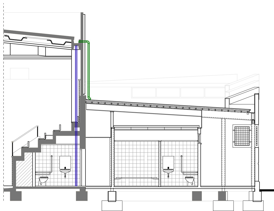
SECCIÓ S1. E: 1/50
