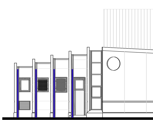
ALÇAT 3. E: 1/200
