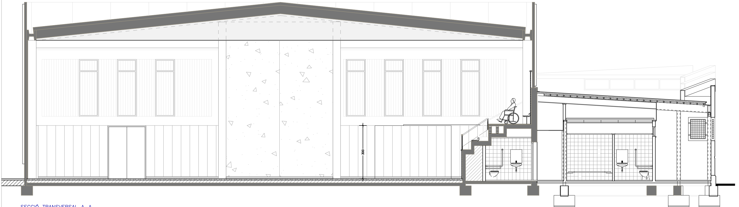
SECCIÓ TRANSVERSAL A-A ESC. 1/100
