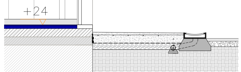
SECCIÓ 1. E: 1/40
