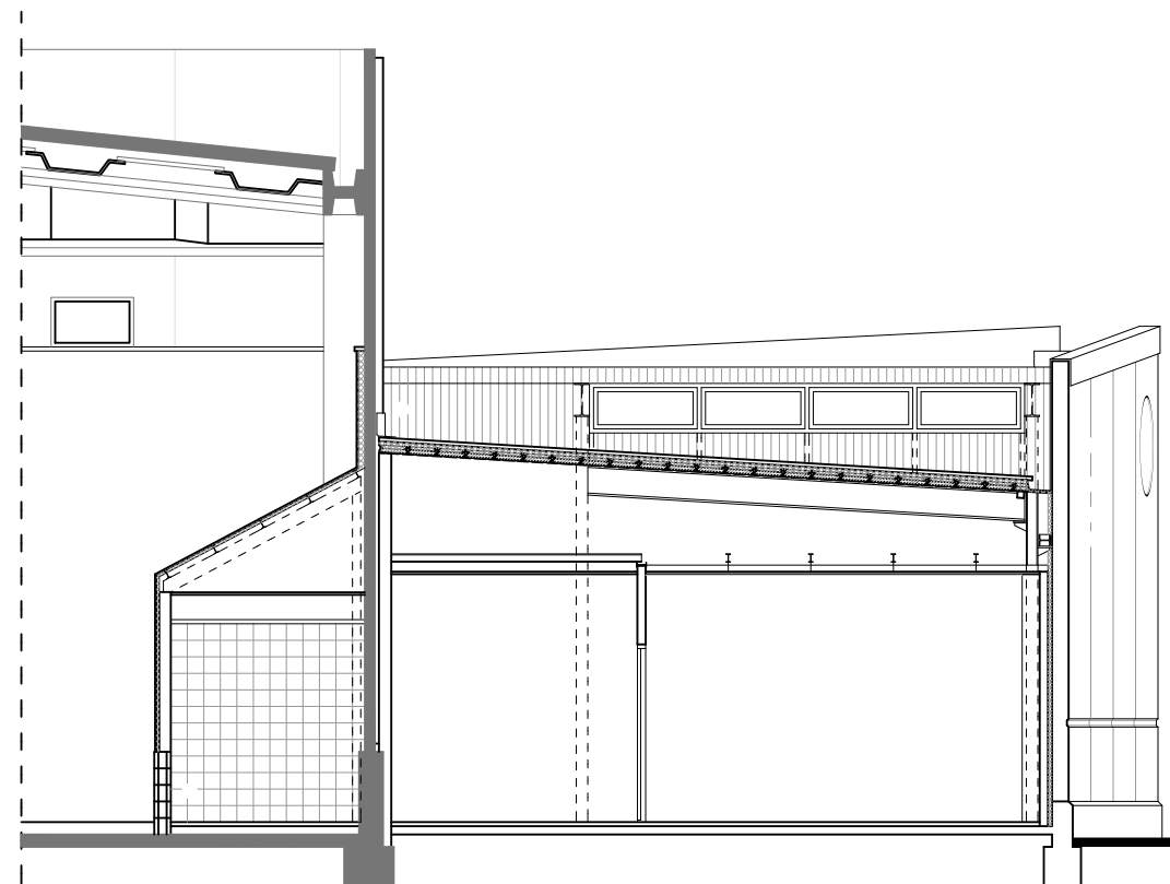
SECCIÓ TRANSVERSAL C-C ESC. 1/100
