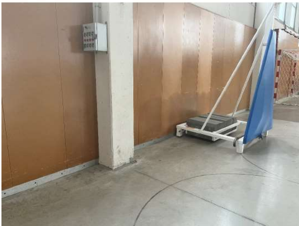
Imatge 6: humitats en revestiments i perímetre paviment
