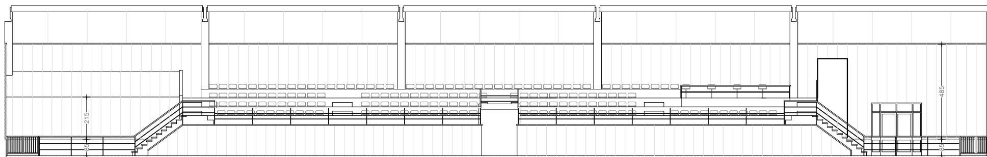
ALÇAT INTERIOR 2 (CARRETERA) ESC. 1/200
