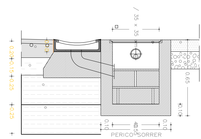
DET. PERICÓ SORRER E: 1/20
