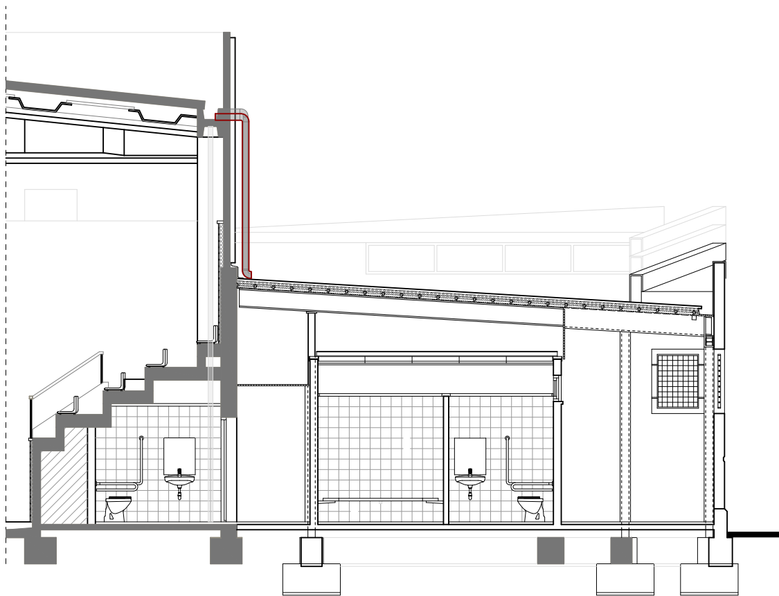
SECCIÓ S1. E: 1/50
