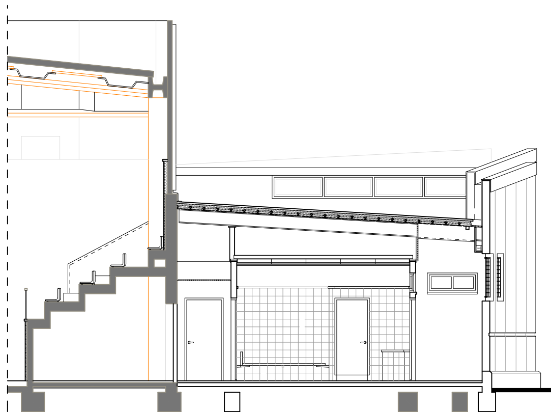
SECCIÓ TRANSVERSAL B-B ESC. 1/100
