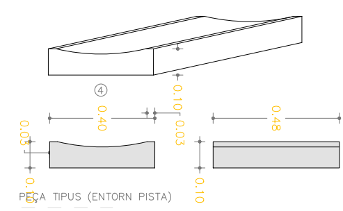
DET. PEÇA TIPUS (ENTORN PISTA) E: 1/20
