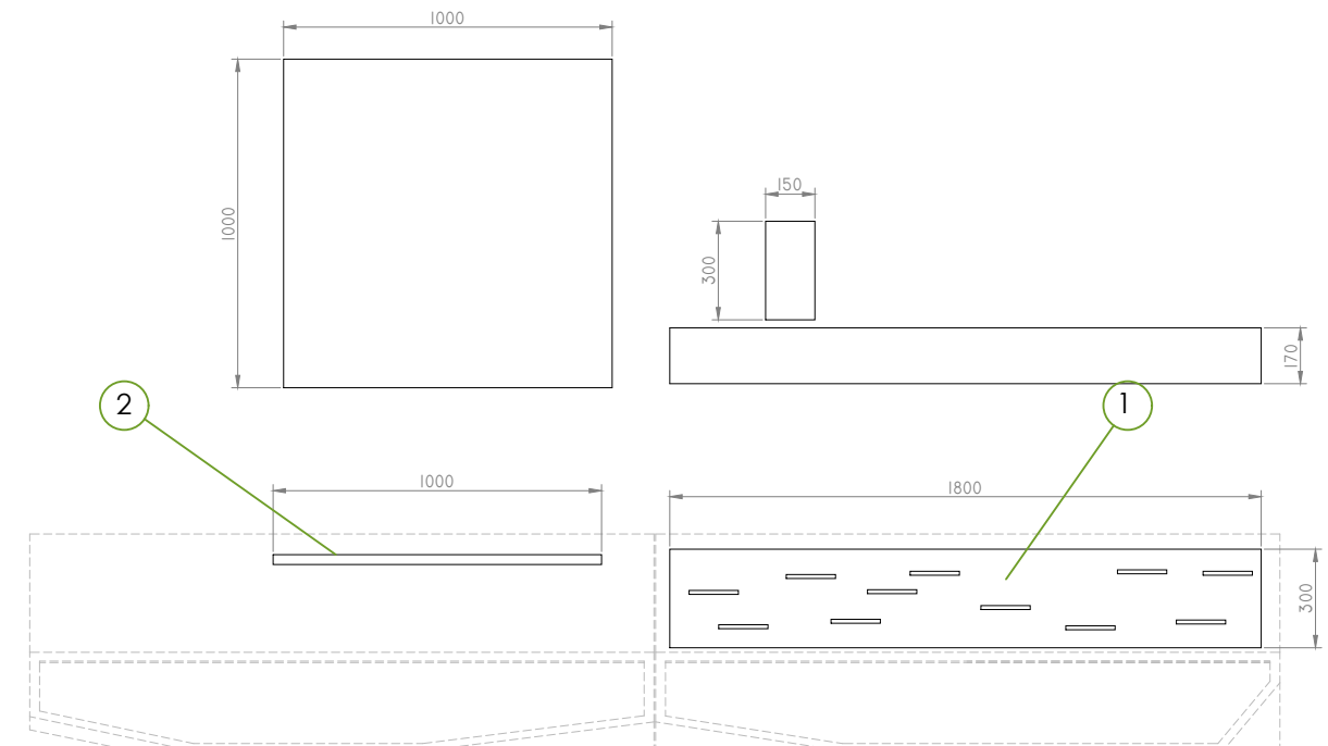
Planta Mobles 7 i 8
