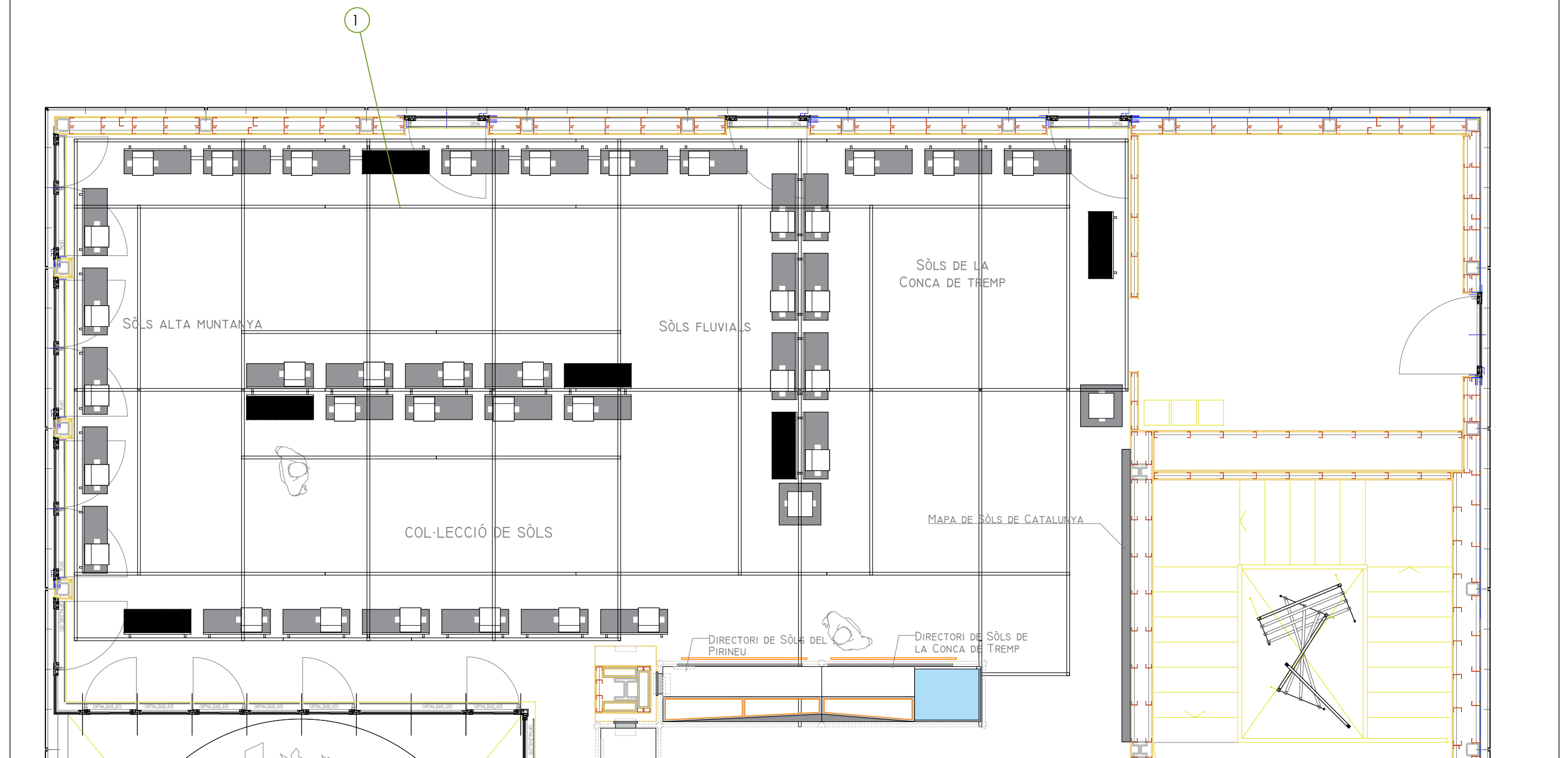
PLANTA COL·LECCIÓ DE SÒLS
