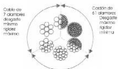
Fig. 11 Ejemplos de cables de 6 cordeles.
