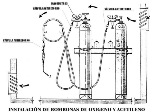
INSTALACIÓN DE BOMBONAS DE OXÍGENO Y ACETILENO
