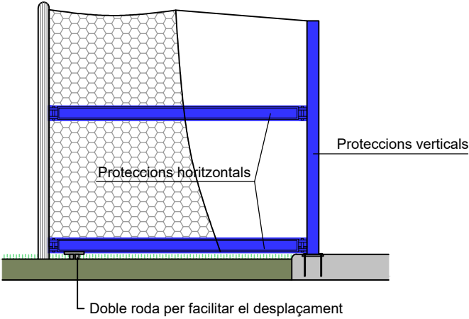
INSTAL·LACIÓ PORTERIES F7
