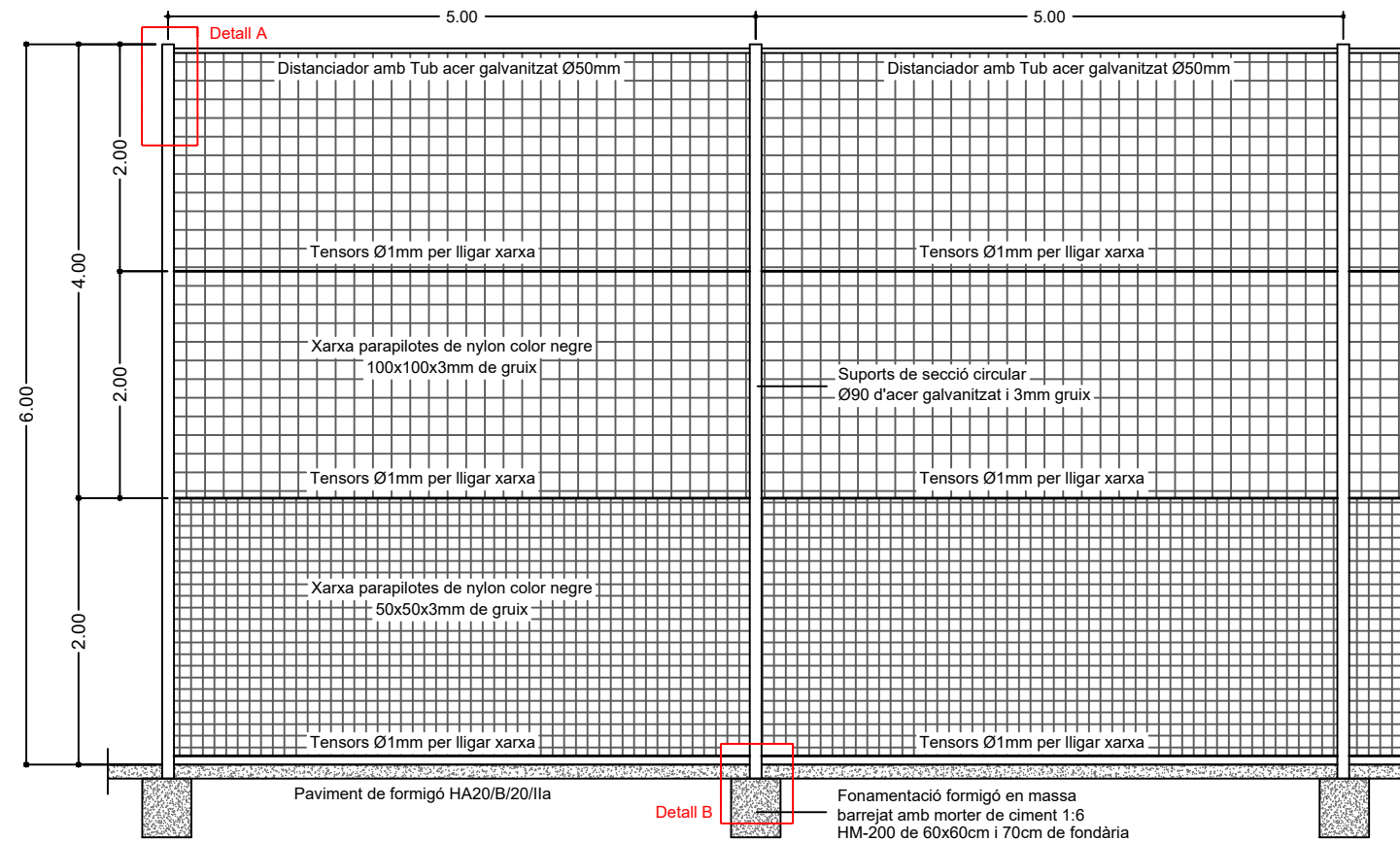
DETALL XARXA PARAPILOTES
