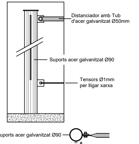
Detall arriostaments i fixacions
