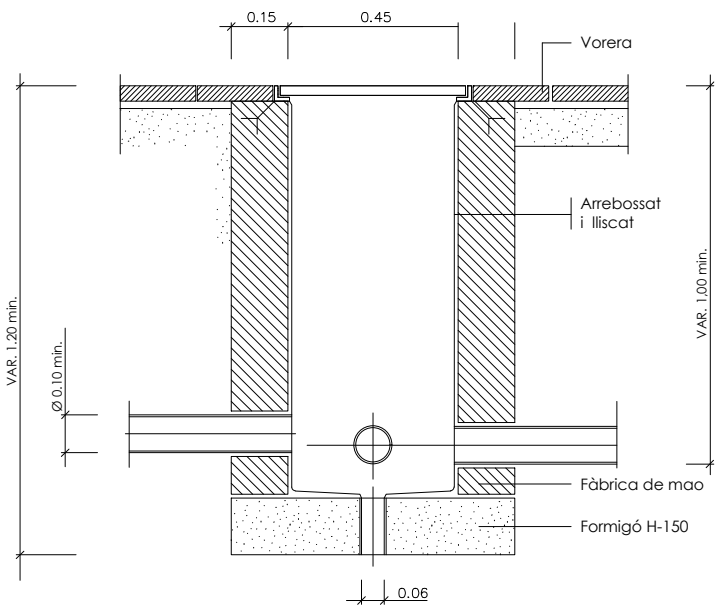
ARQUETA TIPUS
