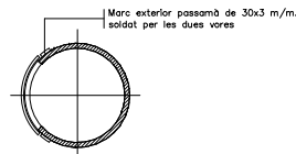
DETALL MARC DE REFORÇ EXTERIOR
