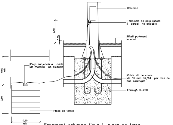
Fonament columna tipus i placa de terra
