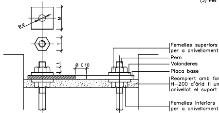
Detall ancoratges de les columnes i bàculs
