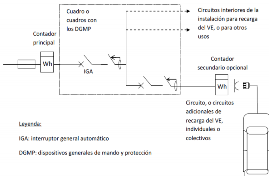
Imatge 8.1. Esquema 4b: instal·lació amb circuit addicional
