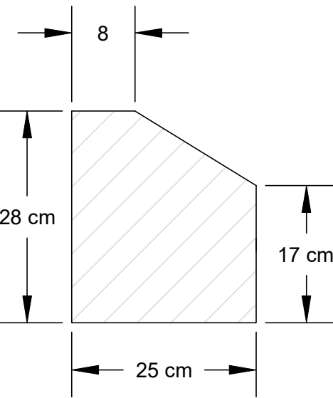
VORADA DE FORMIGO PREFABRICAT REMONTABLE (L=50cm)
