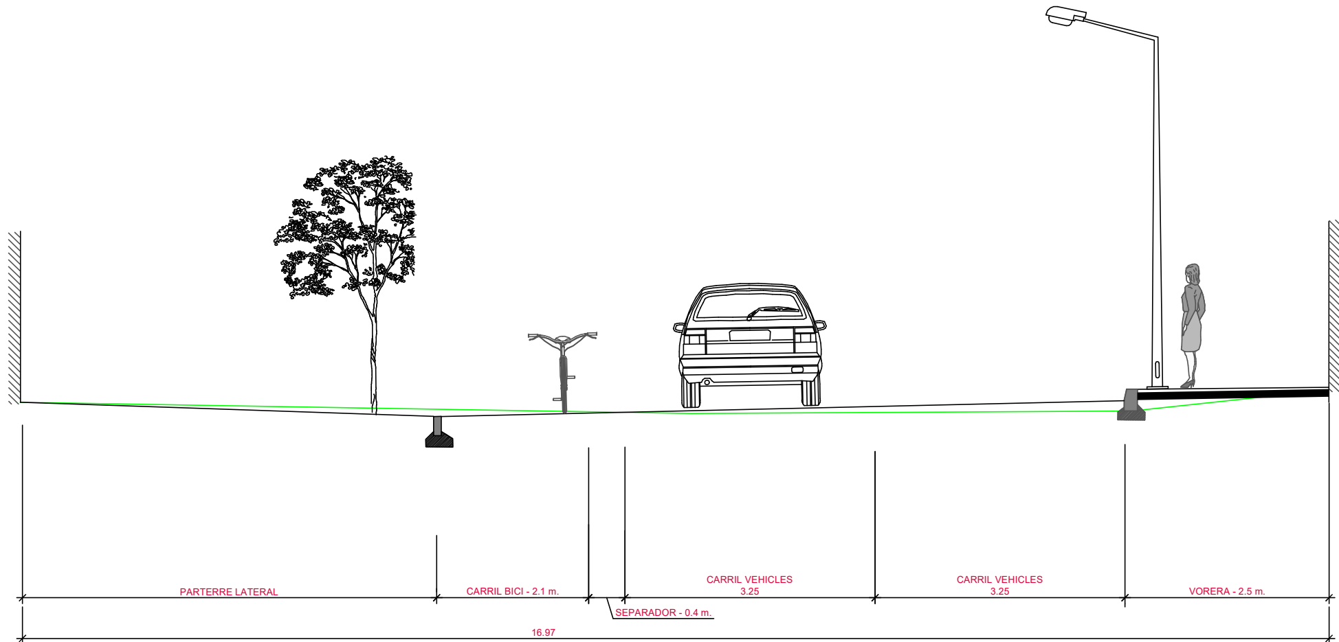
SECCIÓ E-E' TRAM FINAL - SECCIÓ PARTERRE LATERAL
