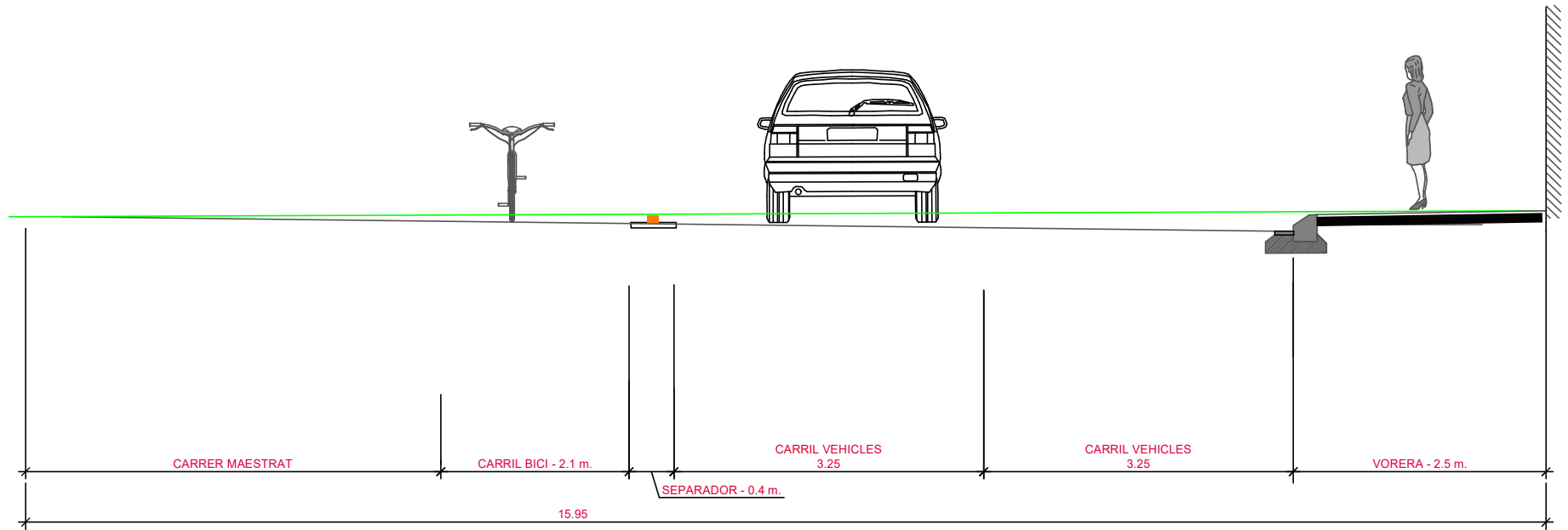
SECCIÓ B-B' TRAM INICIAL - TRANSICIÓ CARRER MAESTRAT
