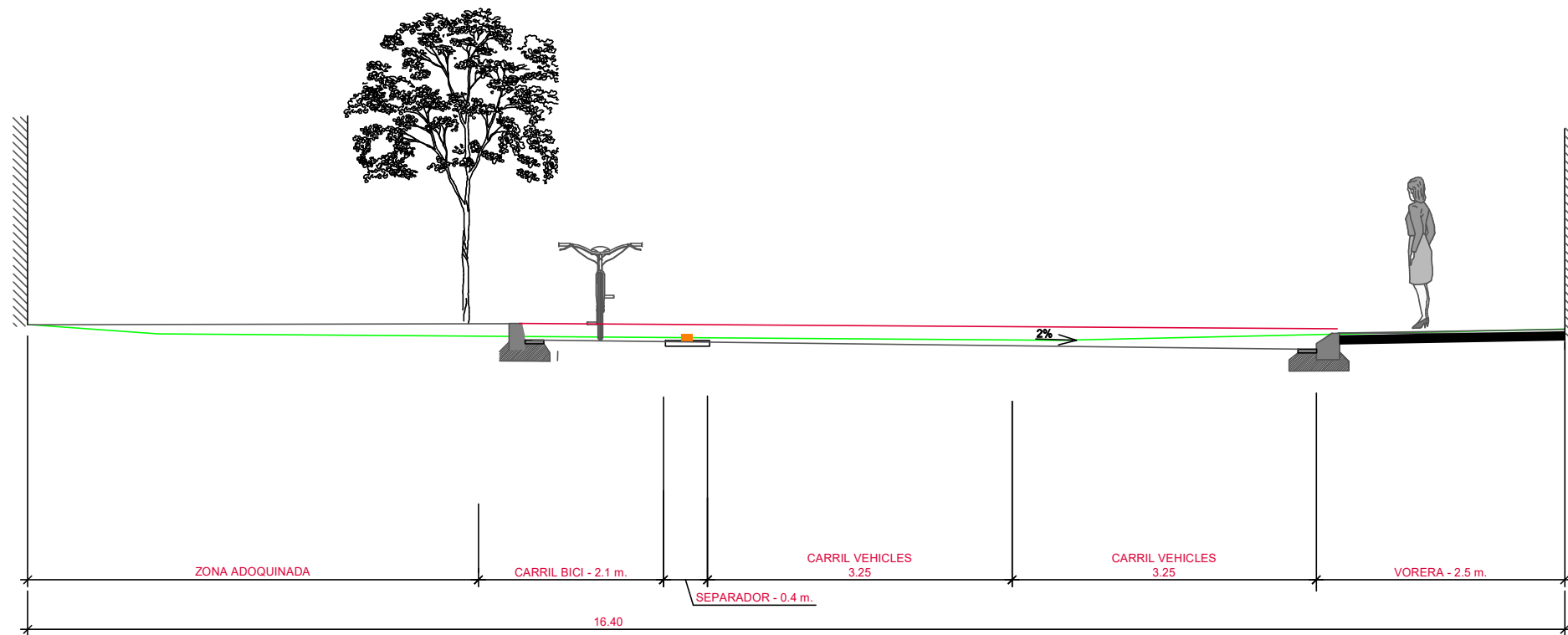
SECCIÓ D-D' TRAM INTERMIG - ZONA ADOQUINADA LATERAL
