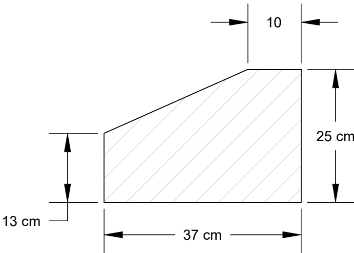
VORADA DE FORMIGO (40) PREFABRICAT REMONTABLE (L=50cm). GUAL VEHICLES 40
