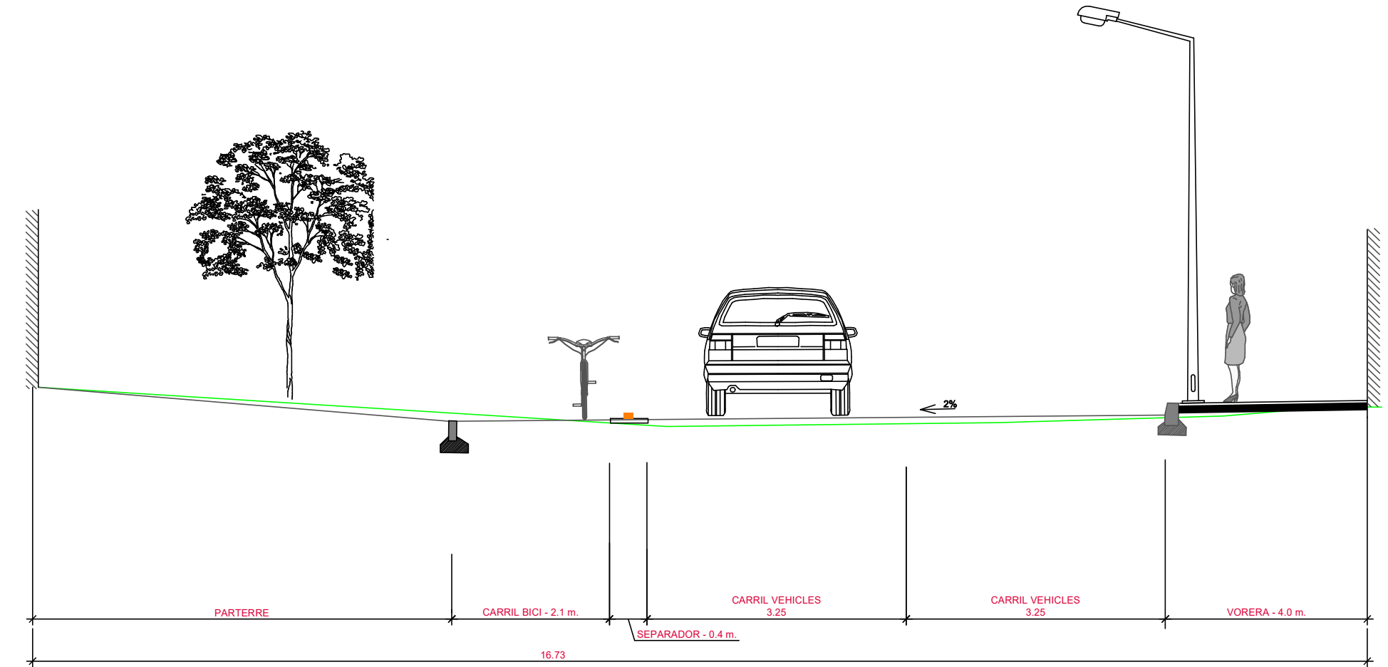
SECCIÓ G-G' TRAM FINAL - PARTERRES LATERALS
