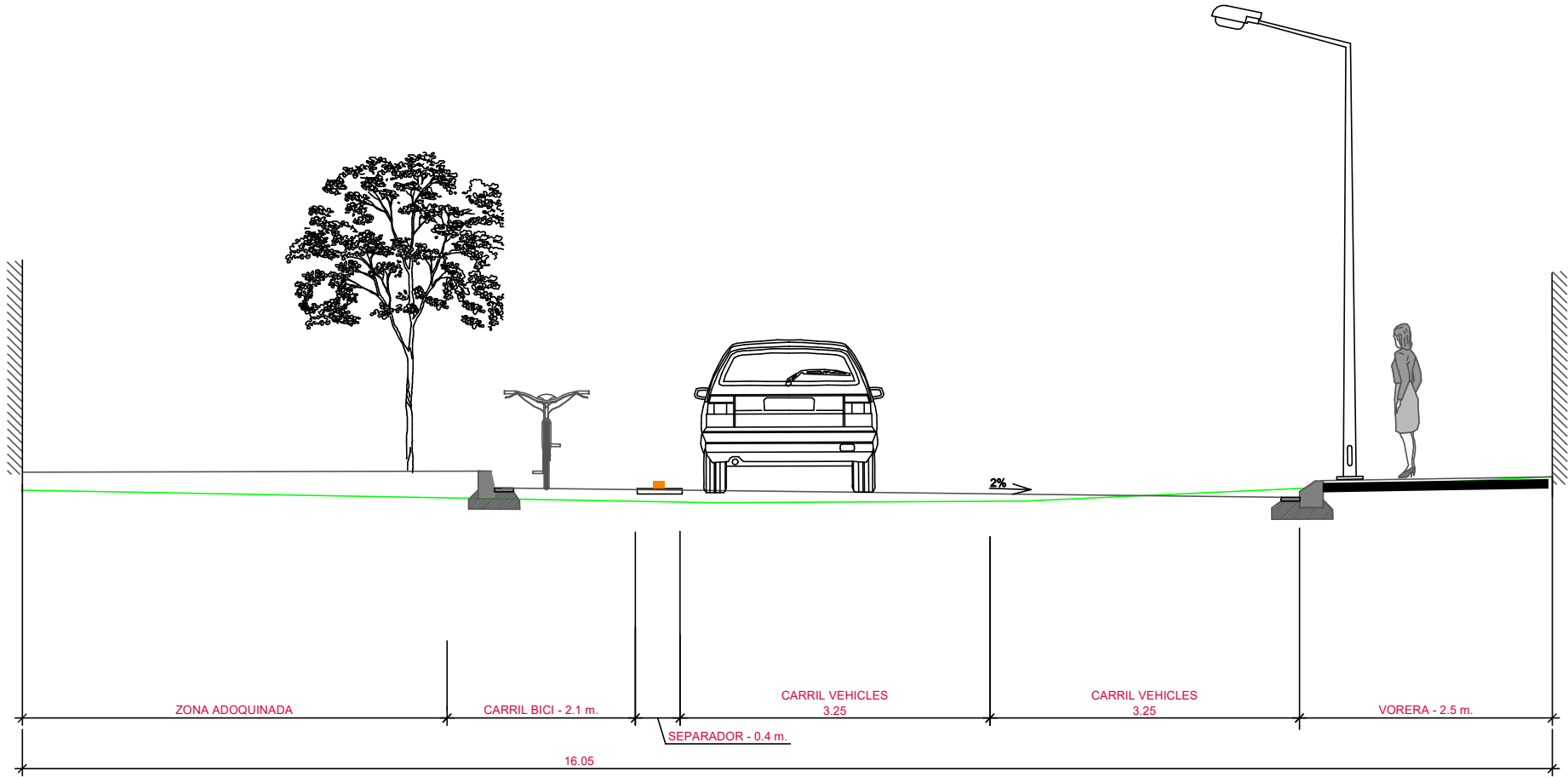
SECCIÓ C-C' TRAM INTERMIG - ZONA ADOQUINADA LATERAL
