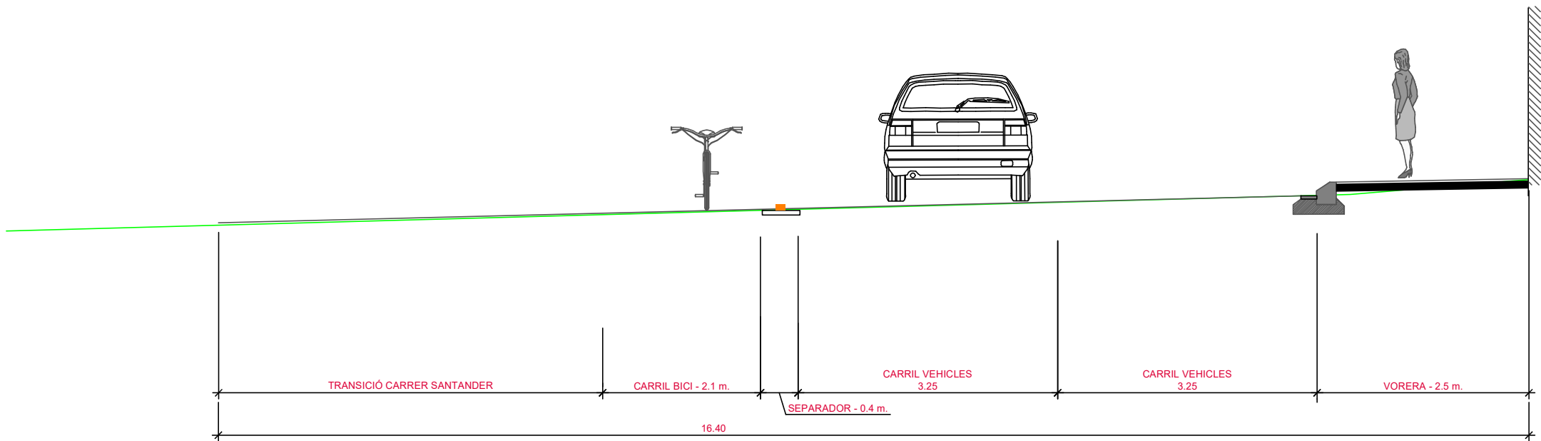
SECCIÓ E-E' TRAM INTERMIG - TRANSICIÓ CARRER SANTANDER
