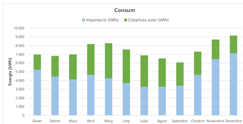
Fig. 7.2. Consum mensual estimat.
