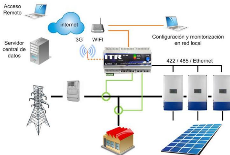
Fig. 7.1. Connexionat i funcionament del sistema de monitoratge.
