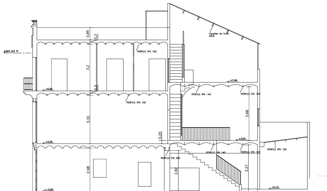
SECCIÓ LONGITUDINAL
