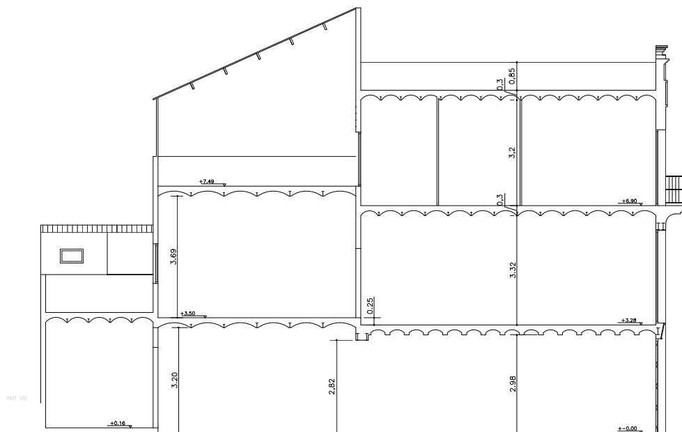
SECCIÓ LONGITUDINAL
