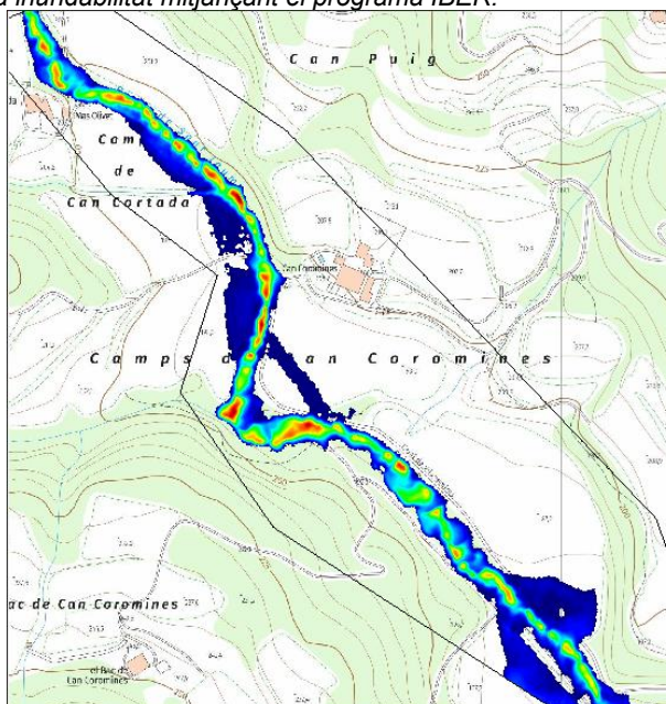
Figura 1. Situació de la carretera respecte la inundabilitat associada a la riera de Sant Jaume.
