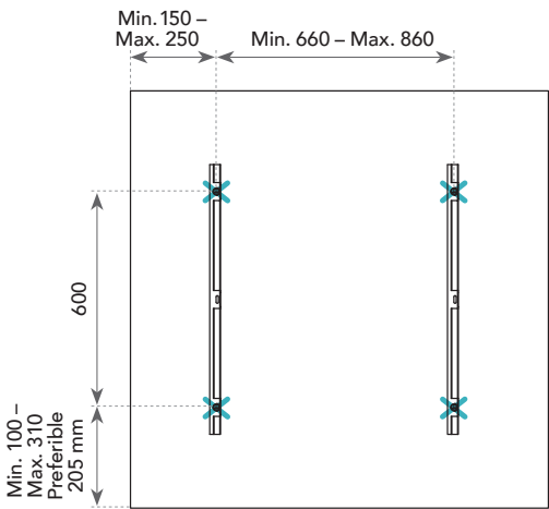
PLANO DE LA ISLA 1160 x 1160 / 4 fijaciones en espiral por isla
