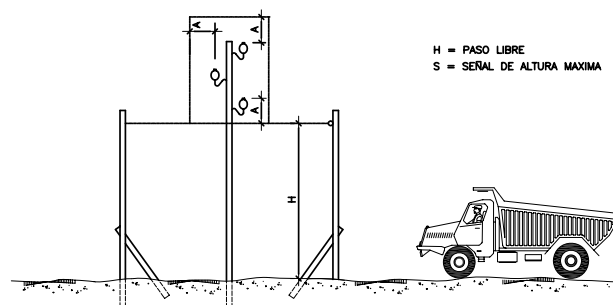
ALZADO
