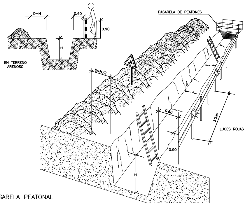
PROTECCION EN ZANJAS
