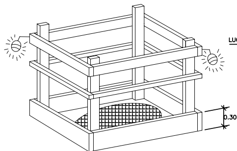
PROTECCION EN HUECOS Y ABERTURAS
