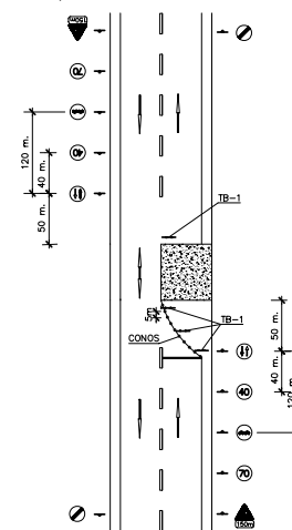
OBRAS QUE OCUPAN UNA VIA COMPLETAS
