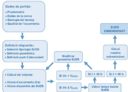
Figura 4. Passos a seguir pel dimensionament dels SUDS.
