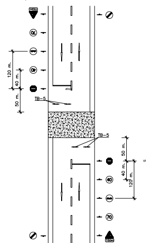
OBRAS QUE OCUPAN DOS VIAS COMPLETAS
