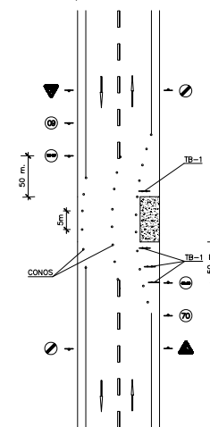
OBRAS QUE OCUPAN UN ARCE
