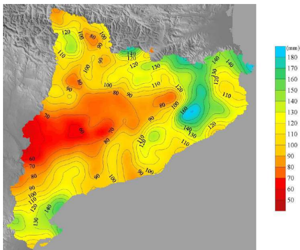
Figura 1. Precipitació màxima en un dia (en mm).
