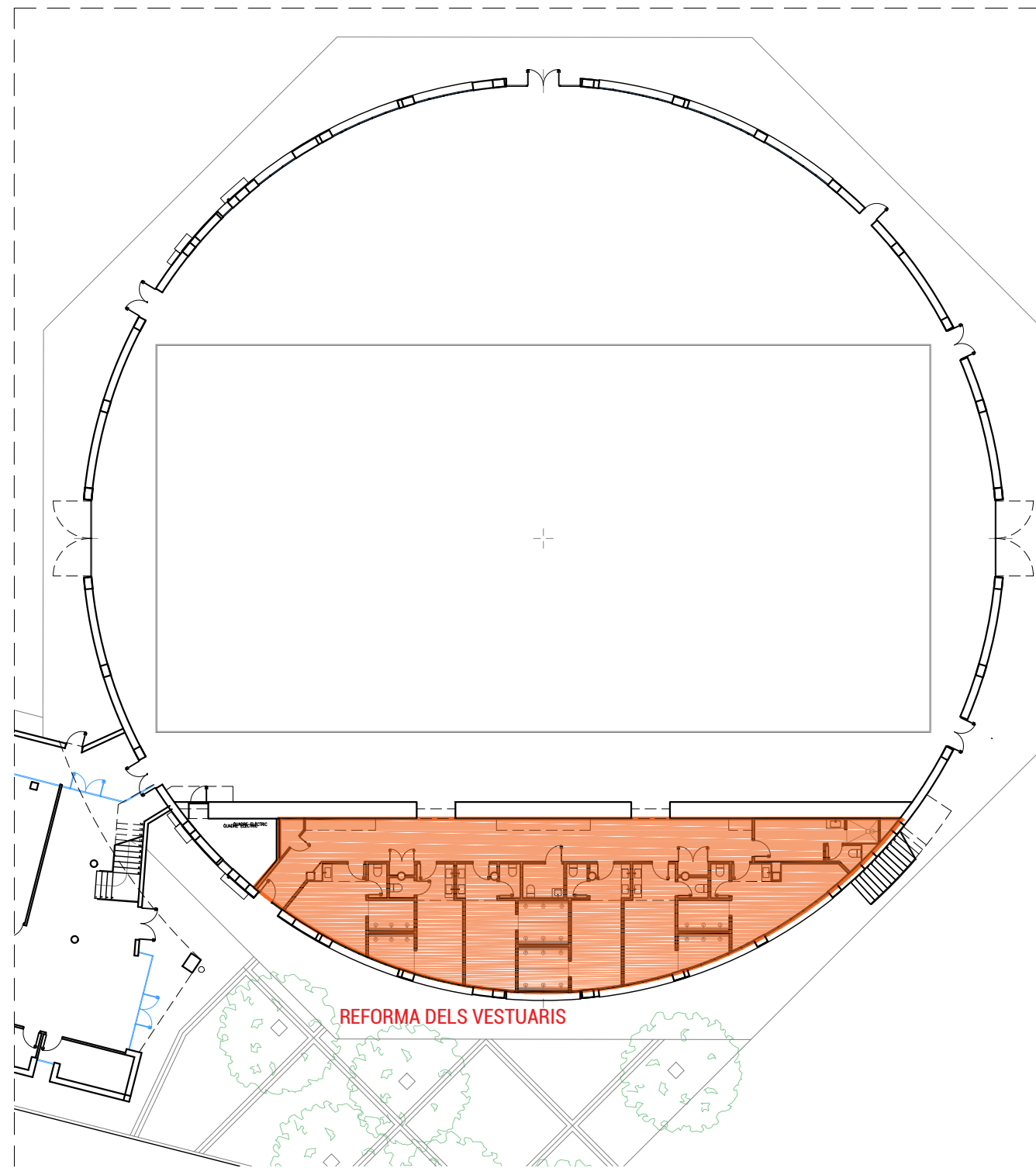
PLANTA BAIXA
