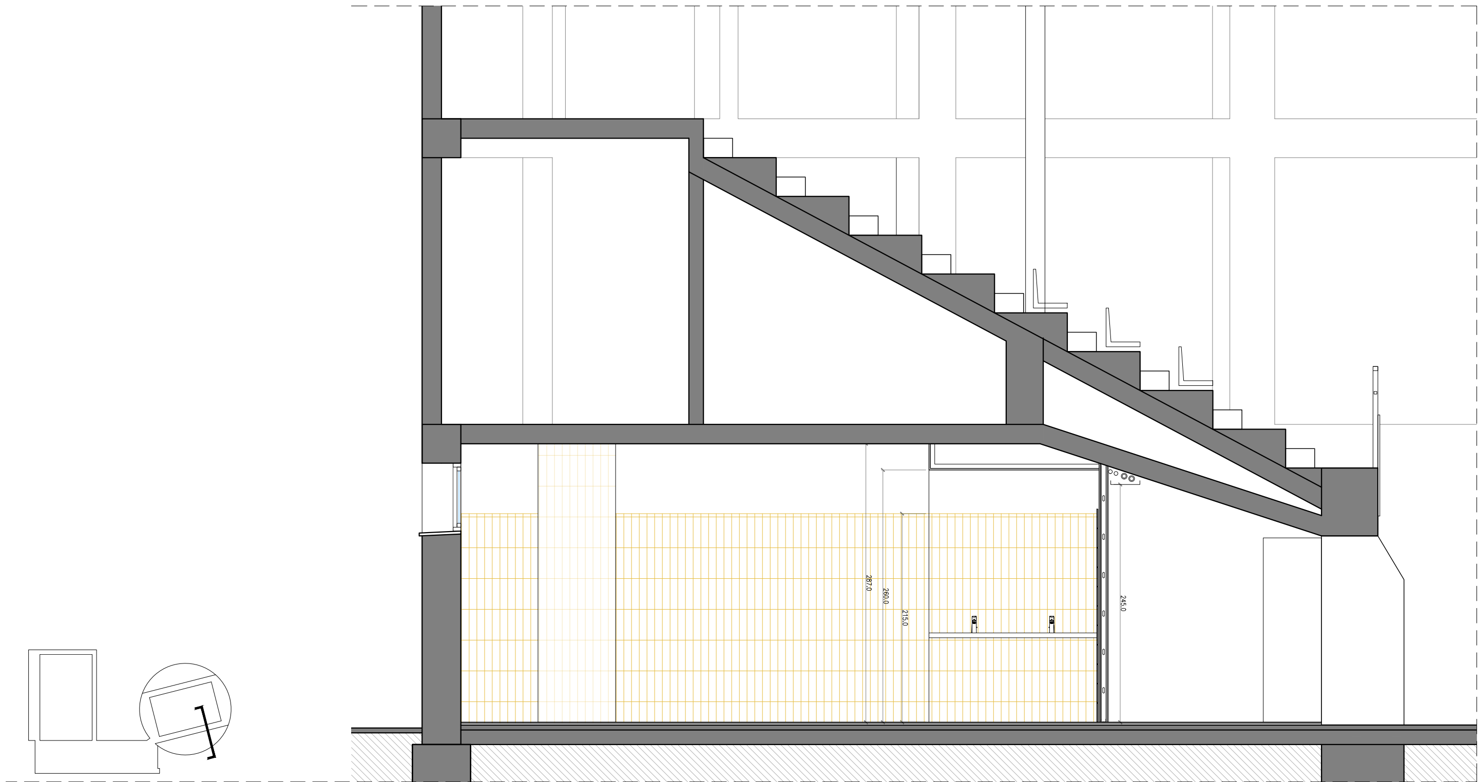
SECCIÓ TRANSVERSAL PER LES GRADES
