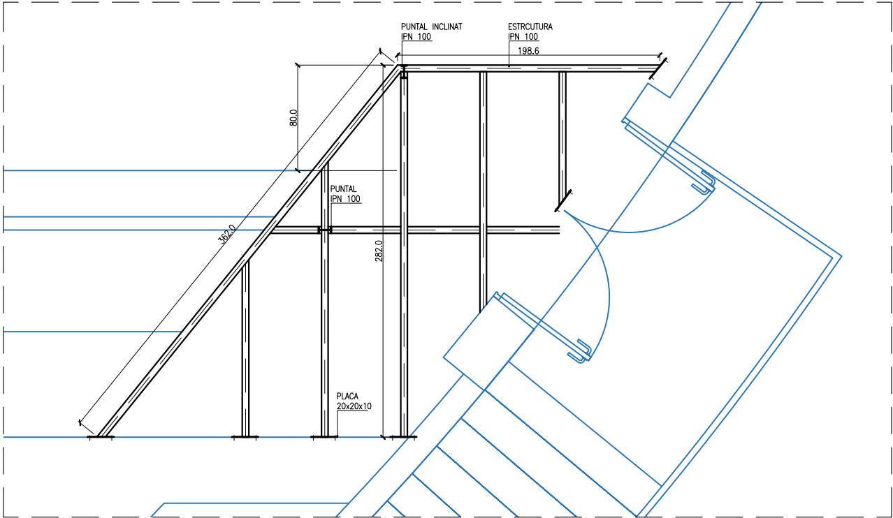
ESTRUCTURA 1:40
