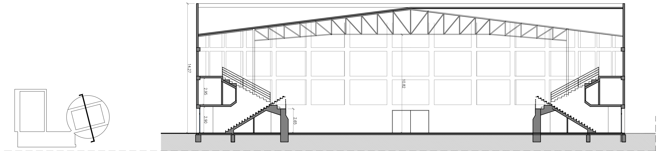
SECCIÓ TRANSVERSAL PER L'ACCÉS
