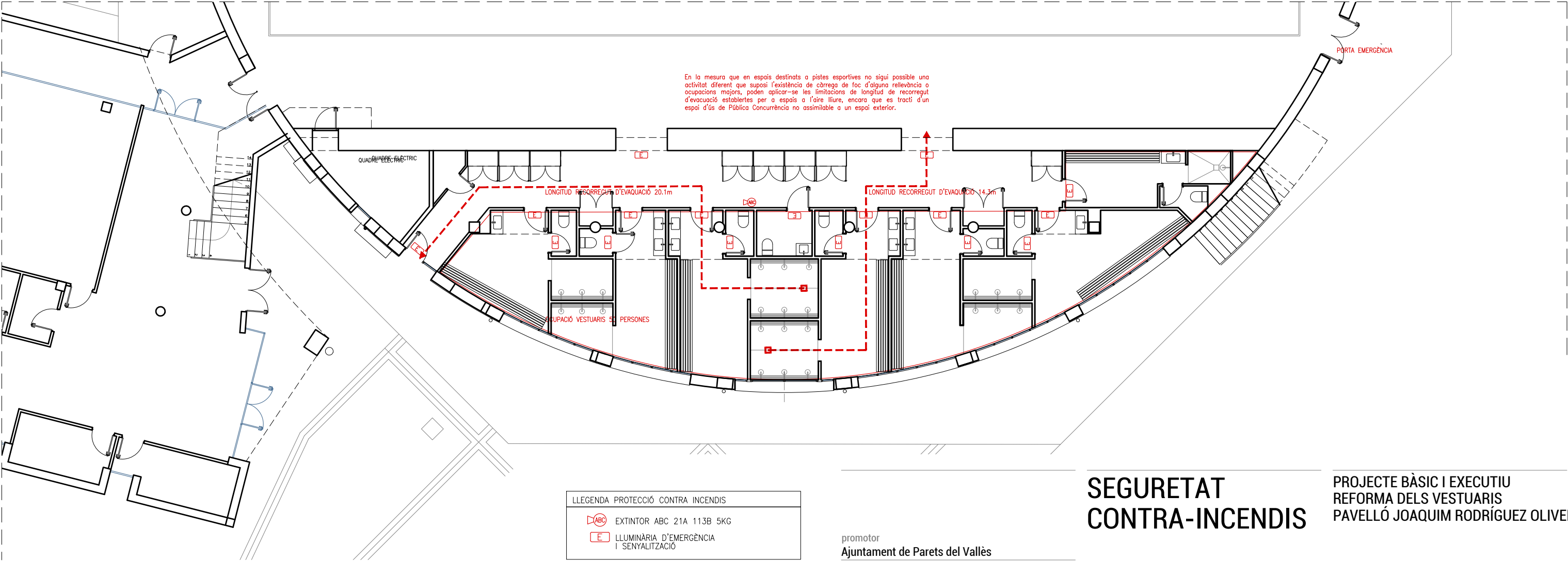
PLANTA BAIXA
