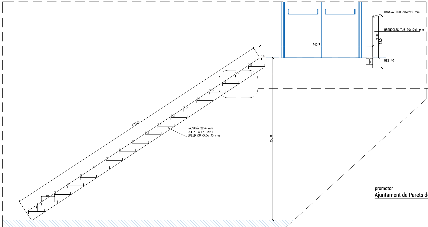
SECCIÓ 1:40
