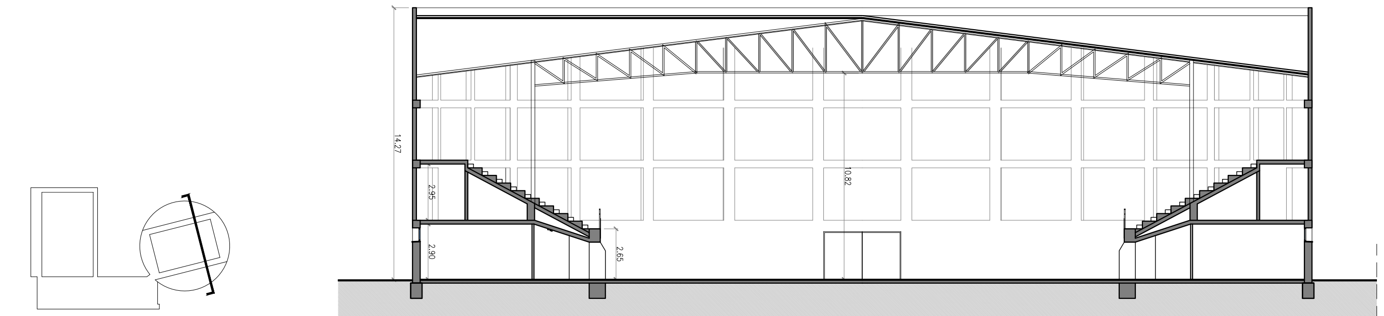
SECCIÓ TRANSVERSAL PER LES GRADES
