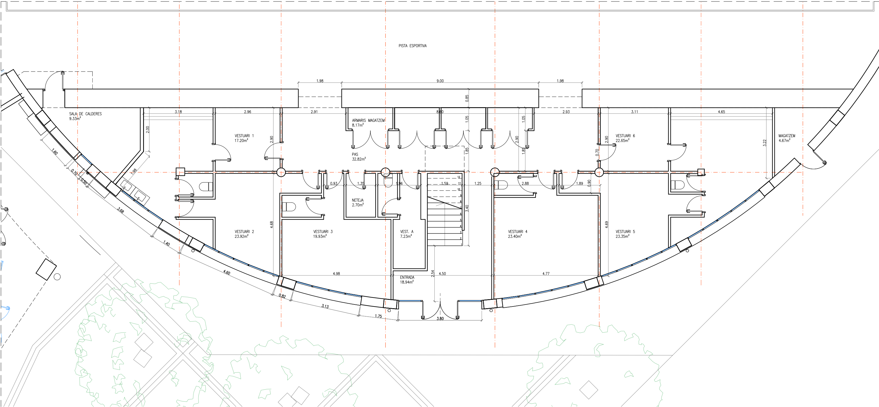
PLANTA BAIXA
