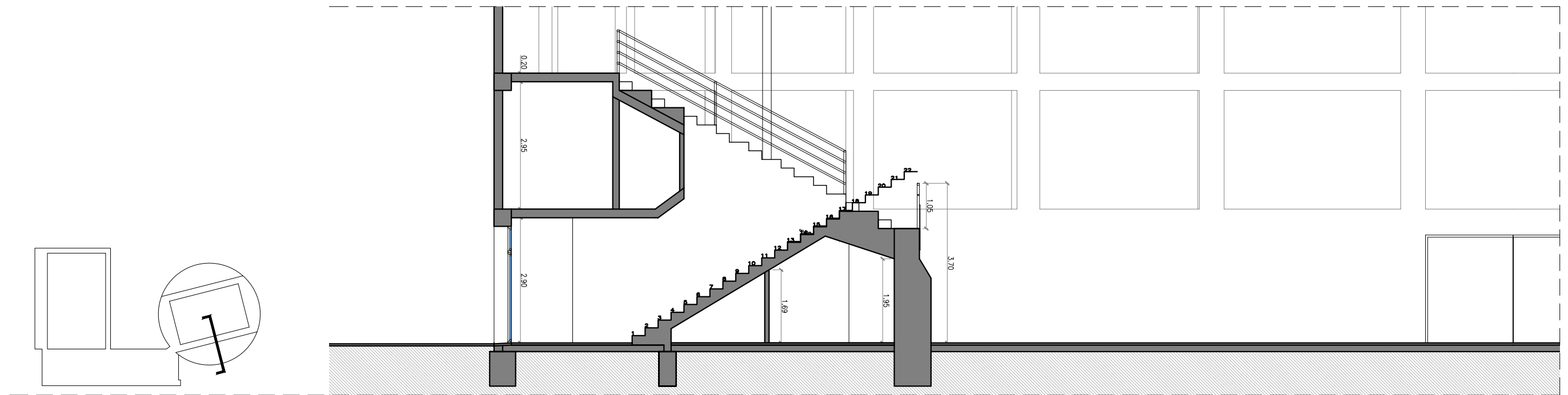
SECCIÓ TRANSVERSAL PER L'ACCÉS
