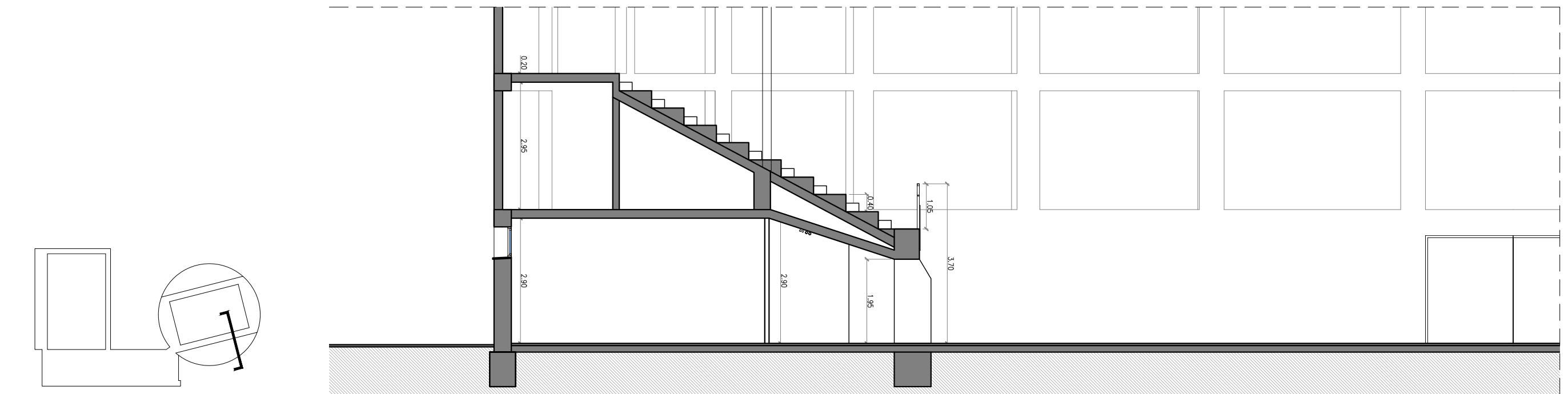
SECCIÓ TRANSVERSAL PER LES GRADES
