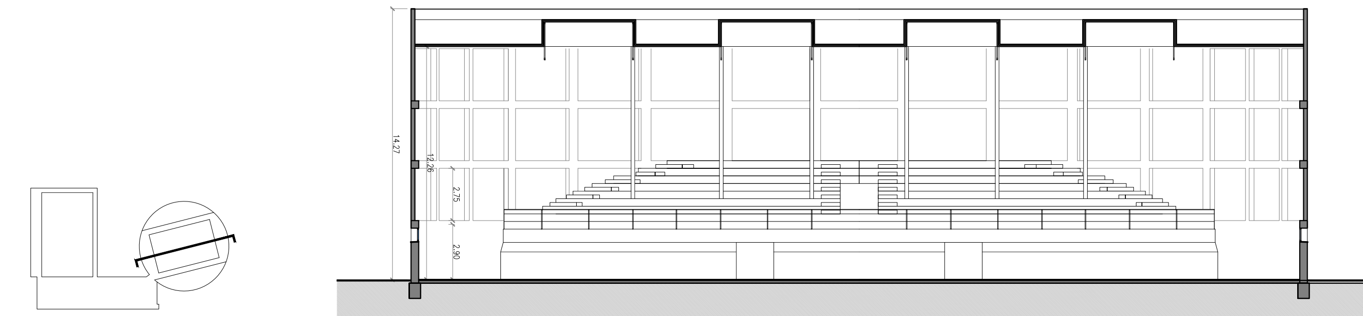
SECCIÓ LONGITUDINAL
