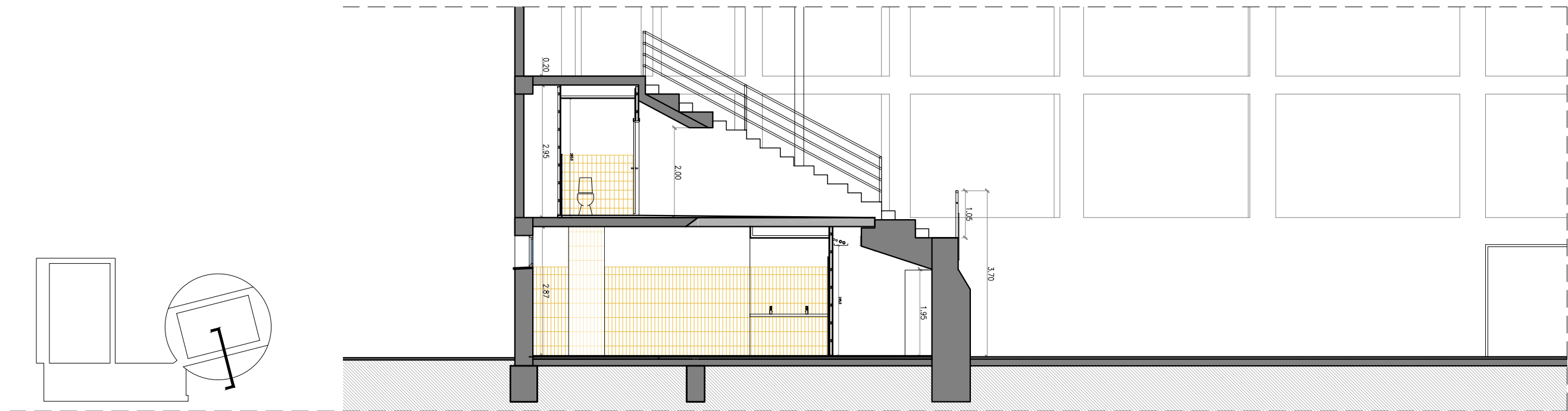
SECCIÓ TRANSVERSAL PER L'ACCÉS
