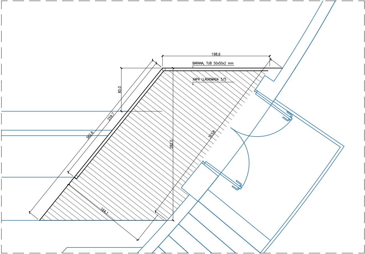
PLANTA 1:40
