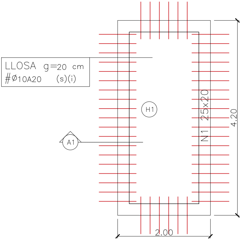
4 SOSTRE PLANTA BAIXA E.: 1/50 DIN A1 E.: 1/100 DIN A3
