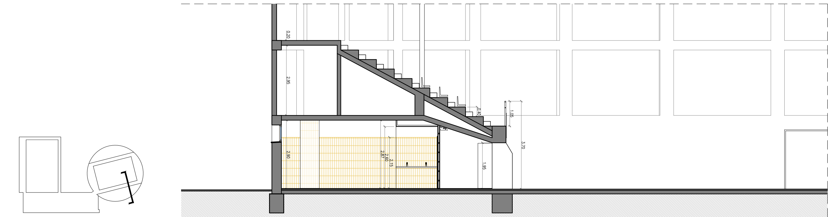
SECCIÓ TRANSVERSAL PER LES GRADES
