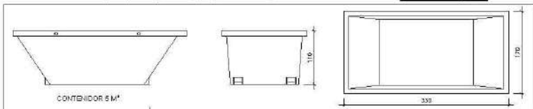
Contenidor 5 m³. Apte per a formigó, ceràmica, petris, fusta i metalls
