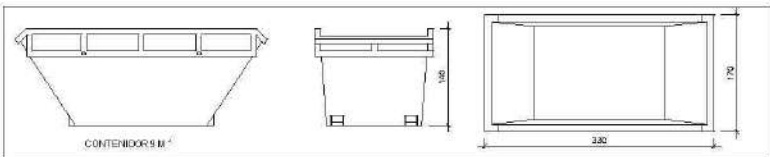
Contenidor 9 m³. Apte per a formigó, ceràmica, petris i fusta
