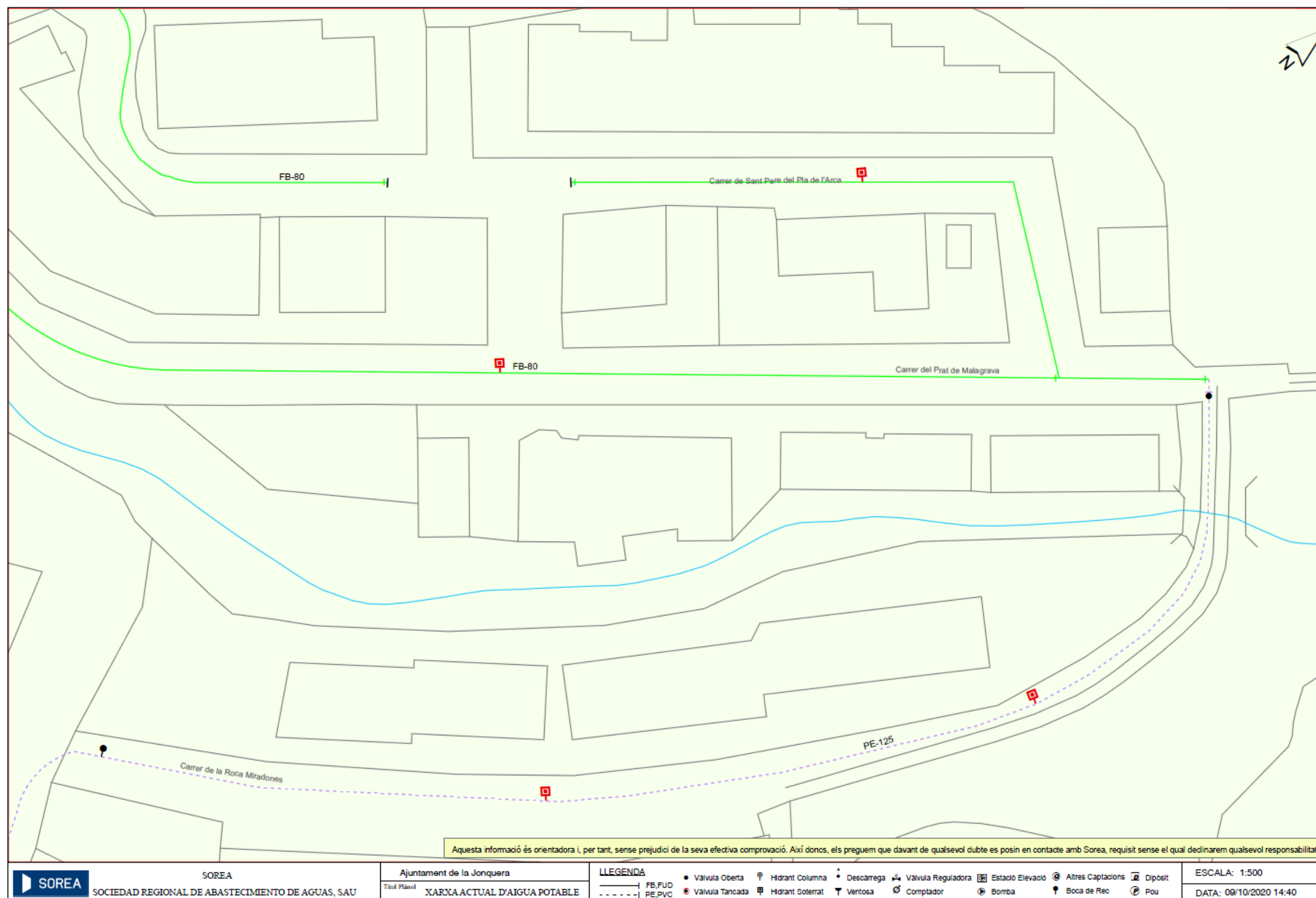
Figura 10. Plànol xarxa d'aigua potable existent. FONT: ACEFAT.
