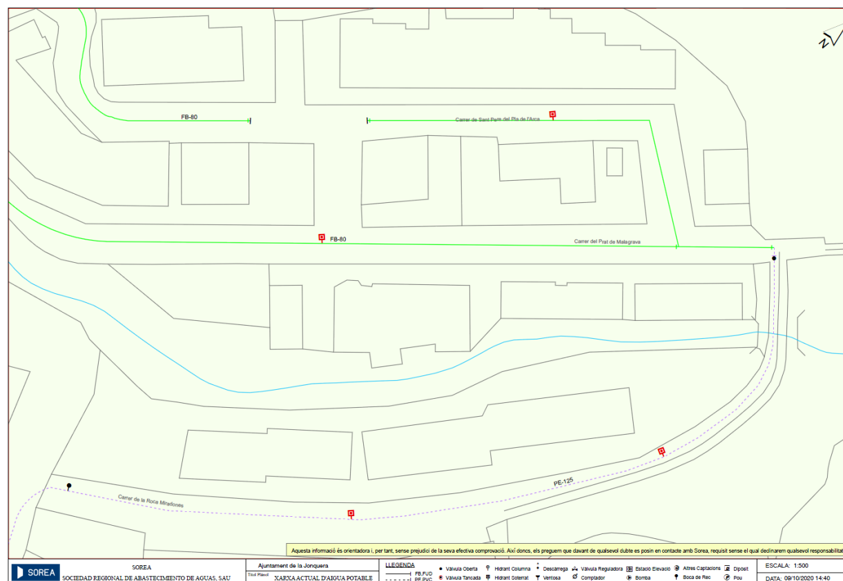
Figura 7. Plànol xarxa d'aigua existent. Font: ACEFAT.
