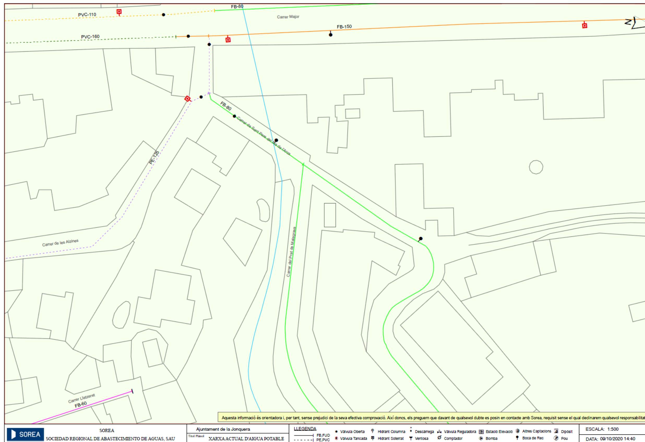
Figura 9. Plànol xarxa d'aigua potable existent. FONT: ACEFAT.
