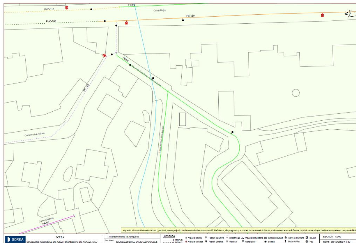
Figura 6. Plànol xarxa d'aigua existent. Font: ACEFAT.
