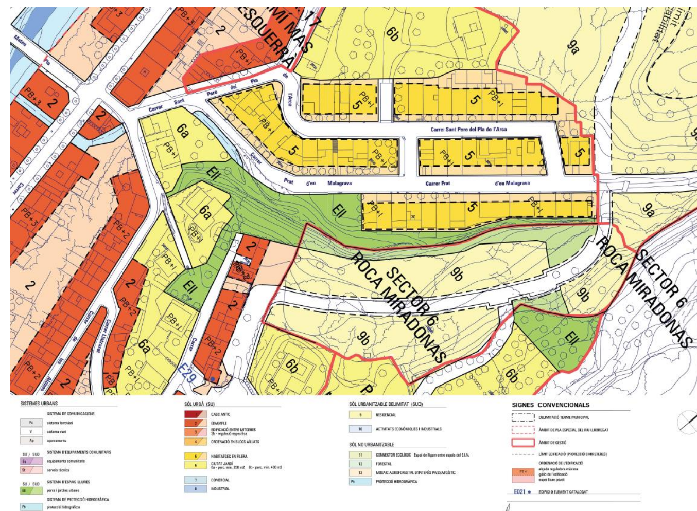
Figura 4. Plànol planejament vigent T.M. La Jonquera. Font: POUM Jonquera.
