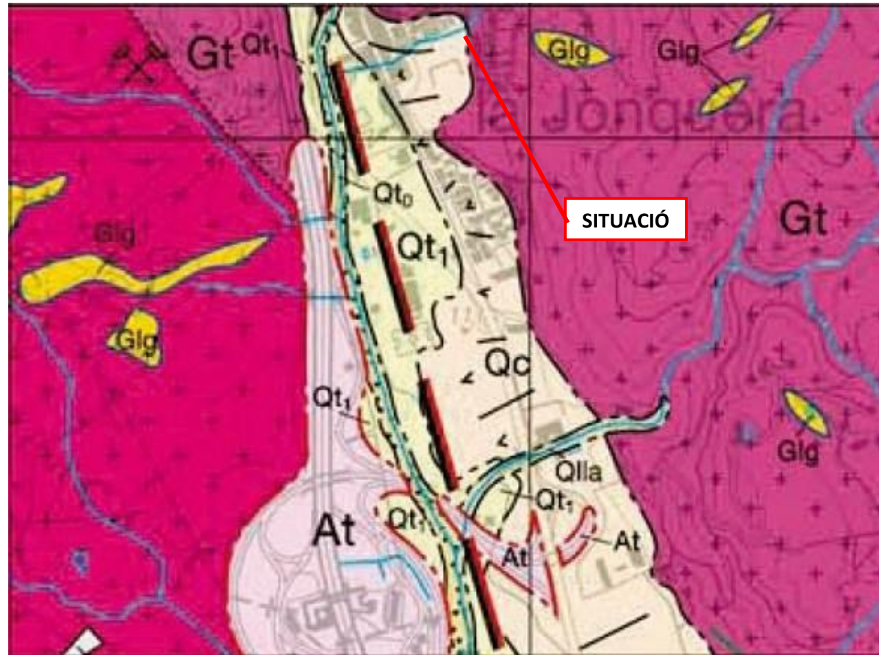
Figura 5. Mapa geològic de Catalunya 1:25.000. Full el Agullana. Font: ICGC
