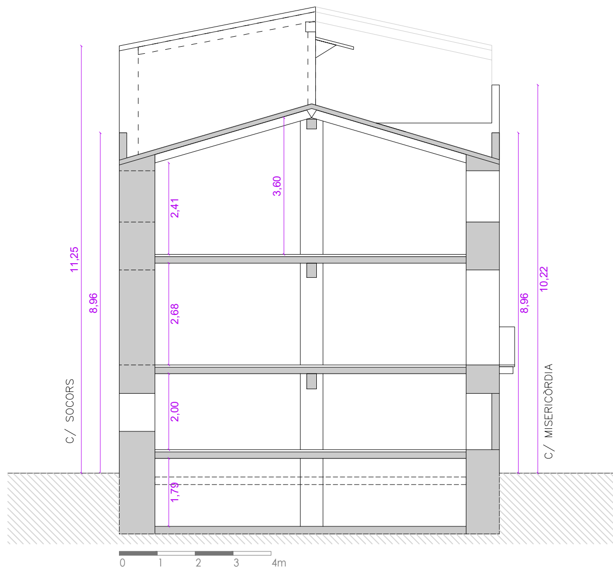
ESTAT ACTUAL SECCIÓ
