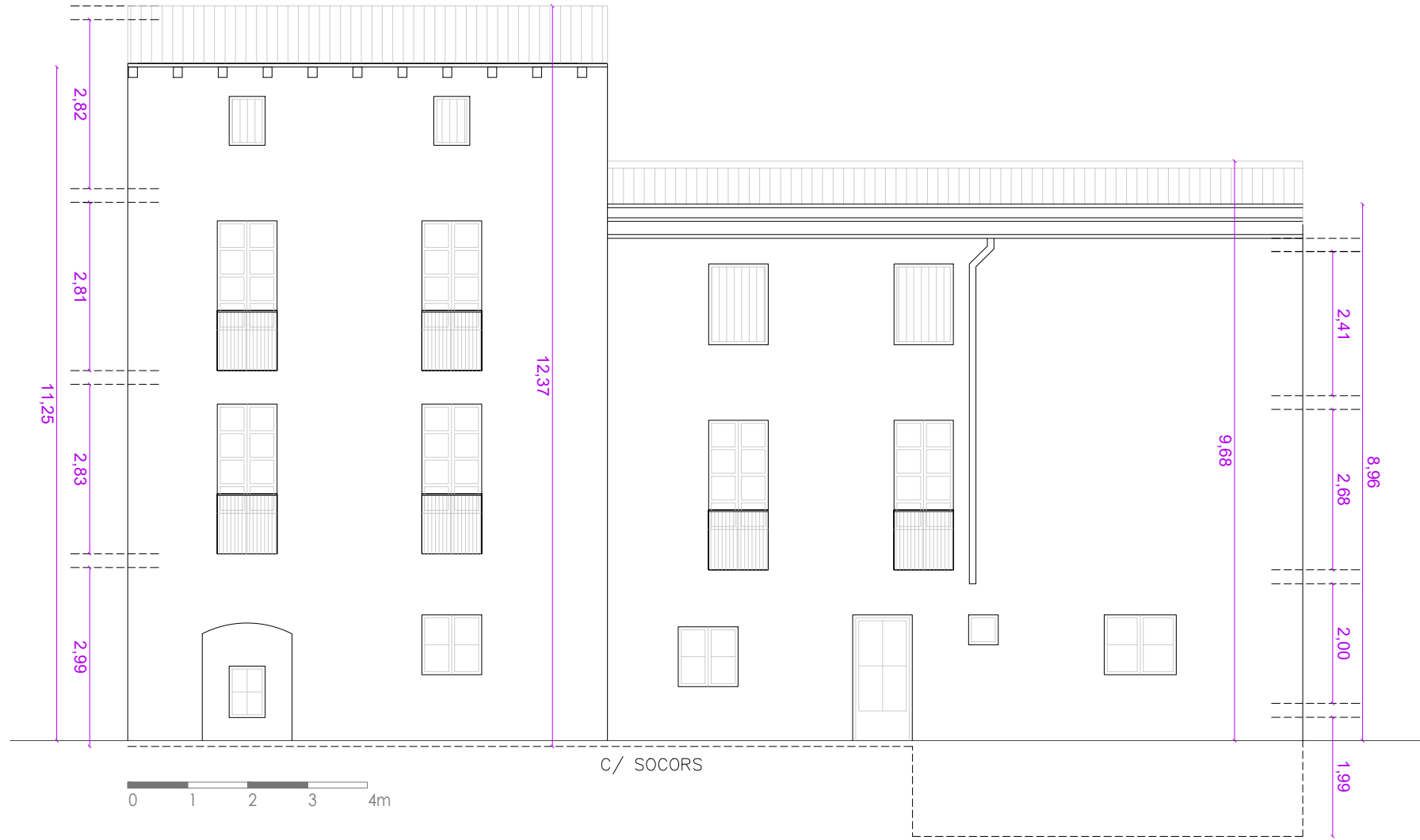
ESTAT ACTUAL FAÇANA CARRER SOCORRS
