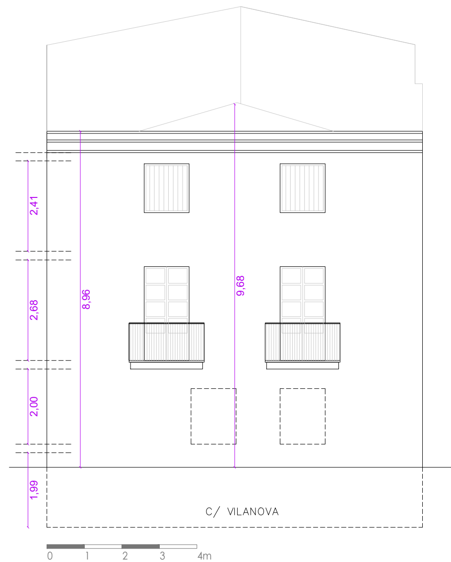
ESTAT ACTUAL ALÇAT CARRER VILANOVA
