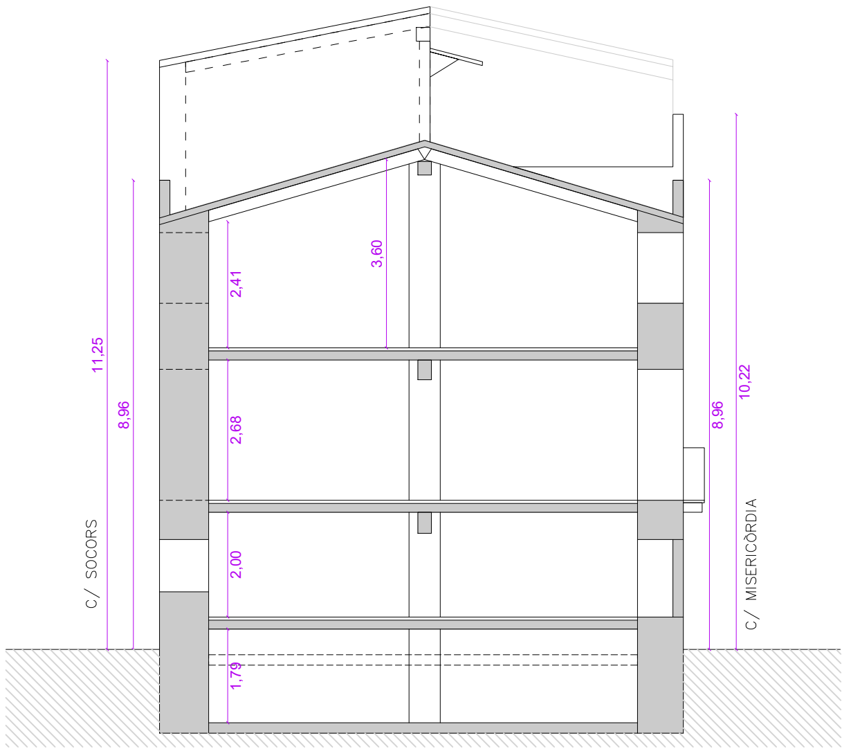
ESTAT PROPOSTA FAÇANA CARRER SOCORRS SECCIÓ
