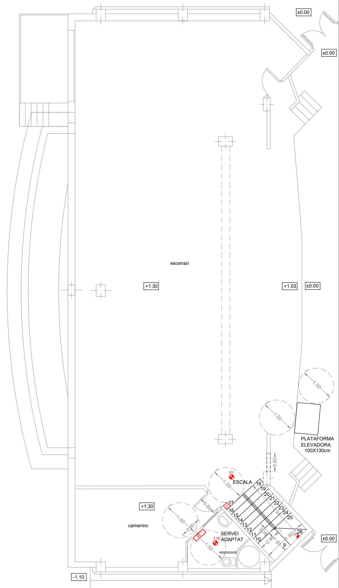
PLANTA BAIXA
