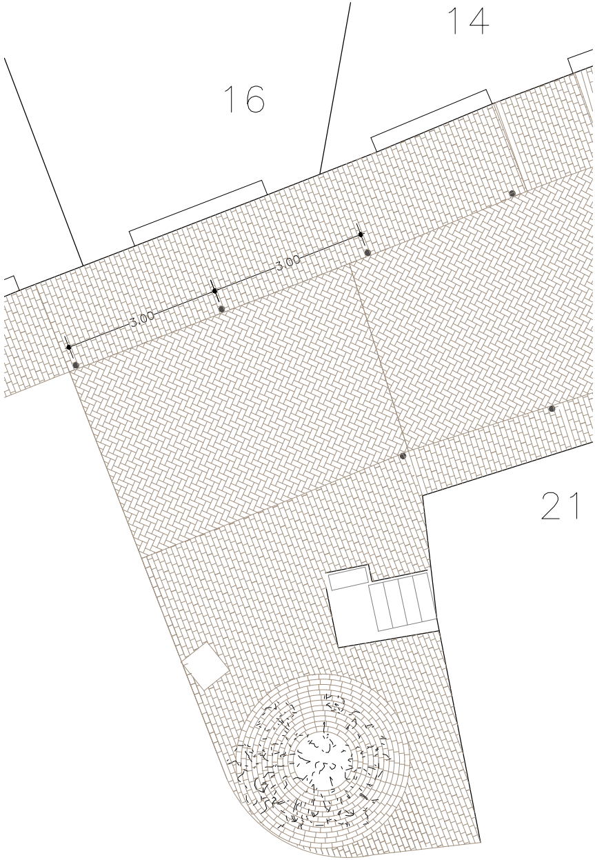
DETALL COL.LOCACIÓ PAVIMENT ESC.1/100
