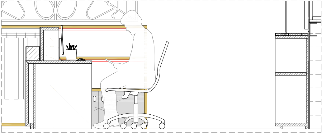
Sección longitudinal FF' e 1/25
