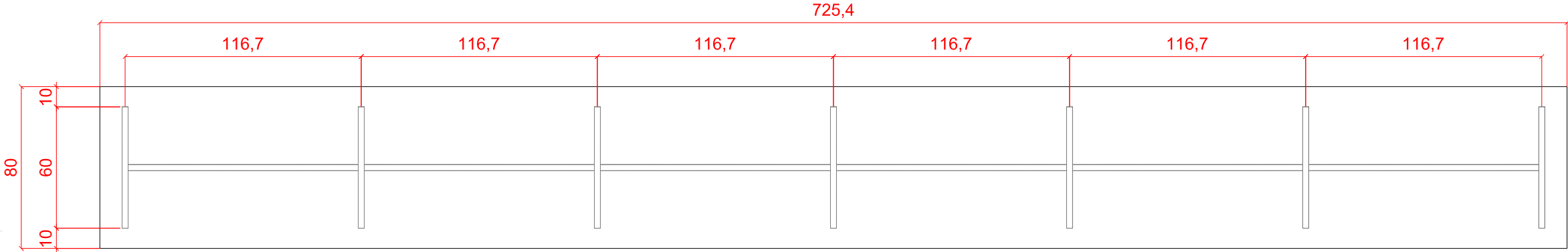
Planta estructura de madera e 1/25
