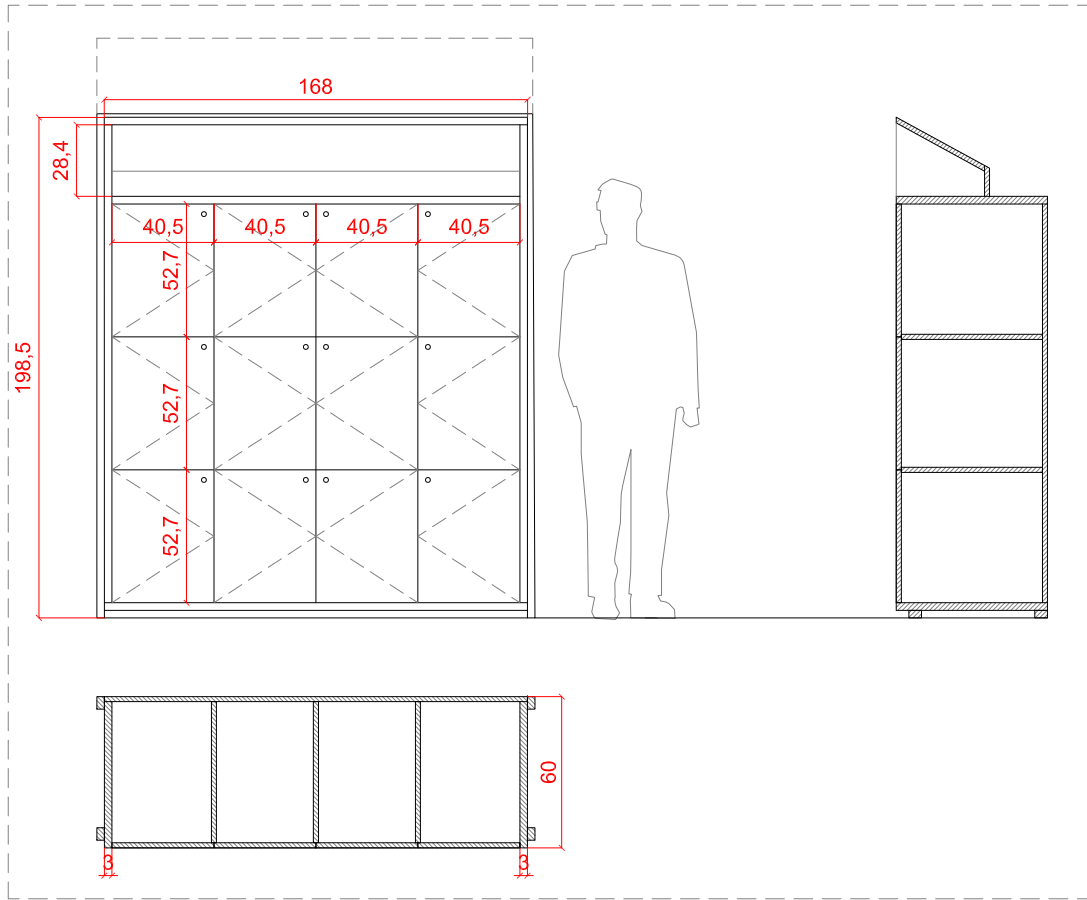
Detalle armario e 1/30
