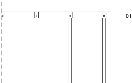
Detalle expositor y arranque de los tirantes
