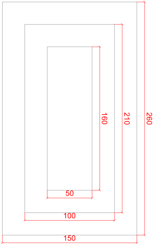
Planta e 1/25
