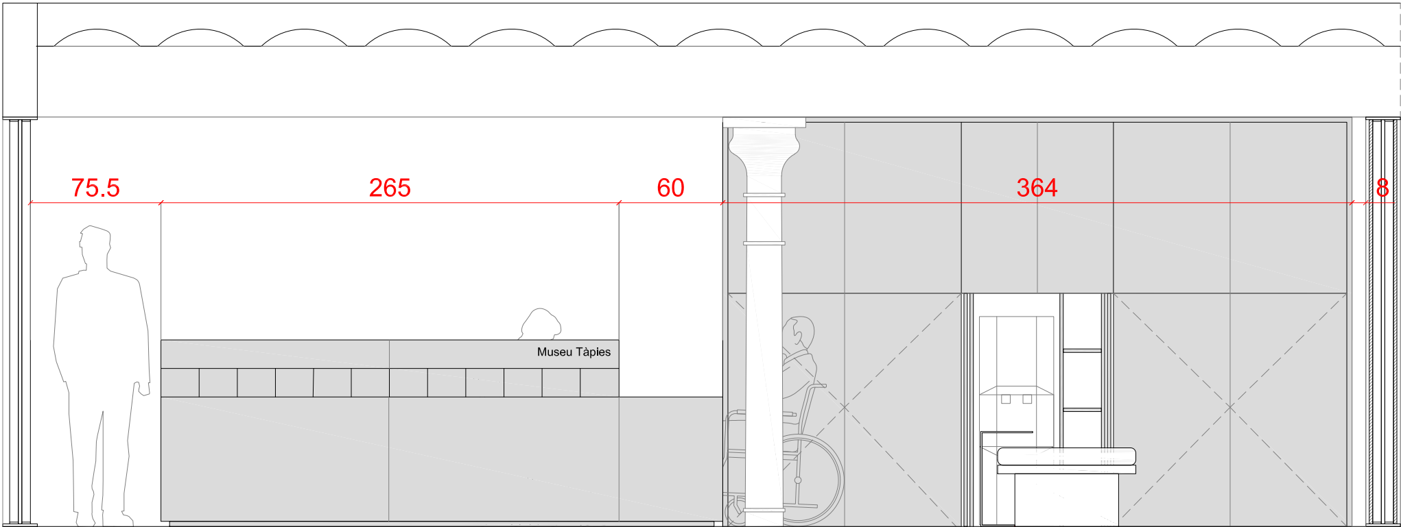
Sección-alzado transversal DD' e 1/30
