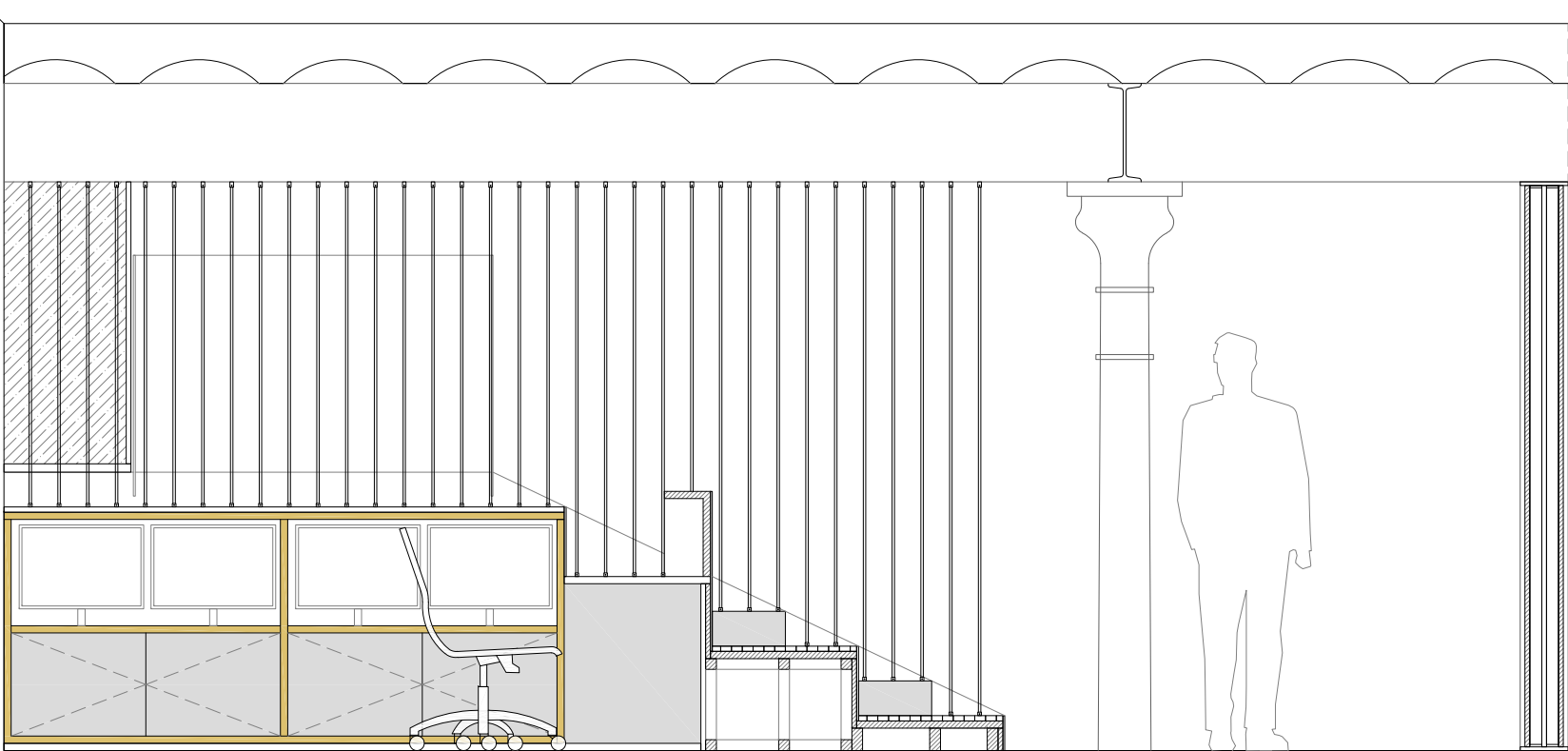
Sección-alzado transversal CC' e 1/30
