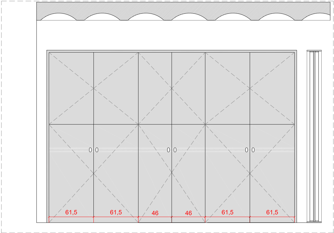
Alzado longitudinal e 1/30
