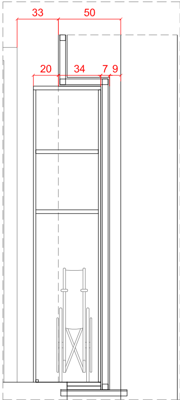
Sección transversal e 1/30
