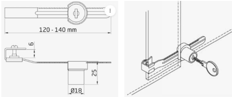
Cerradura para vitrina
