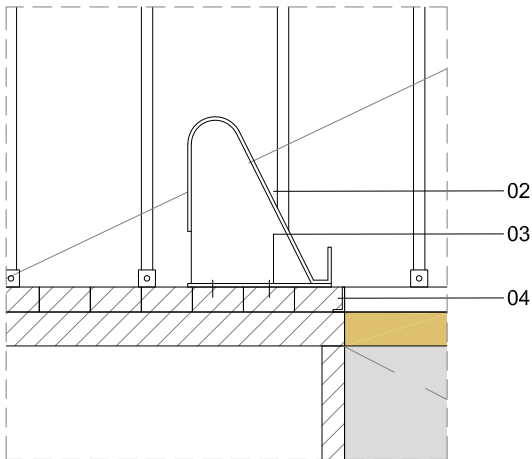
Detalle expositor y arranque de los tirantes
