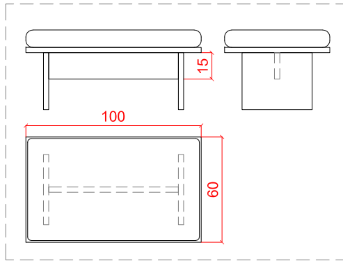
Detalle banco e 1/30
