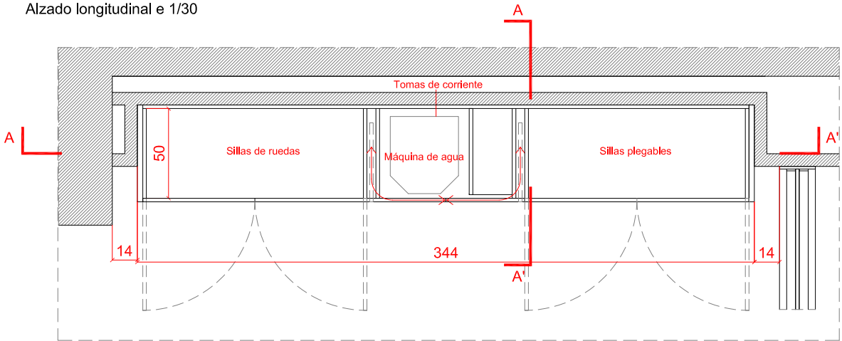
Planta e 1/30
