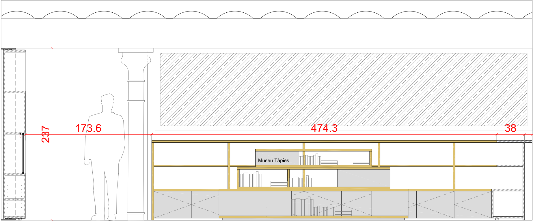
Sección-alzado transversal AA' e 1/30
