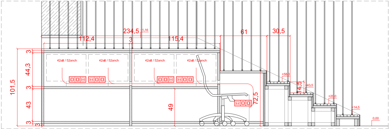
Sección transversal EE' e 1/25
