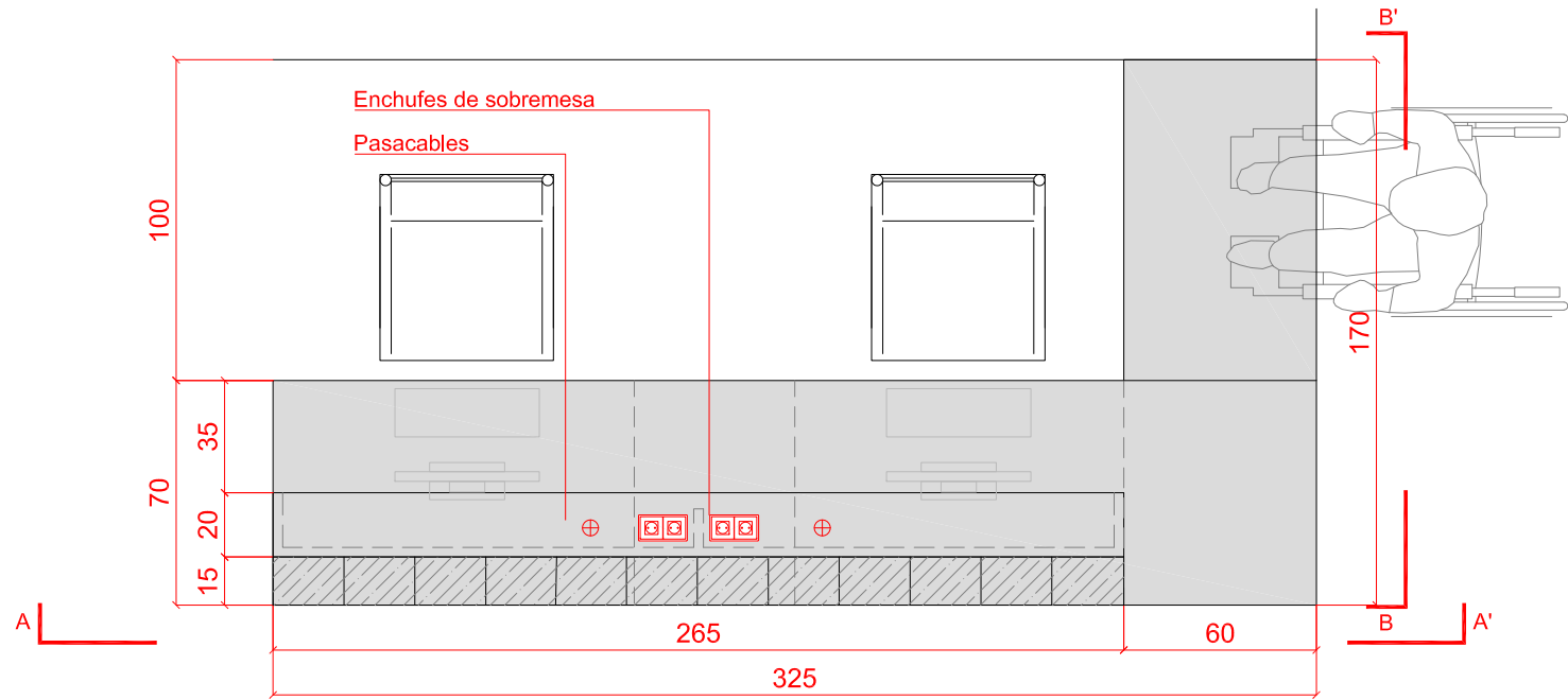
Planta e 1/25
