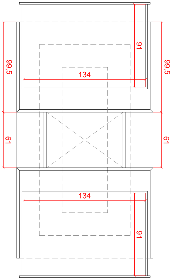
Sección EE' e 1/25
