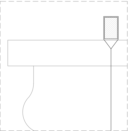
Detalle listón superior de tramo central de cortina
