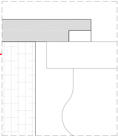
Detalle de apoyo sobre U metálica
