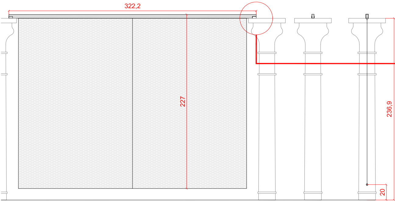
Alzado longitudinal BB' e 1/30
