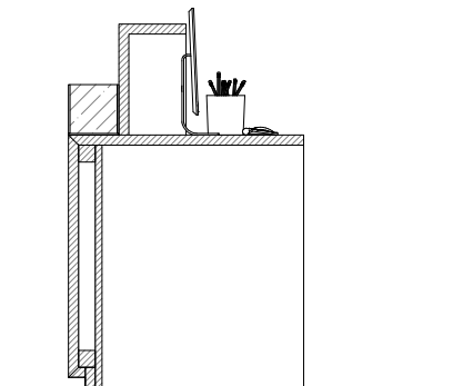
Sección transversal EE' e 1/25
