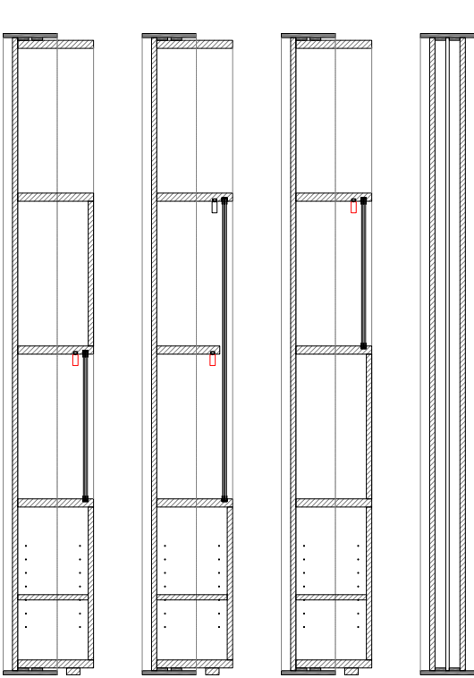
Vitrina (3uds) Secciones transversales A,B,C,D 1/25
