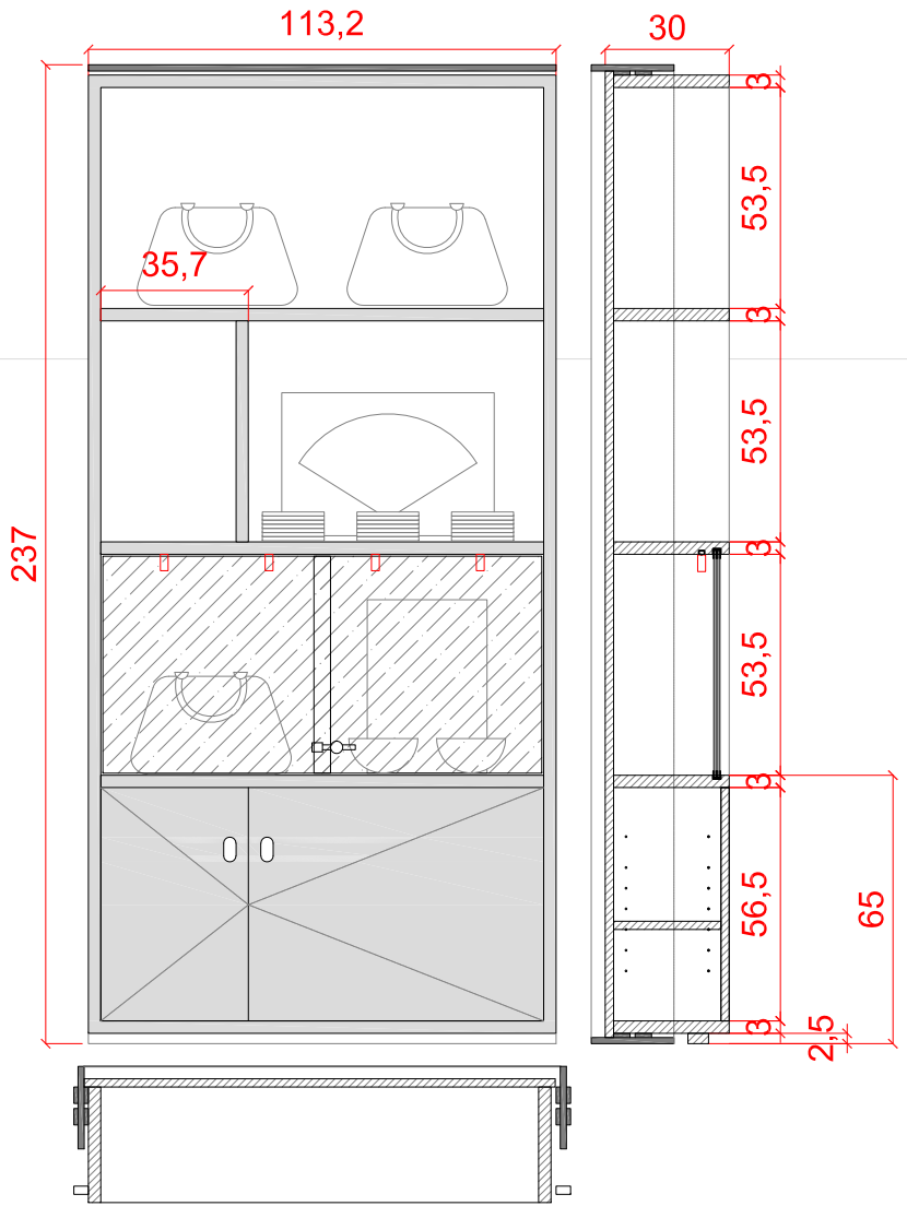
Detalles mueble A-A' e 1/20
