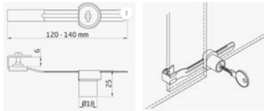
Cerradura para vitrina
