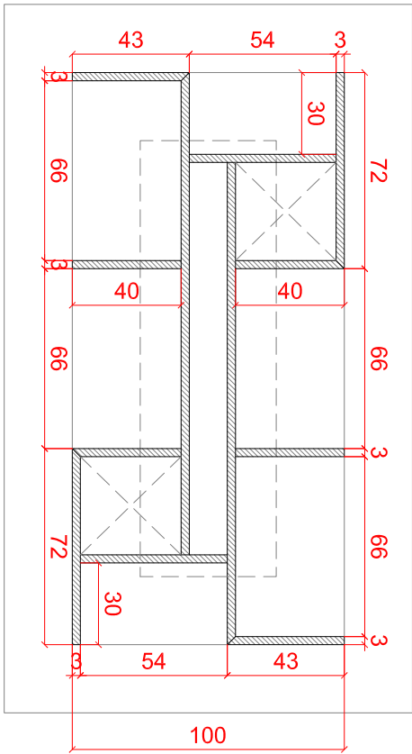
Sección FF' e 1/25
