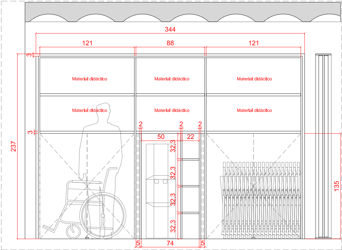
Sección longitudinal AA' e 1/30
