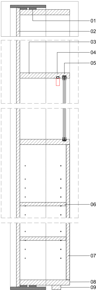
Detalle Secc. transversal DD' e 1/10
