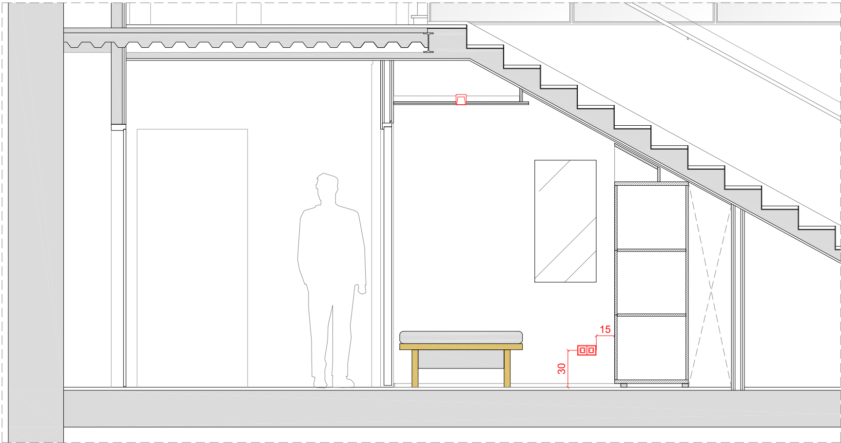
Sección longitudinal AA' e 1/30
