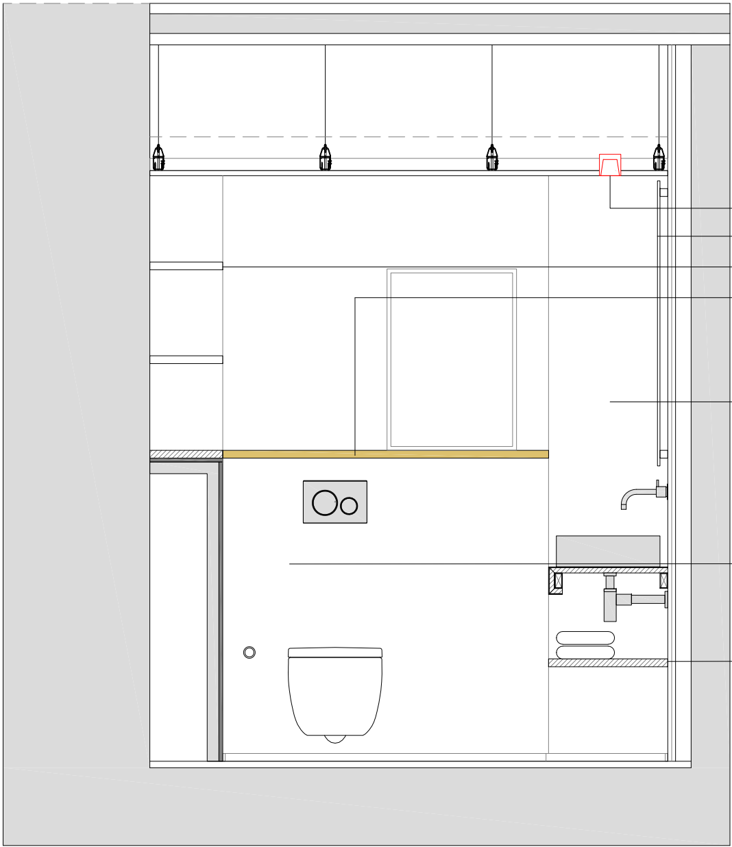
Sección BB. Detalle e 1/20
