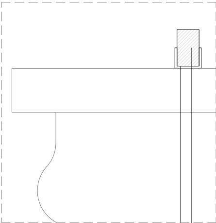
Detalle de apoyo sobre U metálica
