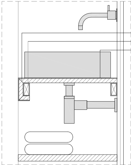
Sección BB. Detalle e 1/10
