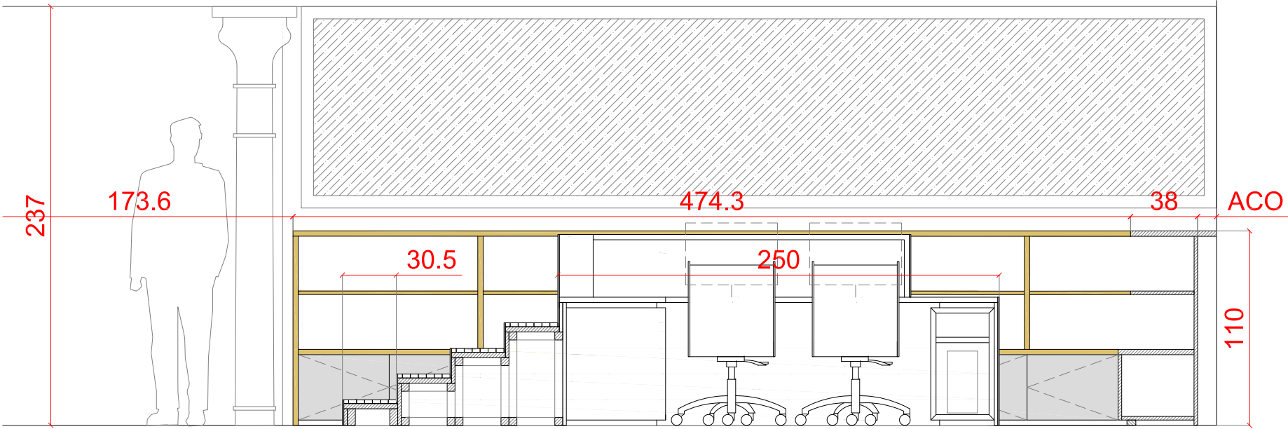
Sección-alzado transversal BB' e 1/30
