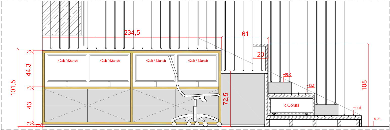
Sección transversal DD' e 1/25
