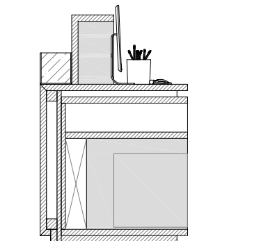
Sección transversal DD' e 1/25
