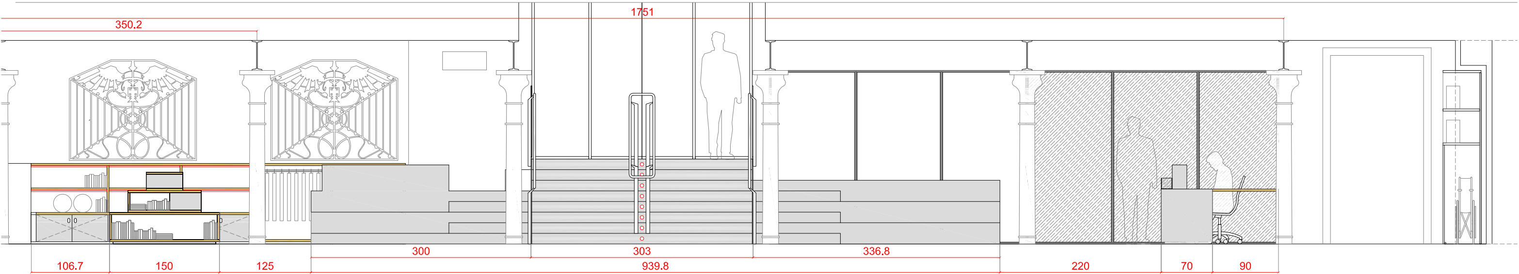
Alzado longitudinal BB' e 1/50
