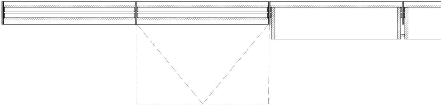
Sección longitudinal FF' e 1/20
