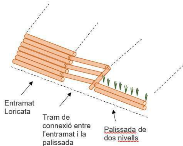
Figura 13 Esquema del tram de transició entre l'entramat i la palissada de dos nivells
