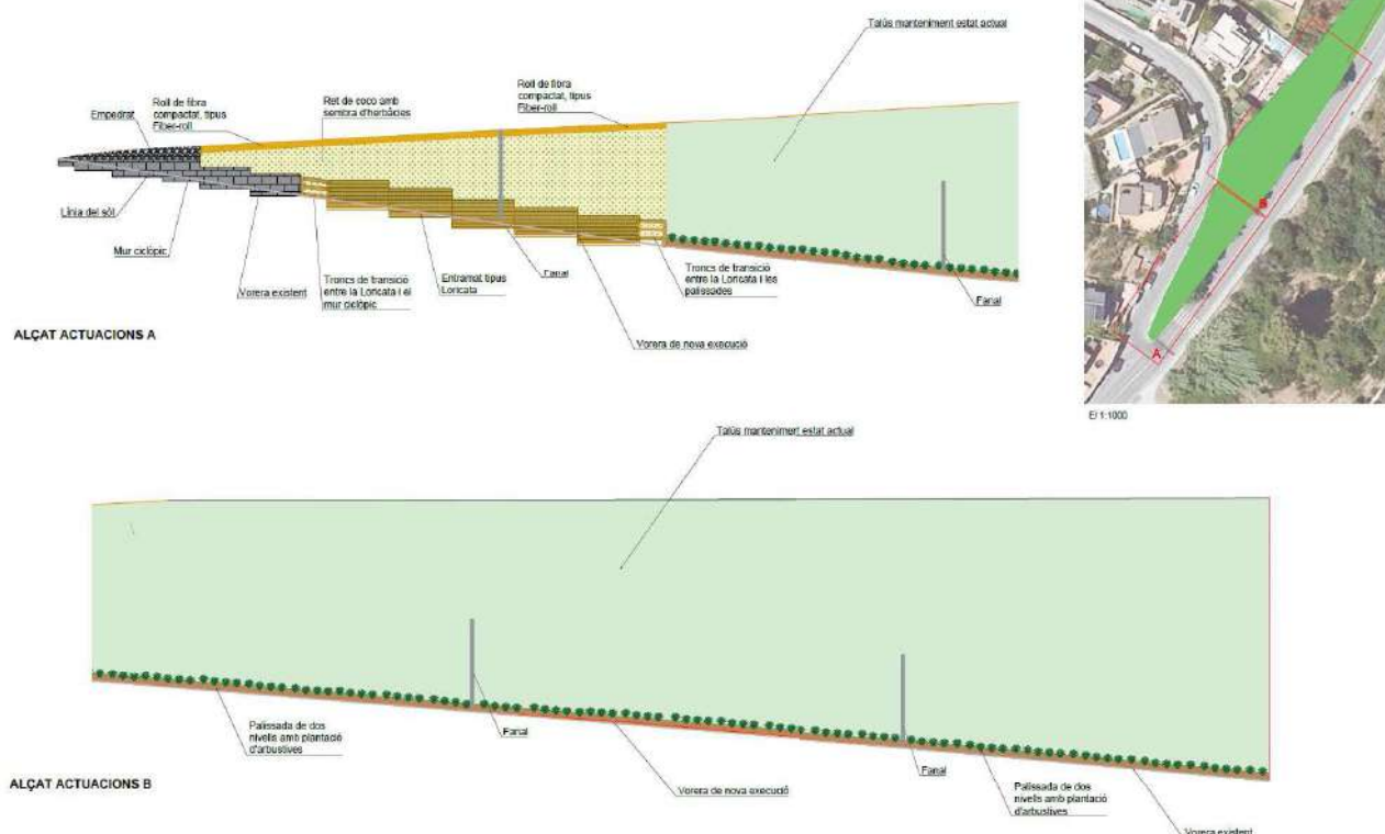
Figura 11 Alçat general de la proposta d'actuació
