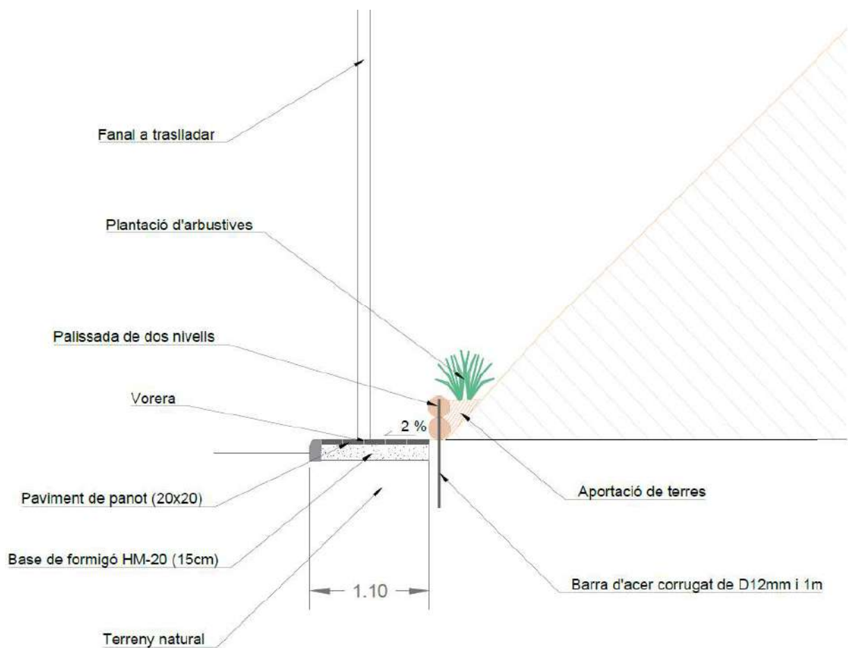
Figura 21 Secció tram amb nova vorera
