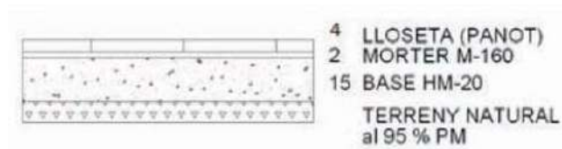
Figura 20 Esquema de la secció tipus de la vorera
