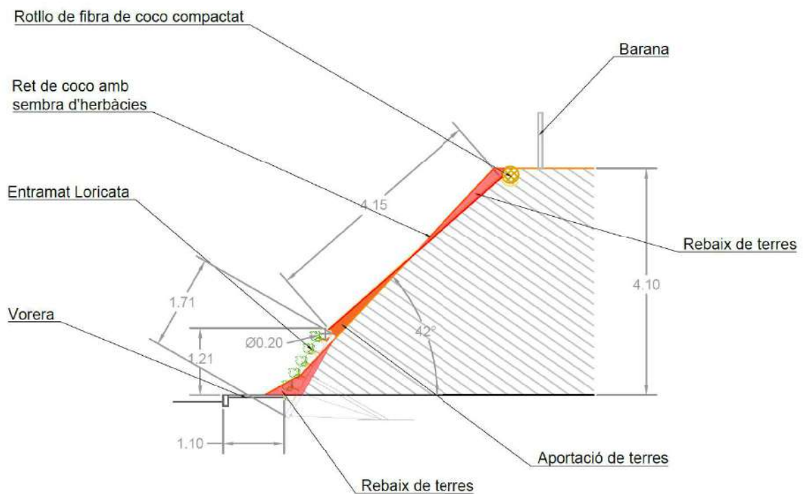
Figura 16 Secció de tram amb entramat Loricata
