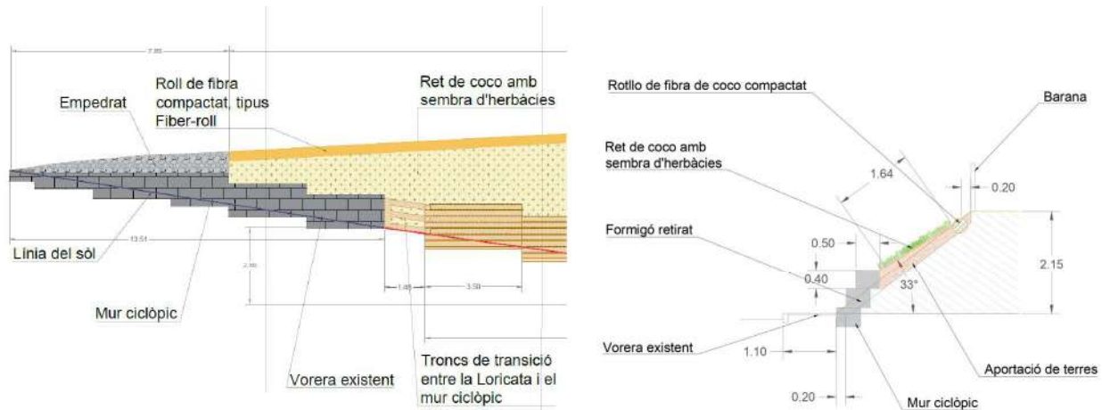
Figura 18 Alçat i secció del mur ciclòpic
