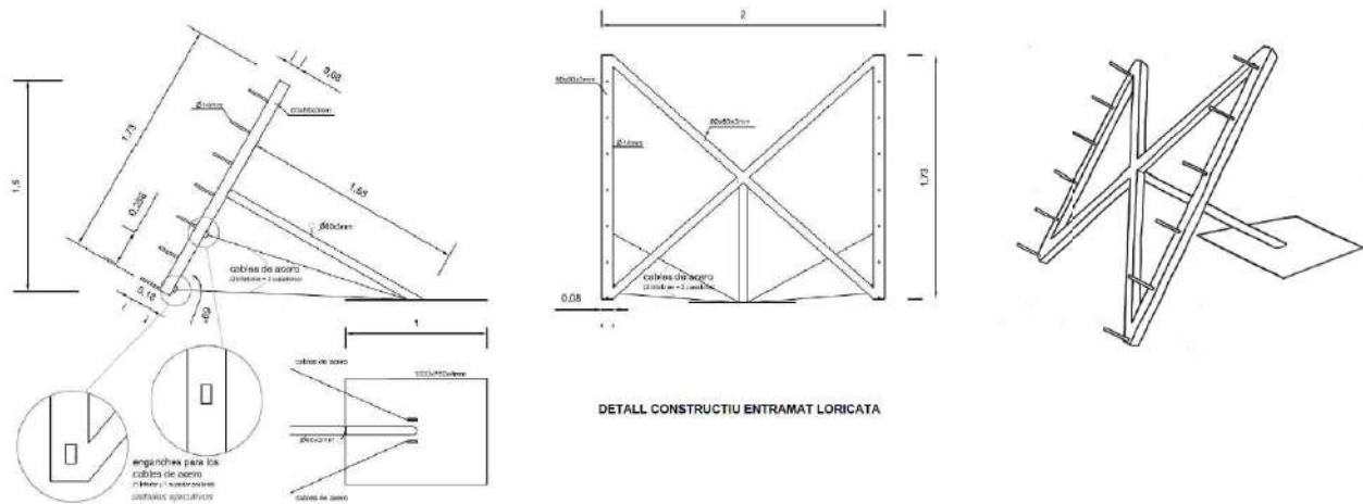
Figura 17 Loricata de 7 nivells utilitzada en el projecte
