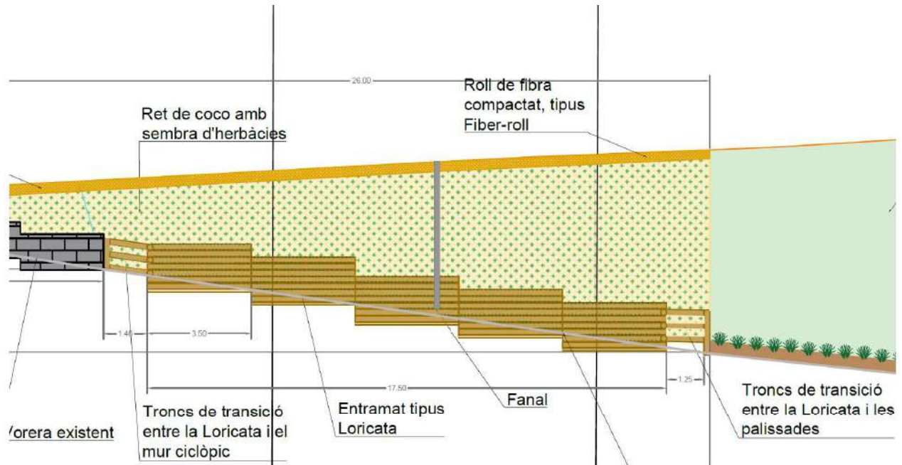
Figura 15 Alçat amb el tram d'entramat Loricata
