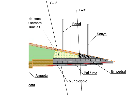
ALÇAT - E 1:150
