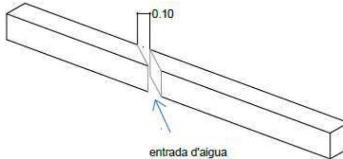
Figura 10 Detall tall de vorada
