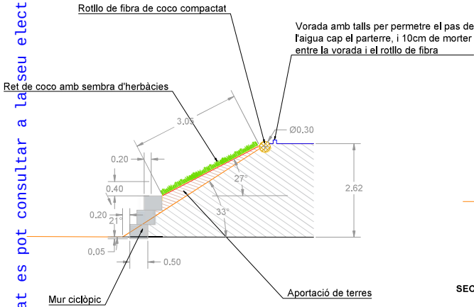
SECCIÓ C-C' - E 1:75
