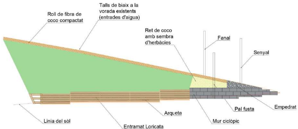
Figura 8 Alçat general de la proposta d'actuació
