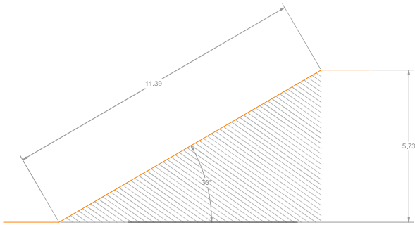
SECCIÓ B-B' - E 1:100
