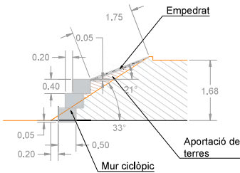
SECCIÓ B-B' - E 1:75
