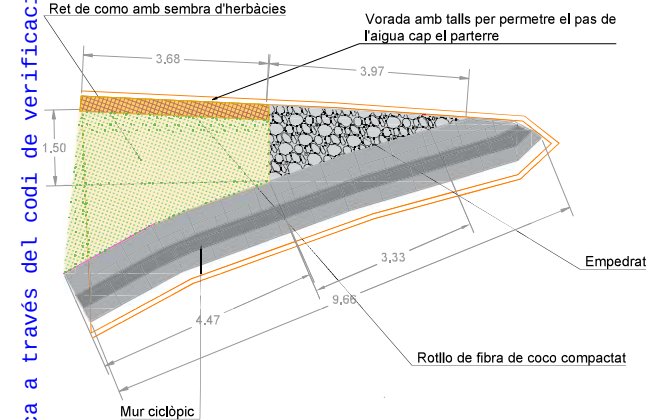
Planta - E 1:75
