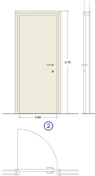
Porta 80 Magatzem-neteja i arxiu (2uts)
