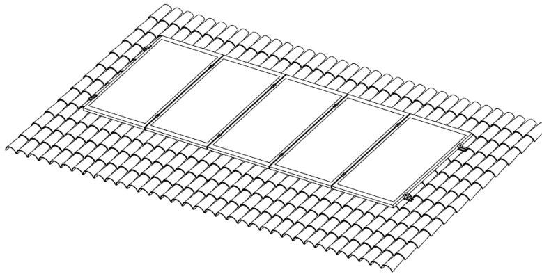
Fig. 6.2. Sistema de subjecció coplanar Aplisun.
