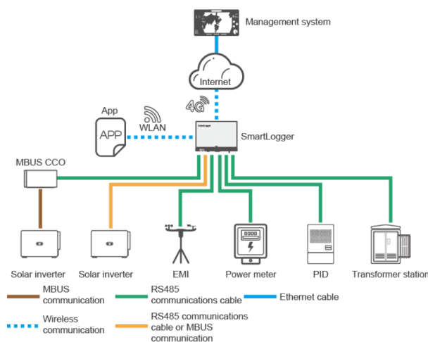
Fig. 6.2. Connexionat i funcionament del sistema de monitoratge.
