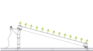
Carga local de succión del viento [kN/m 2 ] en el módulo
