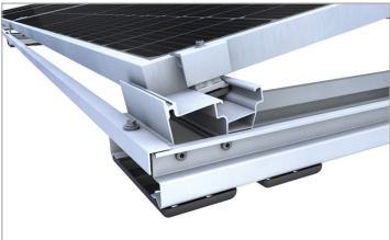
Esquina del módulo con pinza final, pie de apoyo y tira de soporte
