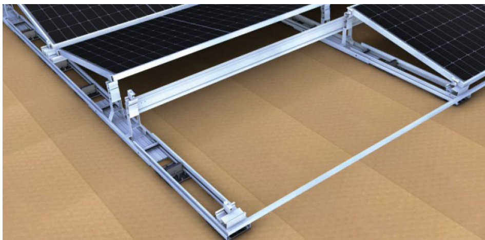
Fig. 6.3. Sistema de subjecció autoportant Novotegra.
