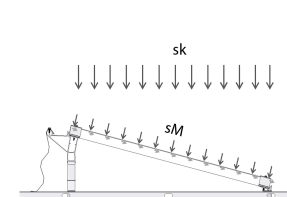
sk: Carga de nieve en suelo sM: Carga de nieve perpendicular en el módulo [kN/m 2 ] = [kPa]
