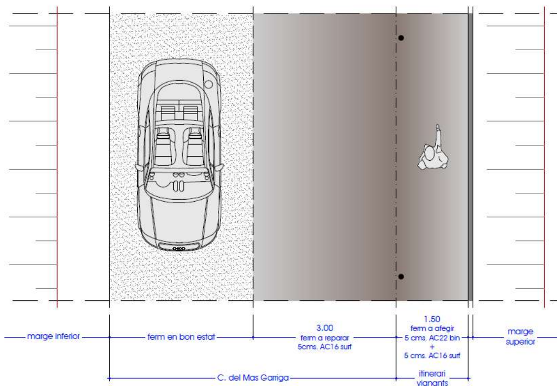
Planta i secció tipus del tram de C. Mas Garriga amb especial detall de l'itinerari per a vianants que discorre paral·lel pel costat dret del carrer.
