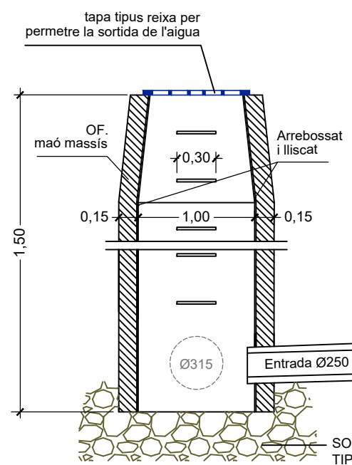
SECCIÓ Pou de graves de secció circular Ø100
