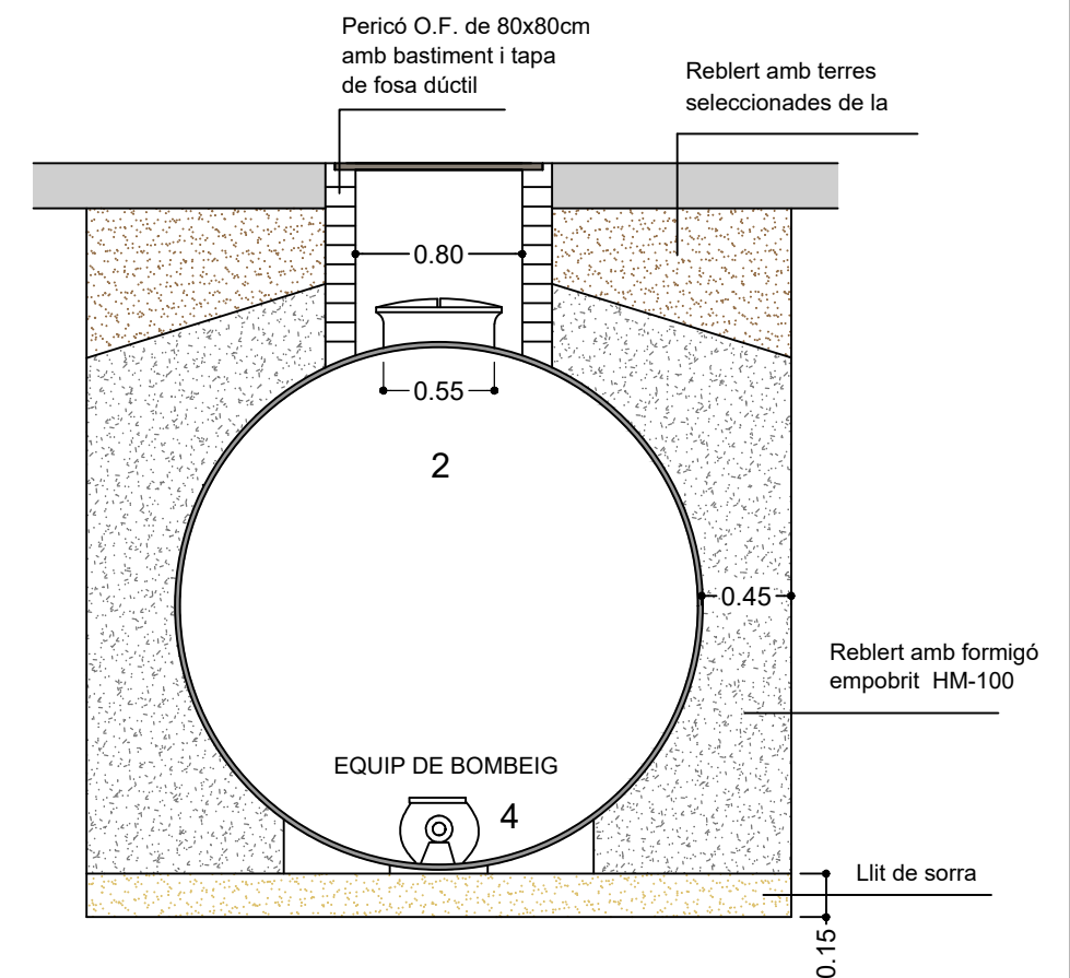
SECCIÓ TRANSVERSAL
