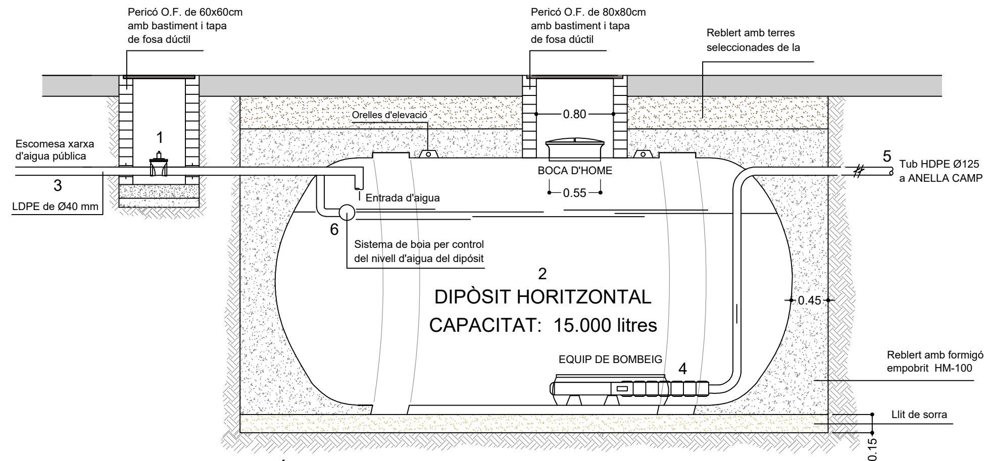
SECCIÓ LONGITUDINAL
