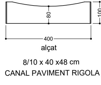
secció A secció B alçat 8/10 x 40 x 48 cm CANAL PAVIMENT RIGOLA
