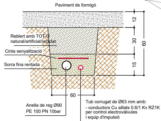
DETALL RASA
